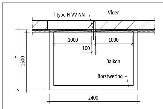
Afb. 212: Schöck Isokorb® T type K-E, K-T met type H: Statisch systeem, en bovenaanzicht
