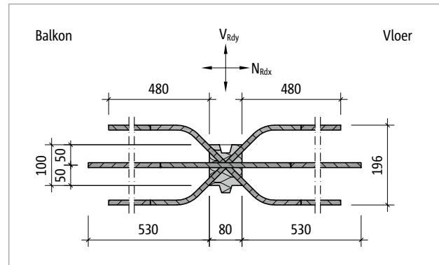
Afb. 211: Schöck Isokorb® T type H-VV2-NN1: Bovenaanzicht
