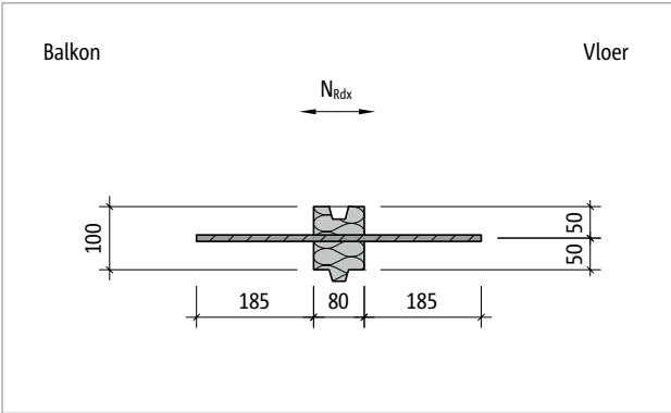
Afb. 205: Schöck Isokorb® T type H-NN1: Bovenaanzicht
