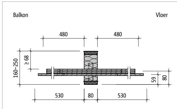
Afb. 210: Schöck Isokorb® T type H-VV2-NN1: Zijaanzicht
