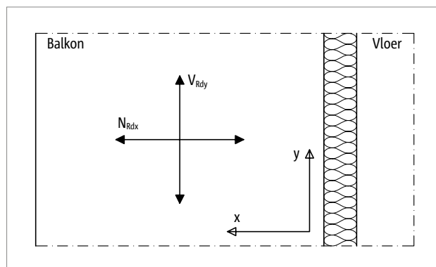
Afb. 202: Schöck Isokorb® T type H: Tekening voor de maatgeving
