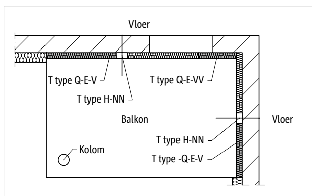
Afb. 198: Schöck Isokorb® T type H: Balkon aan twee kanten ondersteund
