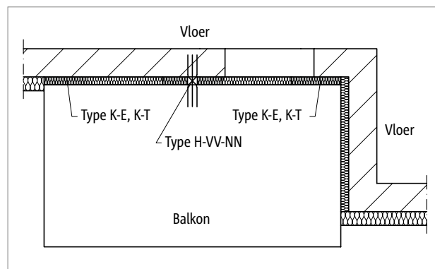
Afb. 197: Schöck Isokorb® T type H: Vrij uitkragend balkon
