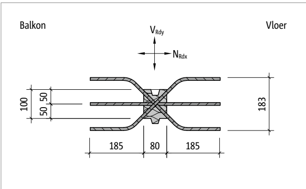
Afb. 209: Schöck Isokorb® T type H-VV1-NN1: Bovenaanzicht
