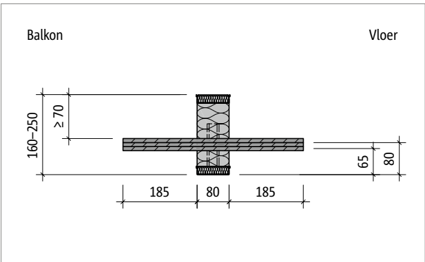
Afb. 208: Schöck Isokorb® T type H-VV1-NN1: Zijaanzicht
