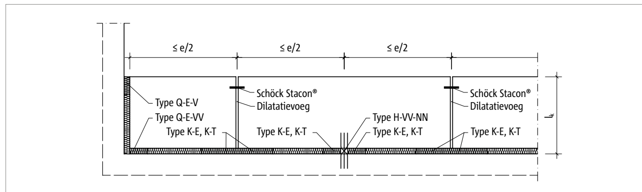
Afb. 203: Schöck Isokorb® T type H: Opstelling uitzetvoegen
