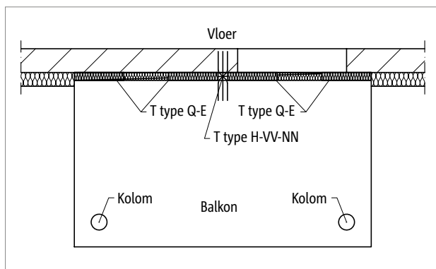
Afb. 196: Schöck Isokorb® T type H: Ondersteund balkon
