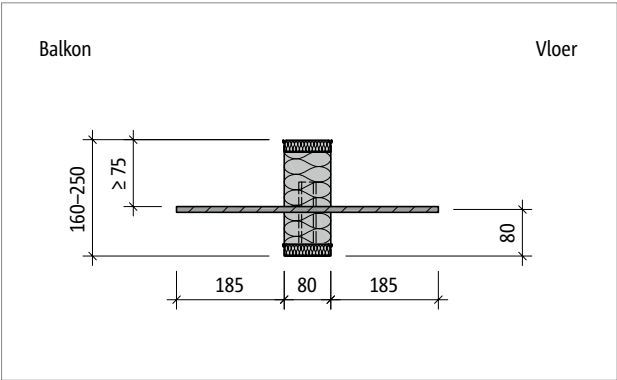
Afb. 204: Schöck Isokorb® T type H-NN1: Zijaanzicht
