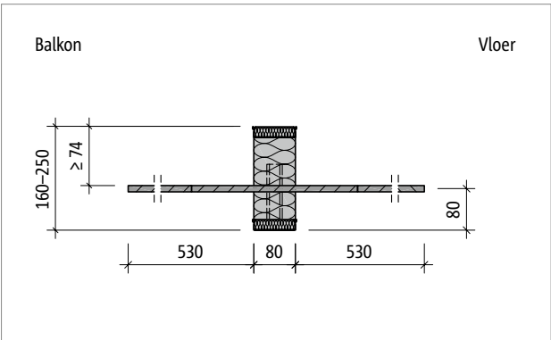
Afb. 206: Schöck Isokorb® T type H-NN2: Zijaanzicht
