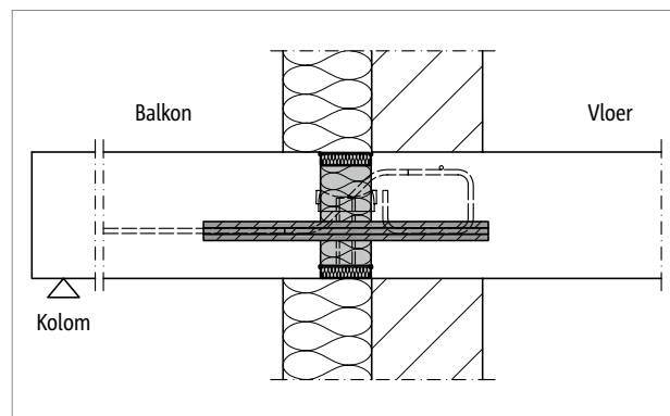
Afb. 200: Schöck Isokorb® T type H-VV-NN: Met T type Q-E; aansluiting bij buitenisolatie
