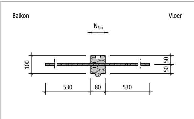
Afb. 207: Schöck Isokorb® T type H-NN2: Bovenaanzicht
