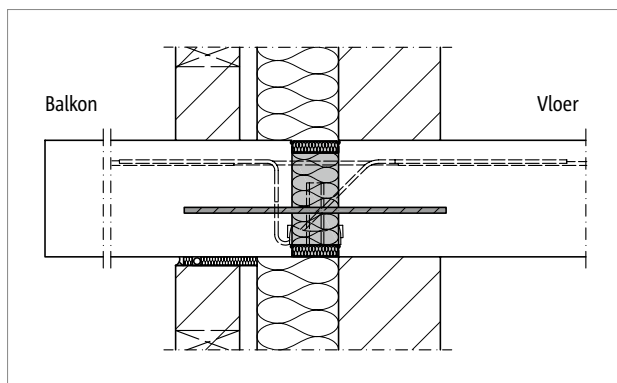
Afb. 199: Schöck Isokorb® T type H-NN: Met T type K-E, K-T; aansluiting bij spouwmuur
