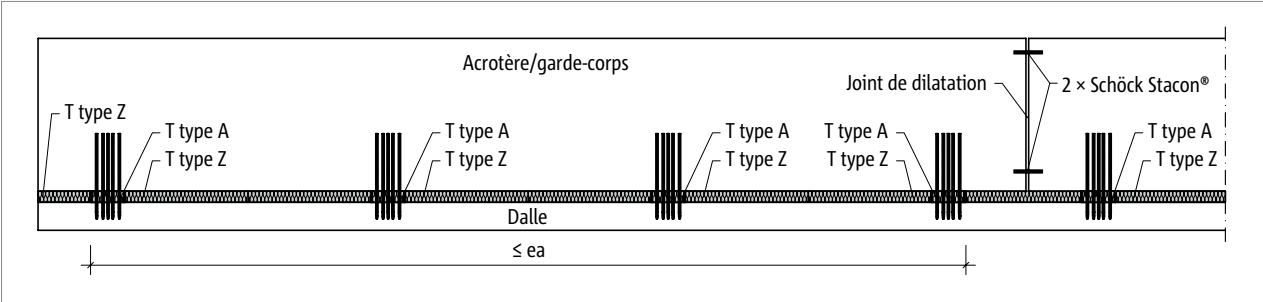
Fig. 233: Schöck Isokorb® T type A : disposition des joints de dilatation
