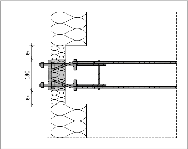
Fig. 108: Schöck Isokorb® T tipo SQP: distanze tra i bordi
