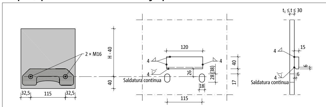
Fig. 111: Schöck Isokorb® T tipo SQP: costruzione del raccordo della piastra di testa
