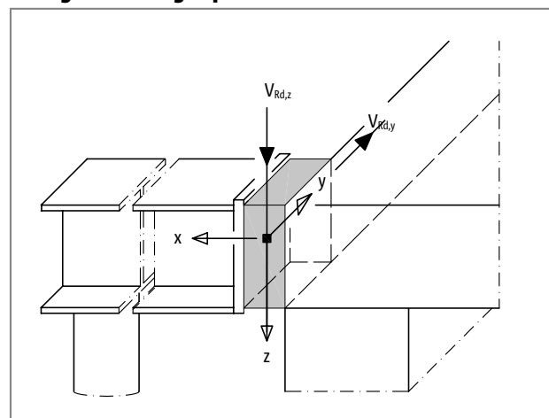
Fig. 104: Schöck Isokorb® T tipo SQP: regola dei segni per il dimensionamento
