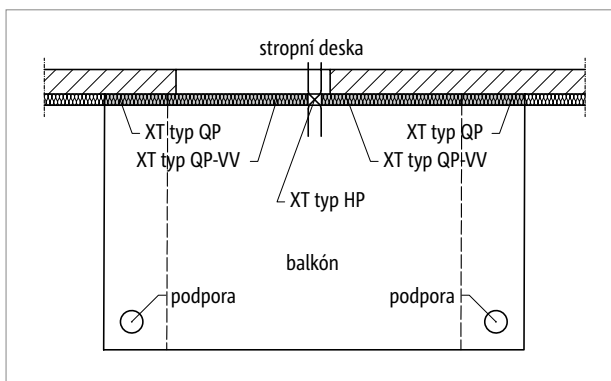
Obr. 117: Schöck Isokorb® XT typ QP, QL-VV: Balkón se sloupovými podporami, napojení s různými tuhostmi uložení; alternativně s prvkem XT typ HP pro přenos vodorovných sil
