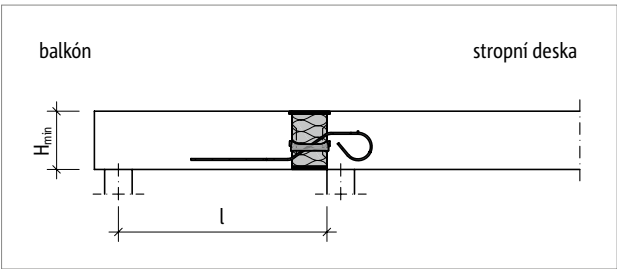
Obr. 122: Schöck Isokorb® XT typ QL: Statický systém (XT typ QL-V1 až V4)
