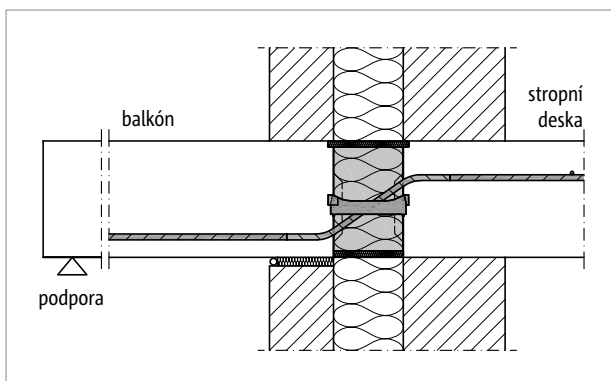
Obr. 119: Schöck Isokorb® XT typ QL: V kombinaci se sendvičovým zdivem (XT typ QL-V5 až V8)
