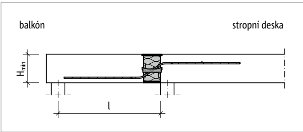
Obr. 123: Schöck Isokorb® XT typ QL: Statický systém (XT typ QL-V5 až V8)
