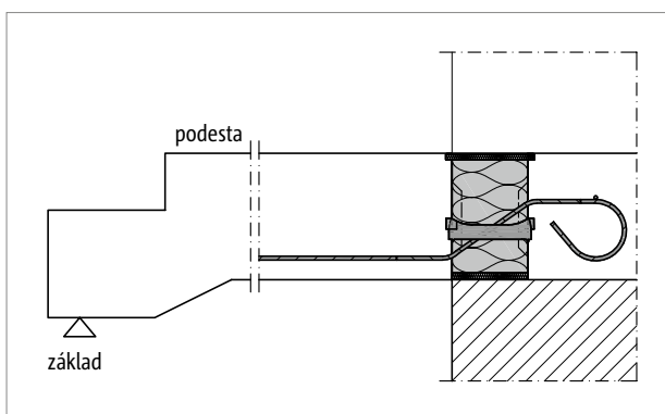
Obr. 121: Schöck Isokorb® XT typ QL: Podesta uložena na nezatepleném zdivu s dobrými tepelně-izolačními vlastnostmi (XT typ QL-V1 až V4)
