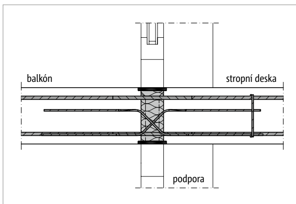
Obr. 192: Schöck Isokorb® T typ DP: Řez, bezprůvlaková stropní deska
