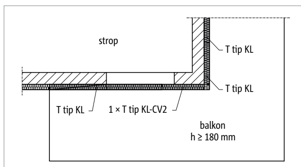
Sl. 52: Schöck Isokorb® T tip KL: balkoni na zunanjem vogalu
