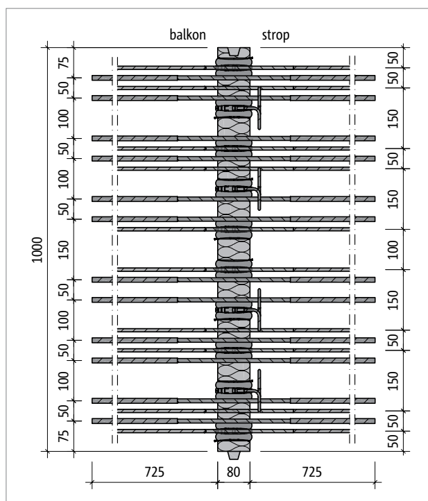
Sl. 63: Schöck Isokorb® T tip KL-M10-V2: tloris proizvoda
