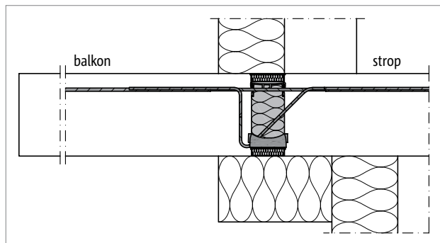
Sl. 56: Schöck Isokorb® T tip KL: priključek pri posredno uležanem stropu in sistemu s toplotno izolacijo
