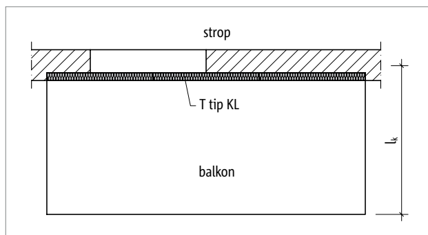
Sl. 50: Schöck Isokorb® T tip KL: nepodprt konzolni balkon
