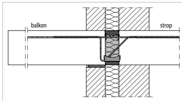
Sl. 57: Schöck Isokorb® T tip KL: dvojno opažni zid pri balkonu na nivoju notranje plošče
