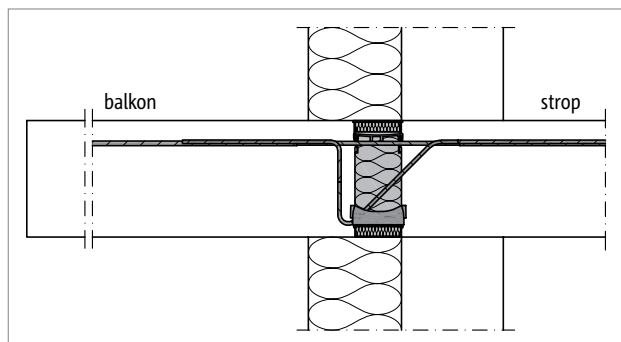
Sl. 54: Schöck Isokorb® T tip KL: zid z zunanjo izolacijo pri balkonu na nivoju notranje plošče
