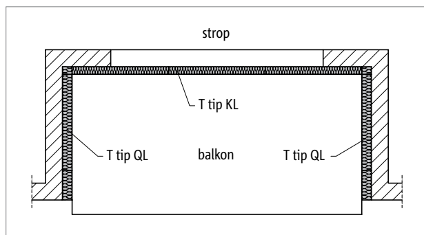
Sl. 51: Schöck Isokorb® T tip KL in tip QL: balkon s tristranskim naleganjem
