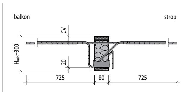
Sl. 61: Schöck Isokorb® T tip KL-M8 do M12: prerez proizvoda
