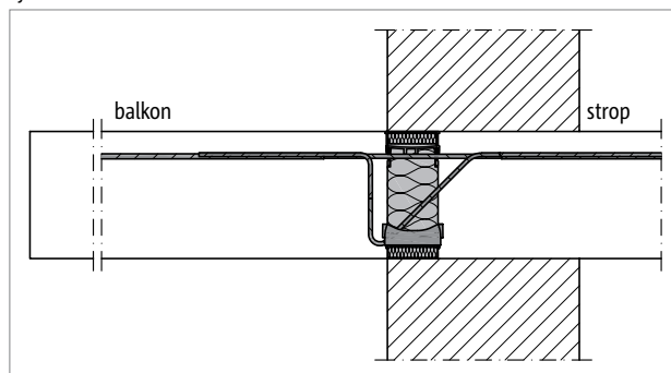
Sl. 55: Schöck Isokorb® T tip KL: enoopažni zid pri balkonu na nivoju notranje plošče
