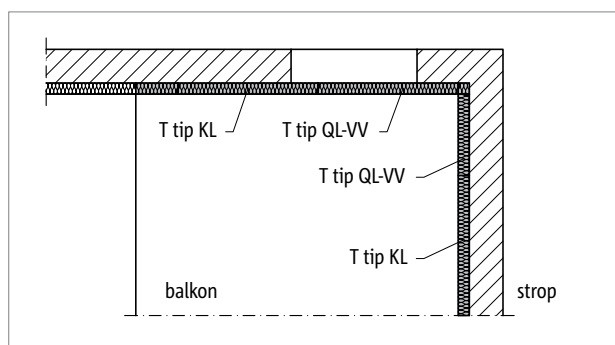
Sl. 53: Schöck Isokorb® T tipa KL in QL-VV: balkon z dvostranskim naleganjem
