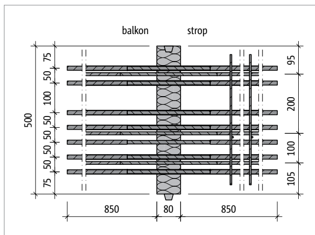
Sl. 67: Schöck Isokorb® T tip KP-M13-V1: tloris proizvoda
