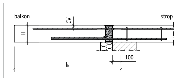
Sl. 58: Schöck Isokorb® T tip KP-M13 do M14: statični sistem
