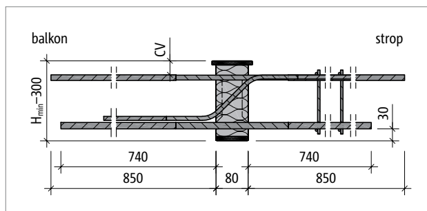
Sl. 66: Schöck Isokorb® T tip KP-M13 do M14-V1: prerez proizvoda
