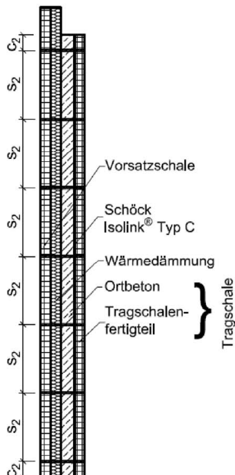
Abb. 5: Beispiel einer mehrschichtigen Fertigteilwand (Montagekennwerte und Schalendicken gemäß Anhang B2)
