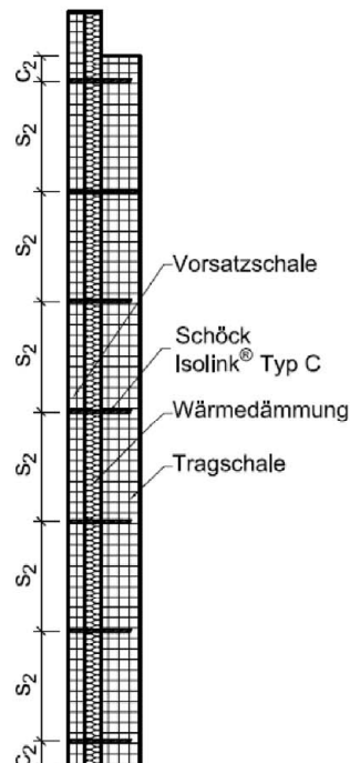
Abb. 5: Beispiel einer mehrschichtigen Fertigteilwand (Montagekennwerte und Schalendicken gemäß Anhang B2)
