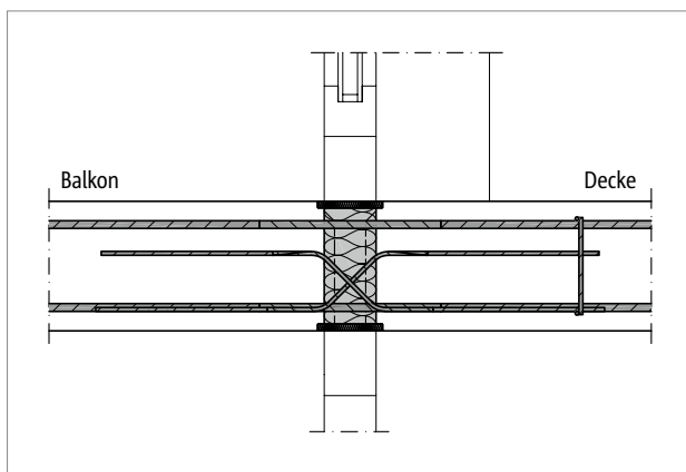
Abb. 205: Schöck Isokorb® T Typ DP: Einbauschritt; einachsrig gespannte Decke
