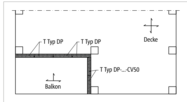
Abb. 204: Schöck Isokorb® T Typ DP: Einsatz in Flachdecken
