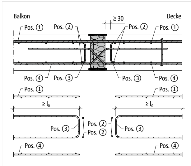
Abb. 214: Schöck Isokorb® T Typ DP: Bauseitige Bewehrung
