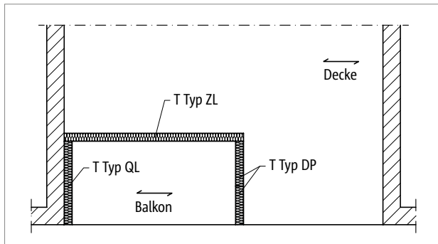
Abb. 203: Schöck Isokorb® T Typ DP, QL-Z, ZL: Decke einachsrig gespannt
