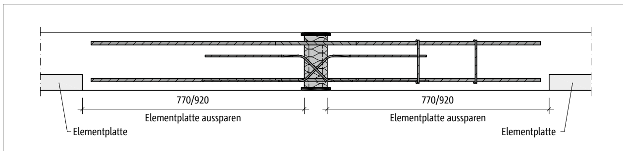
Abb. 216: Schöck Isokorb® T Typ DP: Ausgesparte Elementdecke mit eingesetztem Isokorb® T Typ DP
