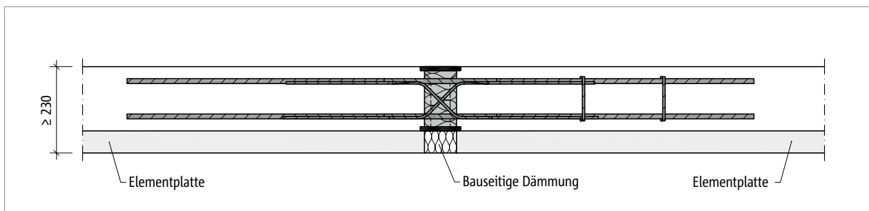
Abb. 217: Schöck Isokorb® T Typ DP: Elementdecke mit aufgesetztem Isokorb® T Typ DP
