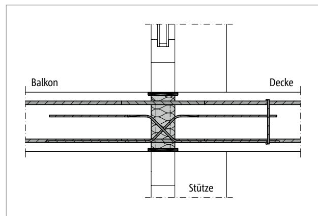
Abb. 206: Schöck Isokorb® T Typ DP: Einbauschritt; Flachdecke
