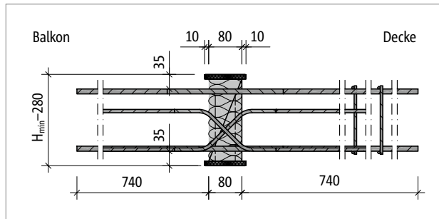
Abb. 210: Schöck Isokorb® T Typ DP-MM1-VV3 bei CV1: Produktschnitt
