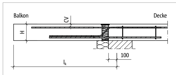
Abb. 58: Schöck Isokorb® T Typ KP-M13 bis M14: Statisches System
