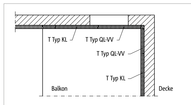
Abb. 53: Schöck Isokorb® T Typ KL und QL-VV: Balkon zweiseitig aufliegend
