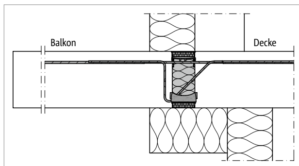
Abb. 56: Schöck Isokorb® T Typ KL: Anschluss bei indirekt gelagerter Decke und WDVS
