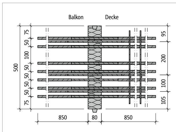
Abb. 67: Schöck Isokorb® T Typ KP-M13-V1: Produktgrundriss
