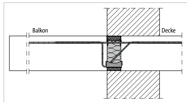
Abb. 55: Schöck Isokorb® T Typ KL: Einschaliges wärmedämmendes Mauerwerk bei deckengleichem Balkon
