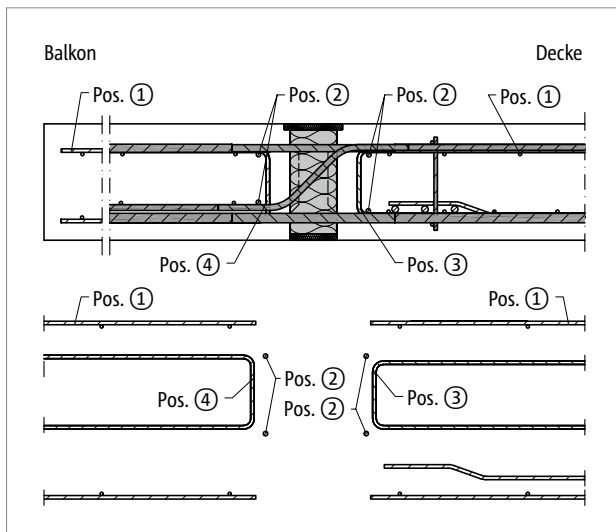
Abb. 70: Schöck Isokorb® T Typ KP-M13 bis M14: Bauseitige Bewehrung bei indirekter Lagerung
