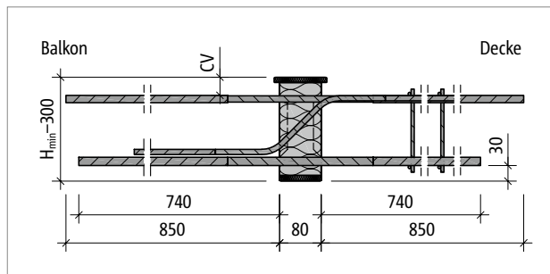
Abb. 66: Schöck Isokorb® T Typ KP-M13 bis M14-V1: Produktschnitt
