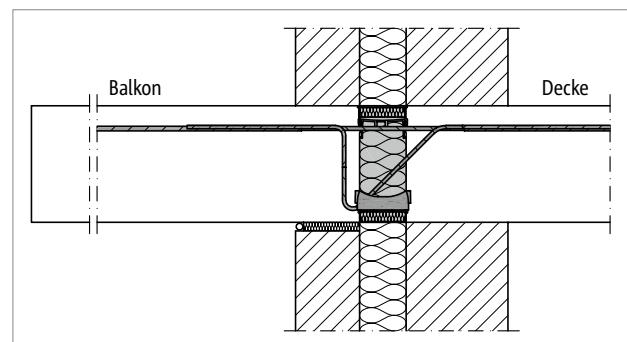
Abb. 57: Schöck Isokorb® T Typ KL: Anschluss bei zweischaligem Mauerwerk mit Kerndämmung
