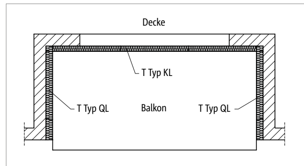
Abb. 51: Schöck Isokorb® T Typ KL und Typ QL: Balkon dreiseitig aufliegend
