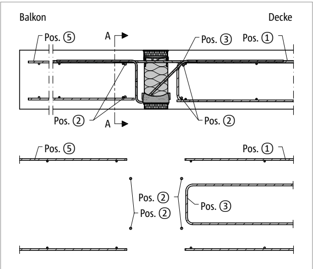
Abb. 69: Schöck Isokorb® T Typ KL: Bauseitige Bewehrung bei indirekter Lagerung
