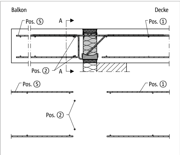
Abb. 68: Schöck Isokorb® T Typ KL: Bauseitige Bewehrung bei direkter Lagerung
