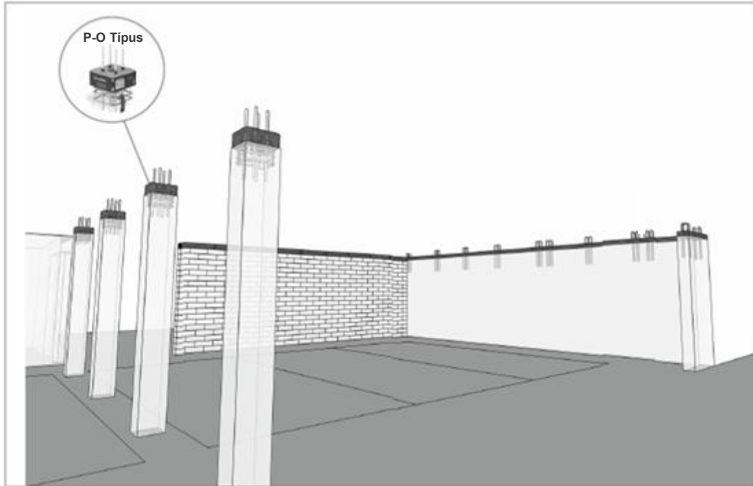
Sconnex® P-O típus elhelyezése a pillérfejnél, hőszigetelés a födém alsó síkján
