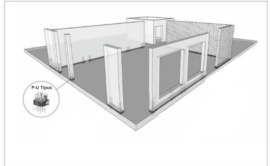
Sconnex® P-U típus elhelyezése a pillértalpnál, hőszigetelés a födém felső síkján
