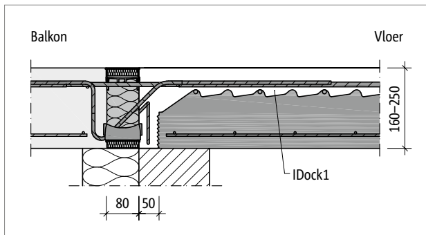
Afb. 5: Schöck Isokorf® T type K-E: Aansluiting van prefabbalkons met plaatdikten van 160 mm tot 250 mm met IDock1
