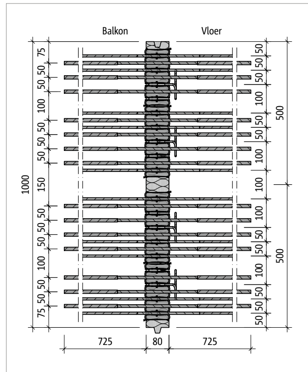
Afb. 58: Schöck Isokorf® T type K-T-M10-V1: Bovenaanzicht
