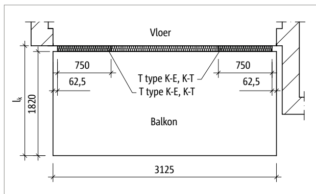
Afb. 7: Schöck Isokorf® T type K-E, K-T: Schöck Isokorf® T type K-E, K-T:
