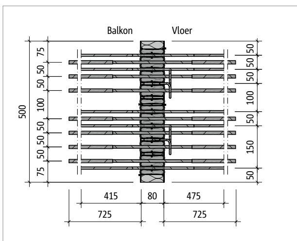
Afb. 62: Schöck Isokorf® T type K-T-M10: Productschets van de variant met lengte L500
