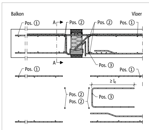
Afb. 64: Schöck Isokorf® T type K-E, K-T: Bijlegwapening; vloerplaat met randbalk
