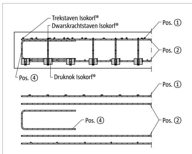
Afb. 65: Schöck Isokorf® T type K-E, K-T: Bijlegwapening aan de balkonzijde in doorsnede A-A; pos.4 = Randwapening aan de vrije rand loodrecht op Schöck Isokorf®
