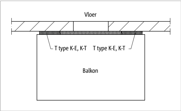
Afb. 39: Schöck Isokorf® T type K-E, K-T: vrij uitkragend balkon
