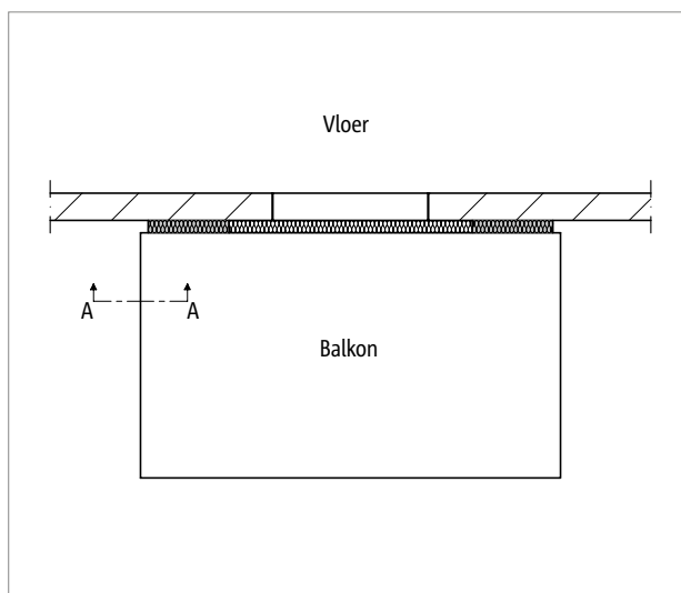
Afb. 66: Schöck Isokorf® T type K-E, K-T: Doorsnede A-A
