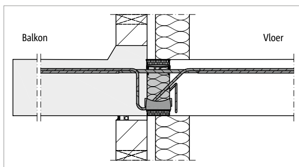
Afb. 46: Schöck Isokorf® T type K-E, K-T: aansluiting prefabbalkon; de vloerhoogte komt overeen met de hoogte van de Schöck Isokorf®
