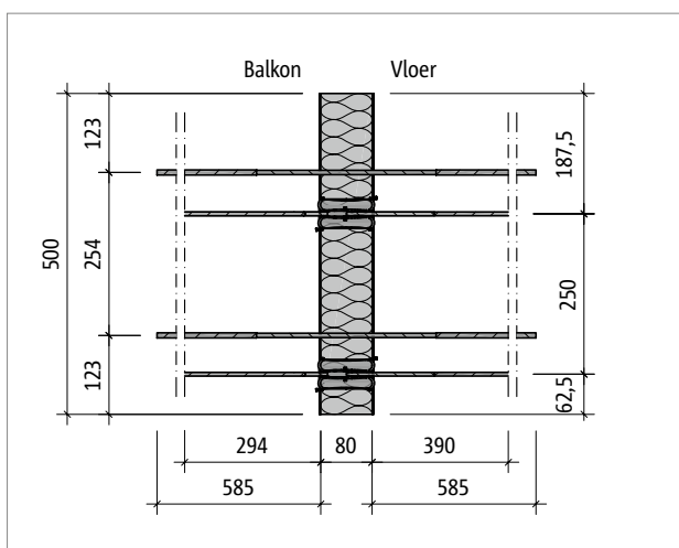
Afb. 61: Schöck Isokorf® T type K-T-M1: Productschets van de variant met lengte L500
