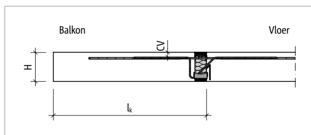
Afb. 1: Schöck Isokorf® T type K-E, K-T: Statisch systeem
