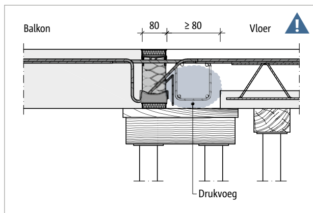
Afb. 4: Schöck Isokorf® T type K-E, K-T: Inbouw bij een vloerplaat met breedplaatvloer en randbalk, drukvoeg in de vloerplaat
