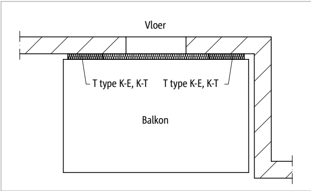
Afb. 40: Schöck Isokorf® T type K-E, K-T: balkon bij verspringende gevel
