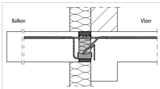
Afb. 44: Schöck Isokorf® T type K-E, K-T: Aansluiting bij randbalk en ETICS
