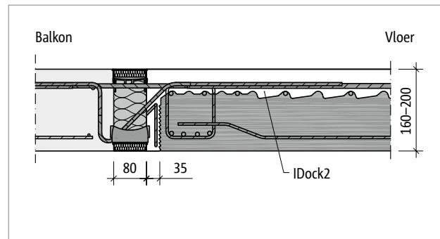
Afb. 6: Schöck Isokorf® T type K-E: Aansluiting van prefabbalkons met plaatdikten van 160 mm tot 200 mm met IDock2
