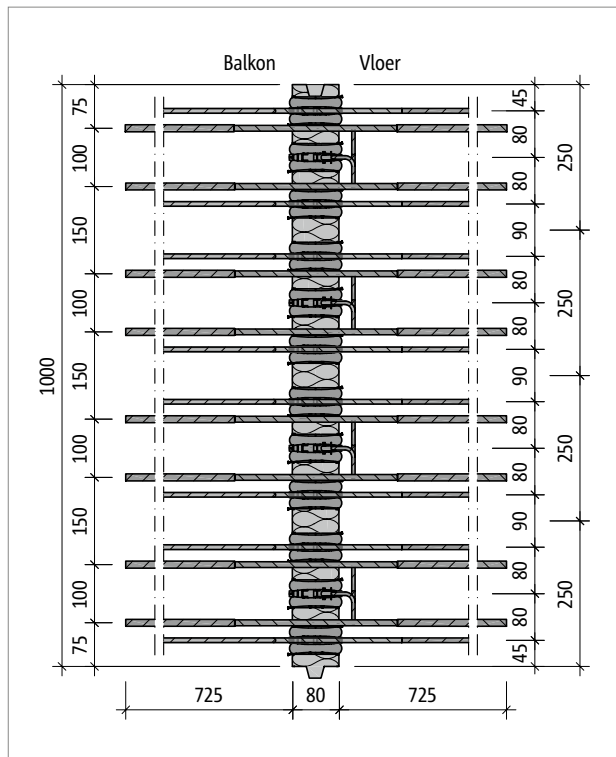
Afb. 57: Schöck Isokorf® T type K-E-M6: Bovenaanzicht
