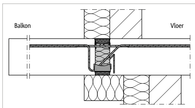
Afb. 45: Schöck Isokorf® T type K-E, K-T: Aansluiting bij indirect ondersteunde vloerplaat en ETICS
