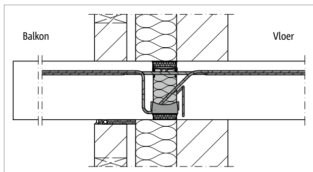
Afb. 43: Schöck Isokorf® T type K-E, K-T: Aansluiting bij geïsoleerde spouw
