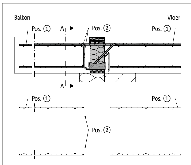
Afb. 63: Schöck Isokorf® T type K-E, K-T: Bijlegwapening; vloerplaatrand met opleg op wand
