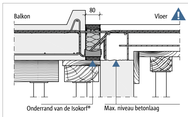
Afb. 2: Schöck Isokorf® T type K-E, K-T: Prefabbalkon met verhoogde vloerplaat op een wand van gewapend beton
