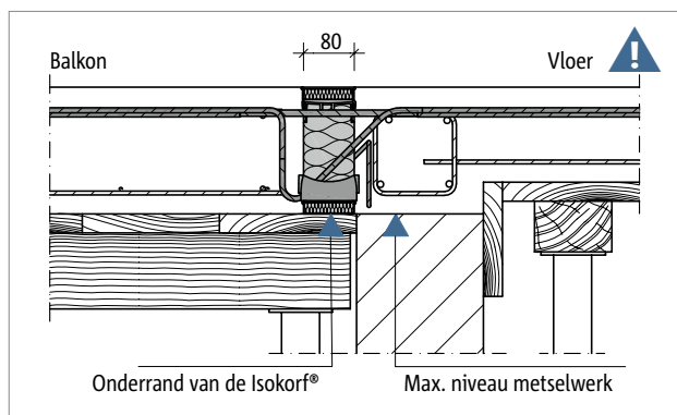
Afb. 1: Schöck Isokorf® T type K-E, K-T: Balkon in ter plaatse gestort beton met verhoogde vloerplaat op metselwerkwand
