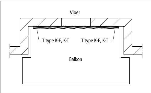
Afb. 41: Schöck Isokorf® T type K-E, K-T: balkon bij achteruitspringende gevel
