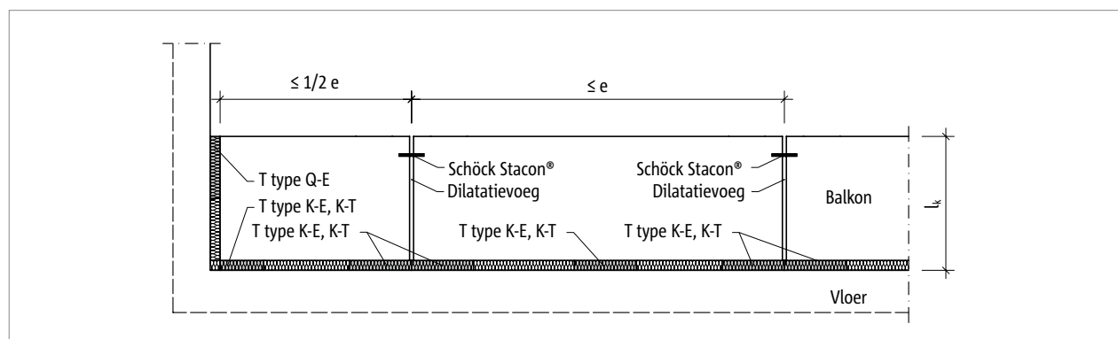
Afb. 2: Schöck Isokorf® T type K-E, K-T: Vereiste uitzetvoegen
