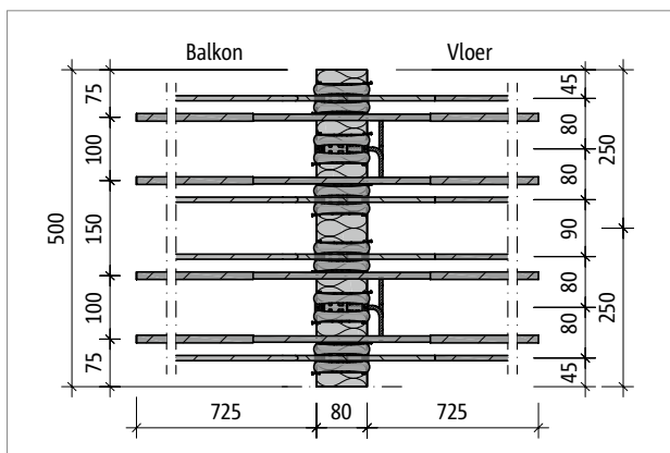
Afb. 59: Schöck Isokorf® T type K-E-M6: Boveanaanzicht van de variant lengte L500
