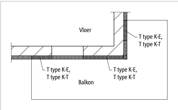
Afb. 42: Schöck Isokorf® T type K-E, K-T: hoekbalkon
