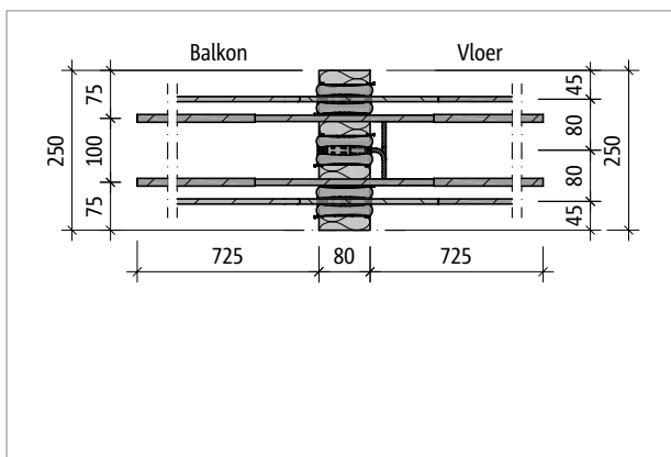
Afb. 60: Schöck Isokorf® T type K-E-M6: Boveanaanzicht van de variant lengte L250
