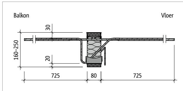
Afb. 55: Schöck Isokorf® T type K-E-M6, K-T-M7, -M9, -M10: Zijaanzicht
