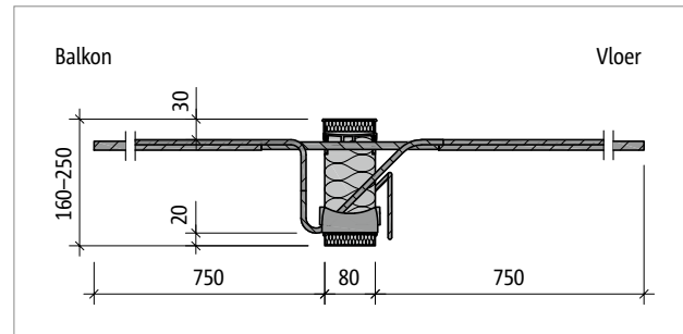
Afb. 56: Schöck Isokorf® T type K-E-M8: Zijaanzicht
