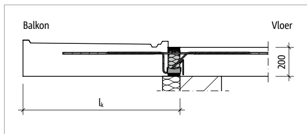
Afb. 8: Schöck Isokorf® T type K-E, K-T: statisch systeem, doorsnede
