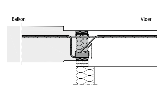
Afb. 47: Schöck Isokorf® T type K-E, K-T: aansluiting prefabbalkon; de vloerhoogte is groter dan de hoogte van de Schöck Isokorf®
