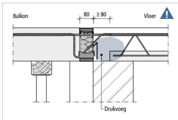
Afb. 3: Schöck Isokorf® T type K-E, K-T: Inbouw bij een vloerplaat met breedplaatvloer en wand opleg, drukvoeg in de vloerplaat
