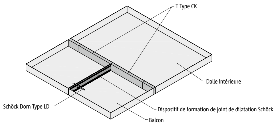
Fig. 23: Schöck Isokorb® Type CK : le dispositif de formation de joint de dilatation
