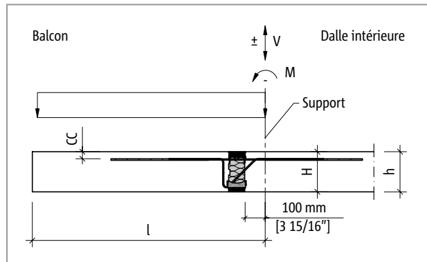
Fig. 20: Schöck Isokorb® T Type CK : système structurel
