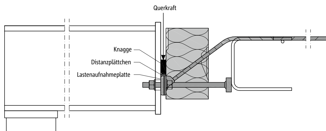
Abb. 78: Schöck Isokorb® XT Typ SQP: Bauseitige Knagge zur Übertragung der Querkraft
