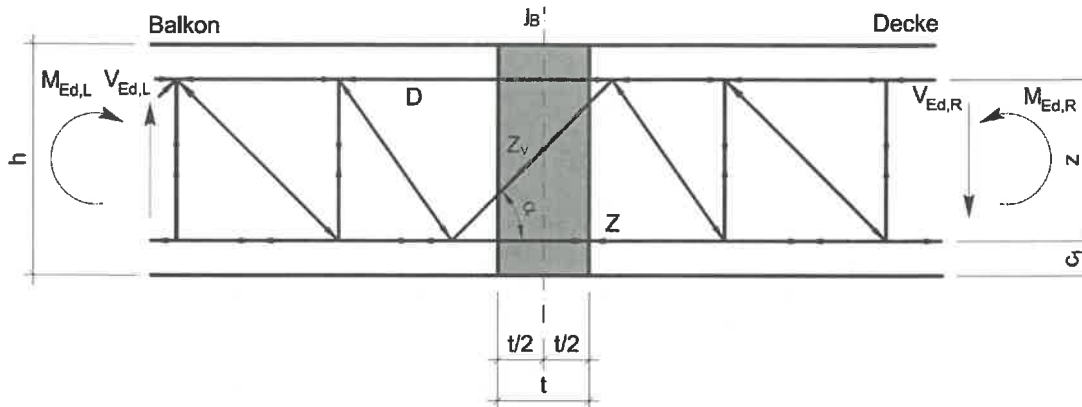
Bild 2-6: Fachwerkmodell Schöck Isokorb® Typ D: oben Druck, |V_{Ed,L}| < |V_{Ed,R}|
