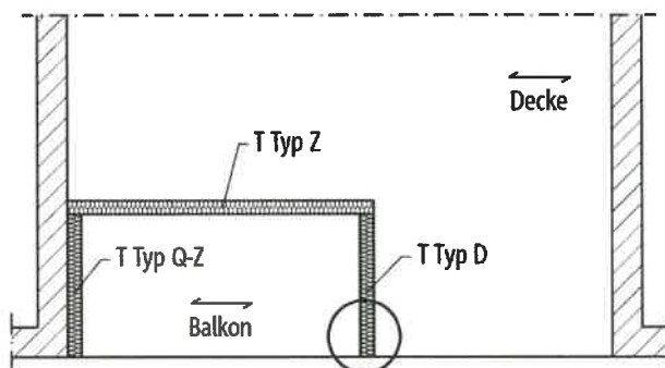
Bild 1-1: Einbausituation (Schöck Isokorb® T Typ D)
