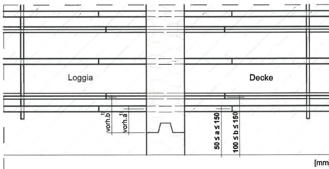
Bild 1-2: Rand- und Dehnfugenabstände der Zug-, Druck- und Querkraftstäbe (Schöck Isokorb® T Typ D)
