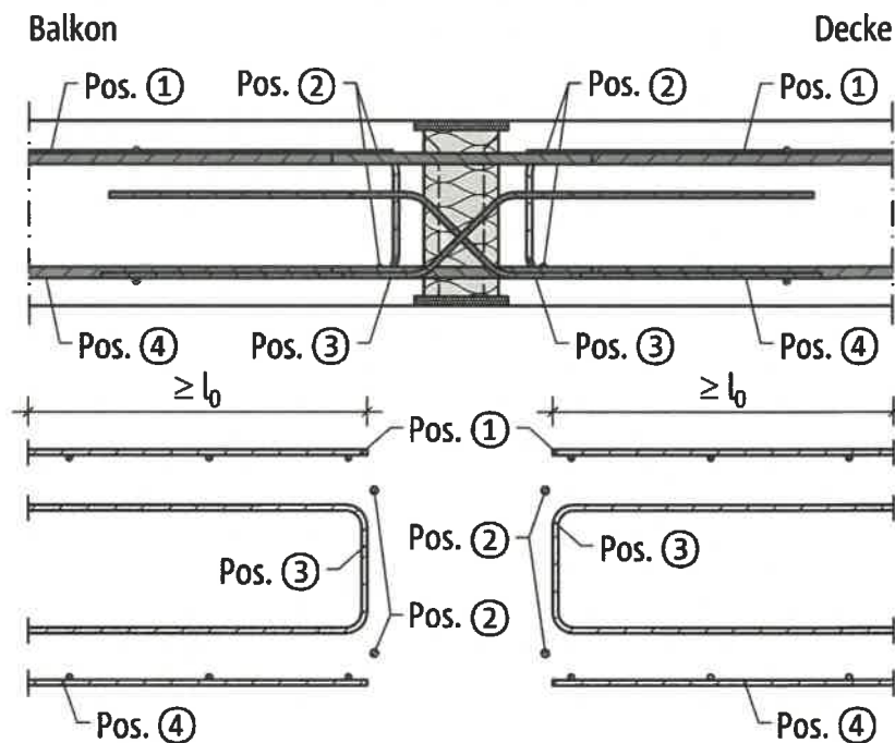
Bild 2-1: Schematische Darstellung der bauseitigen Anschlussbewehrung
