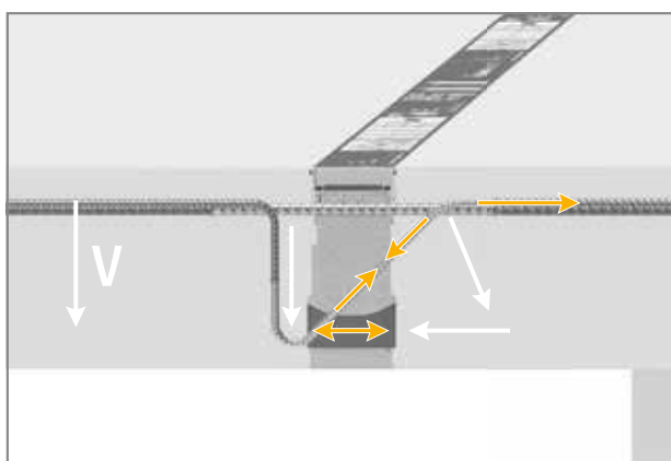
Sl. 16: Schöck Isokorb® tip K: prenašanje prečne sile
