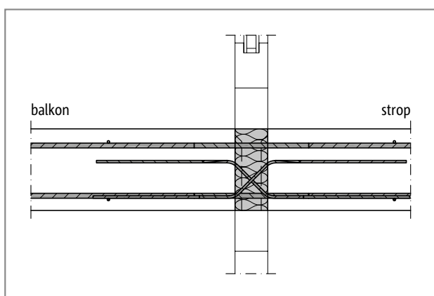
Sl. 139: Schöck Isokorb® tip D: prerez pri vgrajevanju, enosno vpet strop
