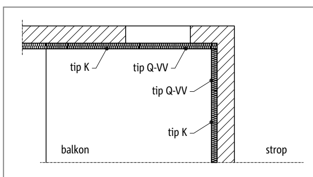
Sl. 60: Schöck Isokorb® tipa K in K-VV: balkon z dvostranskim naleganjem
