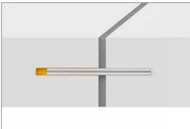
Sl. 39: Schöck Dorn: izdelava dilatacijskega stika
