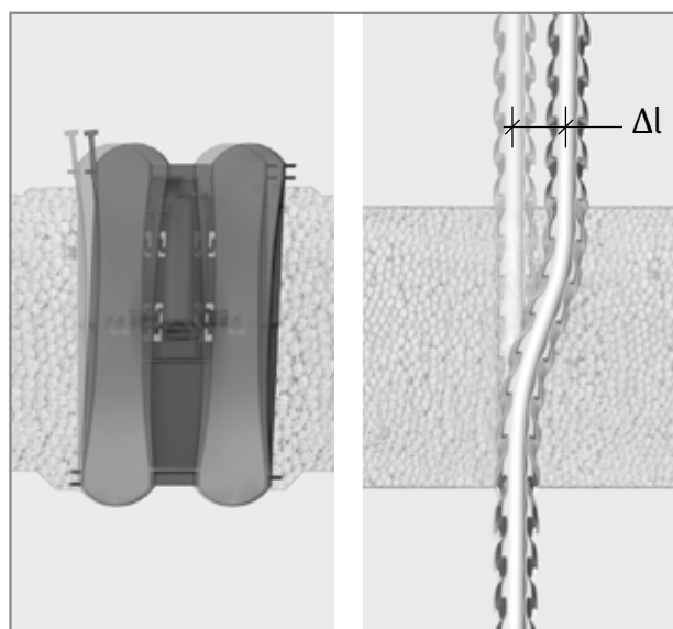
Sl. 38: Schöck Isokorb®: deformacije natezne palice in tlačnega ležaja HTE-Compact® pri toplotni obremenitvi
