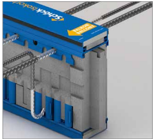
Sl. 6: Schöck Isokorb® tip K: balkonska puščica kaže smer vgrajevanja
