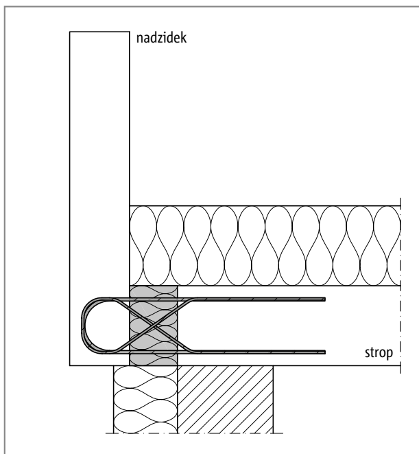
Sl. 180: Schöck Isokorb® tip ABXT za vodoravno namestitev: priključek nadzidka
