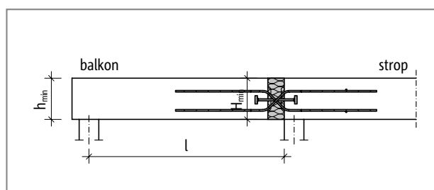
Sl. 115: Schöck Isokorb® tipi QP70L-VV do QP80L-VV: statični sistem
