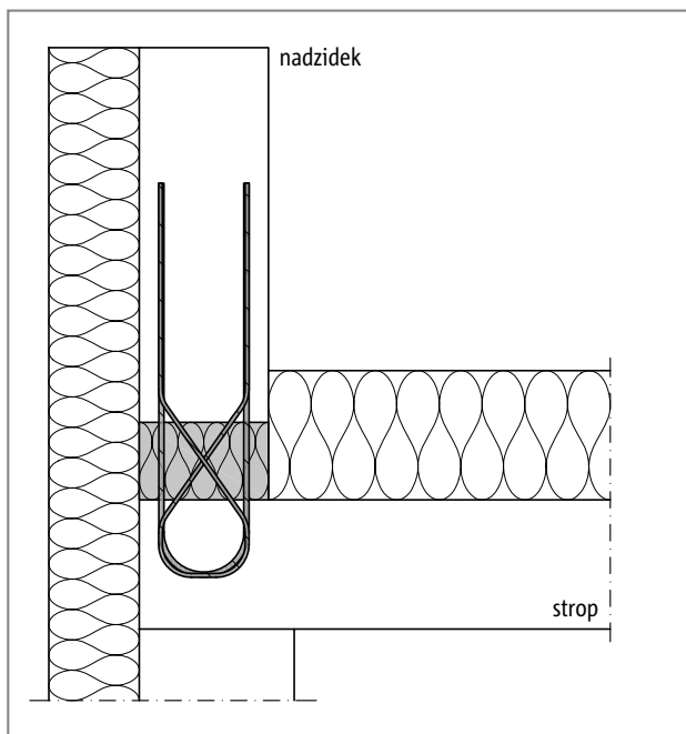
Sl. 179: Schöck Isokorb® tip ABXT za navpično namestitev: priključek atike
