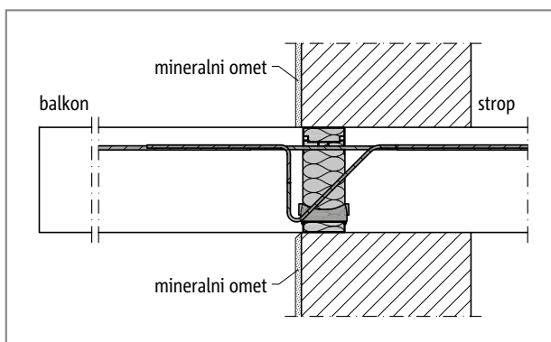
Sl. 198: Schöck Isokorb® tip K: izvedba REI30 na steni na primeru tipa K
