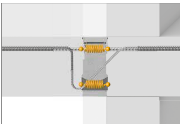
Sl. 31: Schöck Isokorb®: natezna palica in tlačni modul delujeta kot vzmeti
