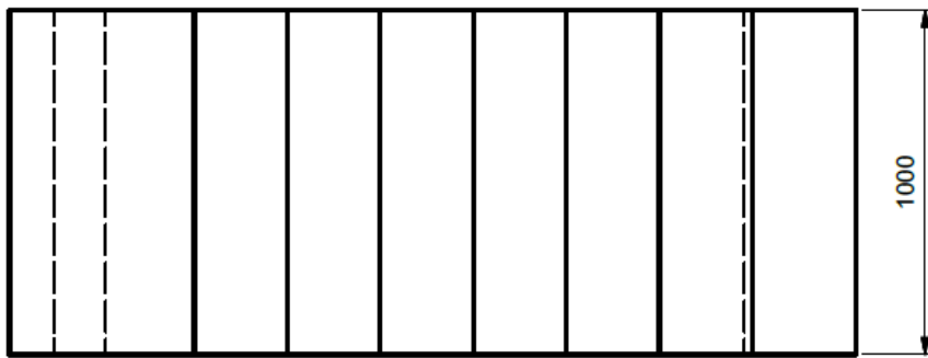
Abbildung 4: Draufsicht und Ansicht des Referenztreppenlaufes (alle Maße in mm)
