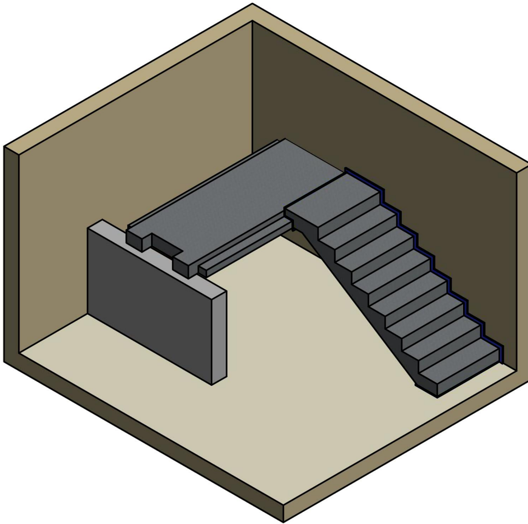
Abbildung 2: 3-D Ansicht des Prüfaufbaus
