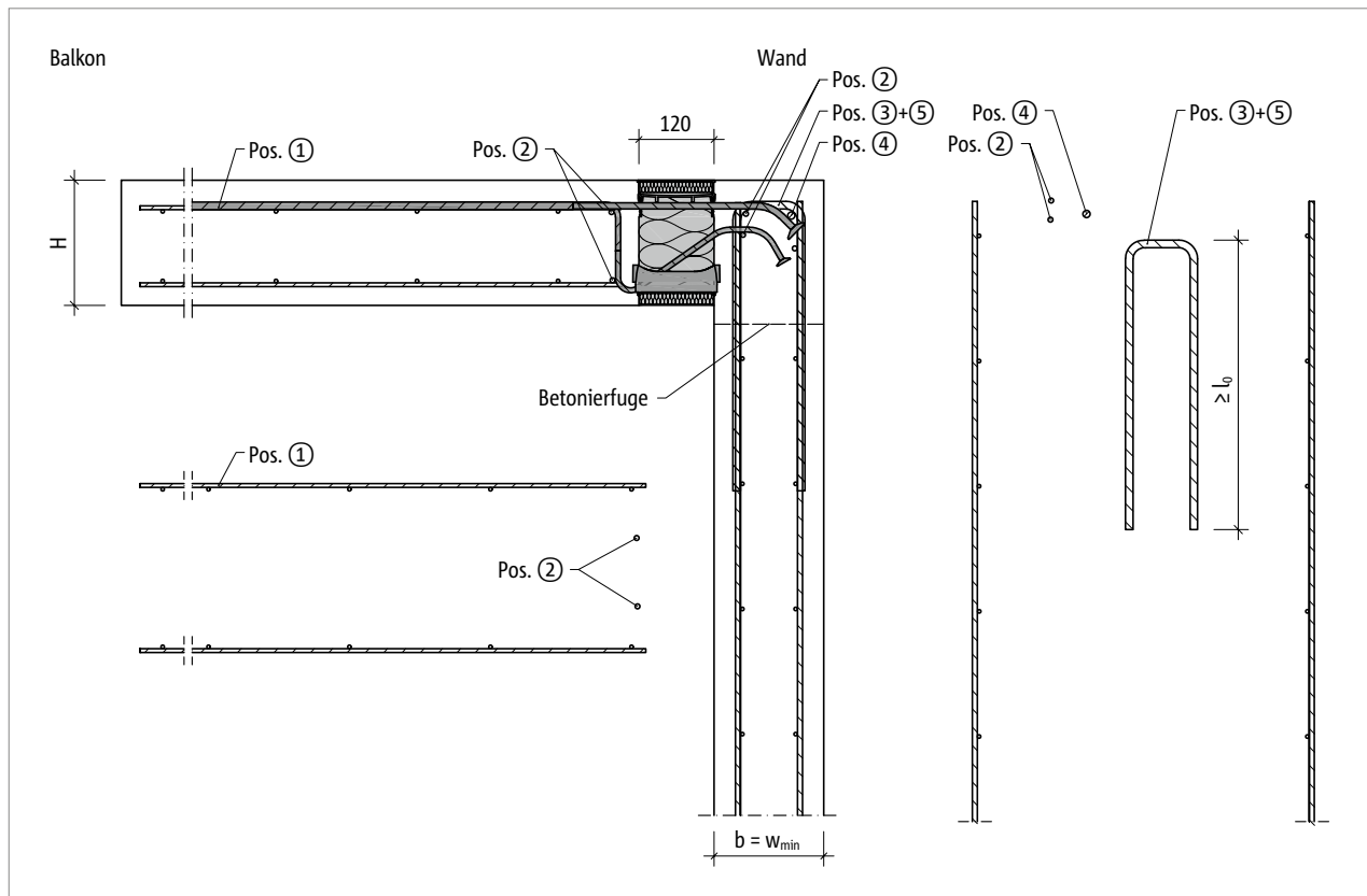
Abb. 118: Schöck Isokorb® XT Typ K-O: Bauseitige Bewehrung für Wandanschluss nach unten mit minimaler Bauteilabmessung ( w_{\text{vorh}} = w_{\min} )
