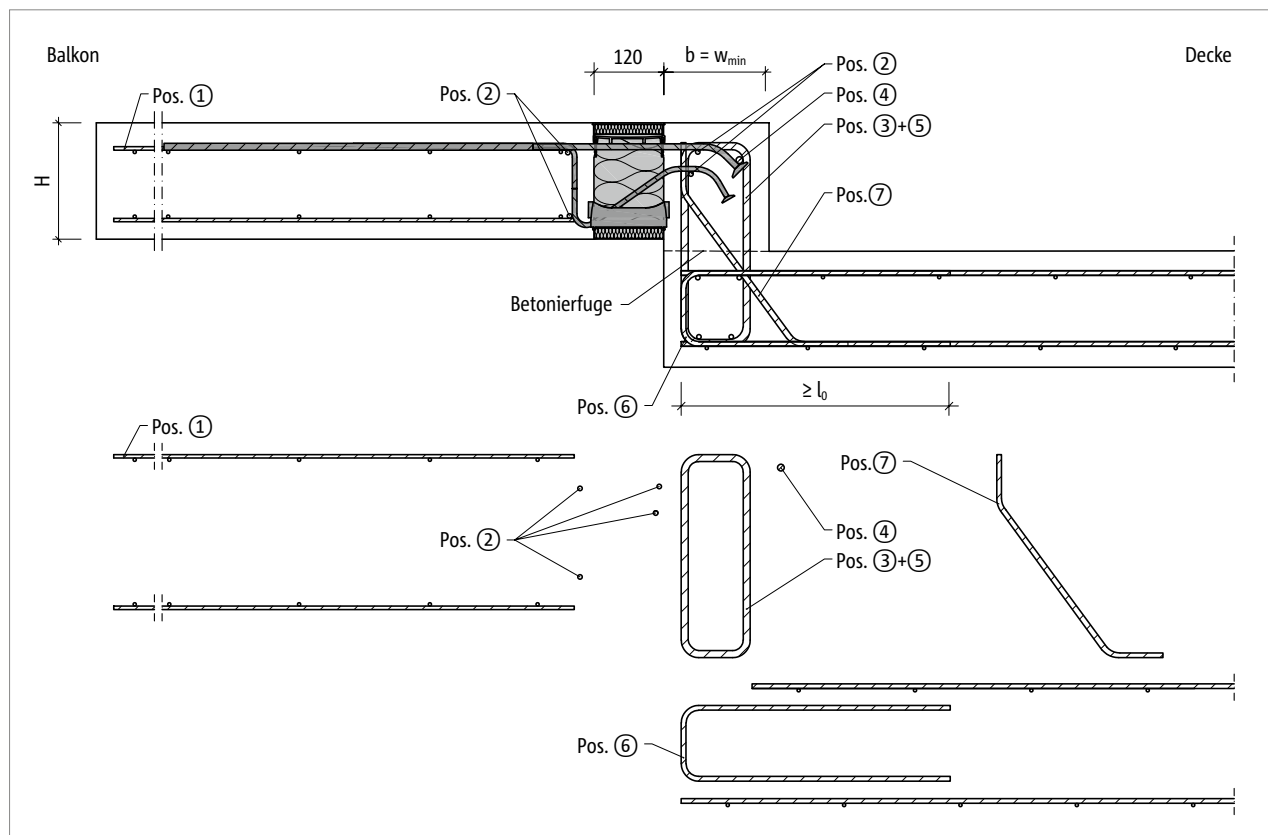
Abb. 116: Schöck Isokorb® XT Typ K-O: Bauseitige Bewehrung für Balkon mit Höhenversatz nach oben mit minimaler Bauteilabmessung ( w_{vorh} = w_{min} )
