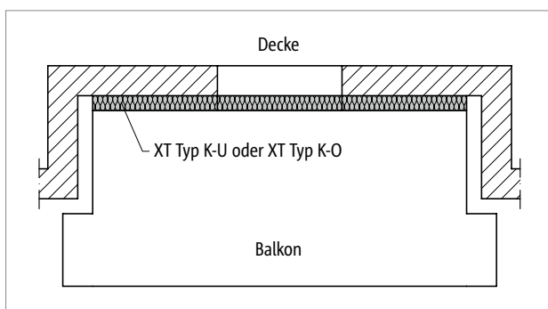
Abb. 87: Schöck Isokorb® XT Typ K-U/K-O: Balkon bei Fassadenvorsprung
