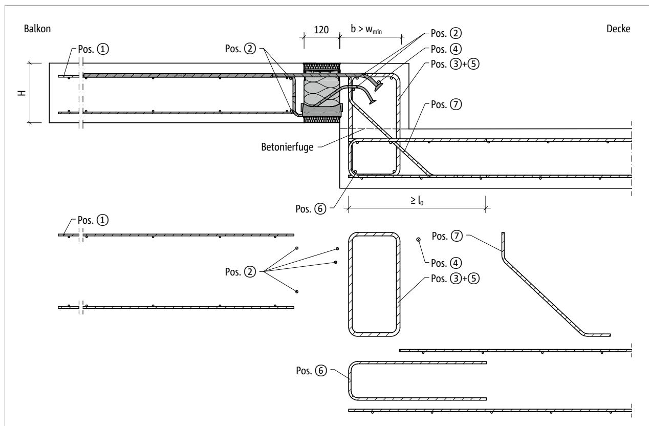
Abb. 117: Schöck Isokorb® XT Typ K-O: Bauseitige Bewehrung für Balkon mit Höhenversatz nach oben mit größerer Bauteilabmessung ( w_{vorh} > w_{min} )
