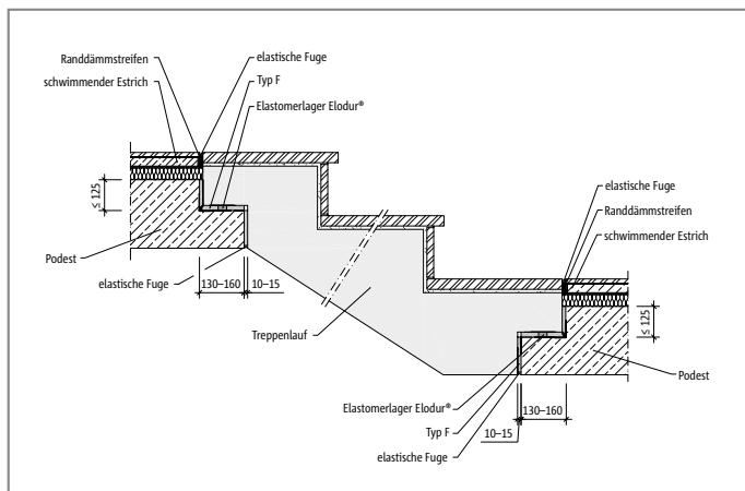
Abb. 22: Schöck Tronsole® Typ F: Einbauschnitt
