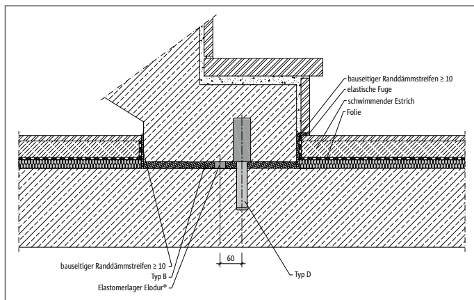
Abb. 24: Schöck Tronsole® Typ B + Typ D: Einbauschnitt
