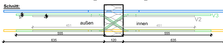
Schöck Isokorb XT_D-MM2-VV1 bis XT_D-MM5-VV3
