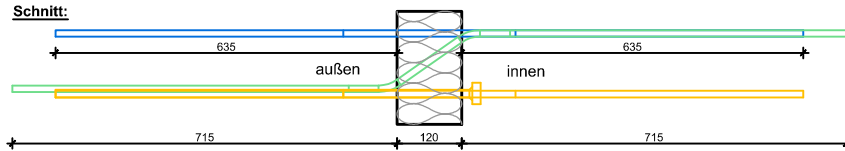
Schöck Isokorb XT_C-L(R)-M2-V2 (=max. Stablängen)
