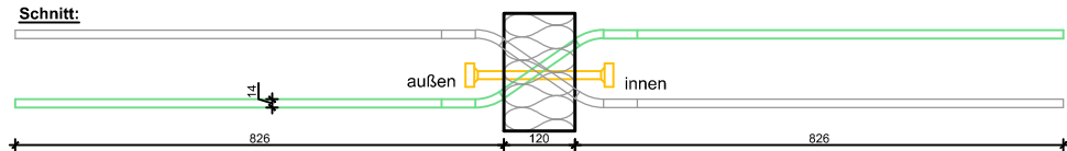
Schöck Isokorb XT_Q-V(V)11 + XT_Q-P-V(V)6 bis V(V)10
