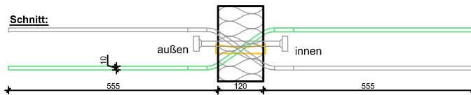
Schöck Isokorb XT_Q-V(V)6 bis XT_Q-V(V)9 + XT_Q-P-V(V)1 bis XT_Q-P-V(V)3
