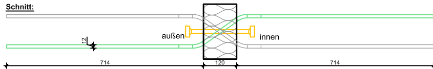
Schöck Isokorb XT_Q-V(V)10 + XT_Q-P-V(V)4 und XT_Q-P-V(V)5
