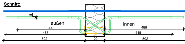
Schöck Isokorb XT_K(-F)-M3-VV bis XT_K(-F)-M5-VV
