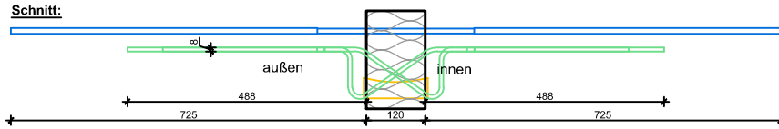
Schöck Isokorb XT_K(-F)-M6-VV bis XT_K(-F)-M8-VV
