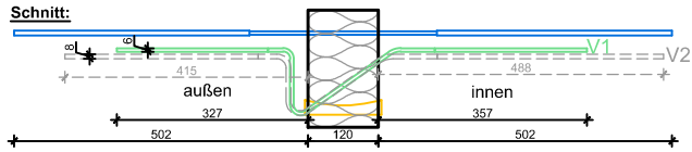
Schöck Isokorb XT_K(-F)-M1-V1/V2 bis XT_K(-F)-M6-V1/V2
