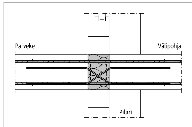
Schöck Isokorb® DXT: Tasokuva, välipohja
