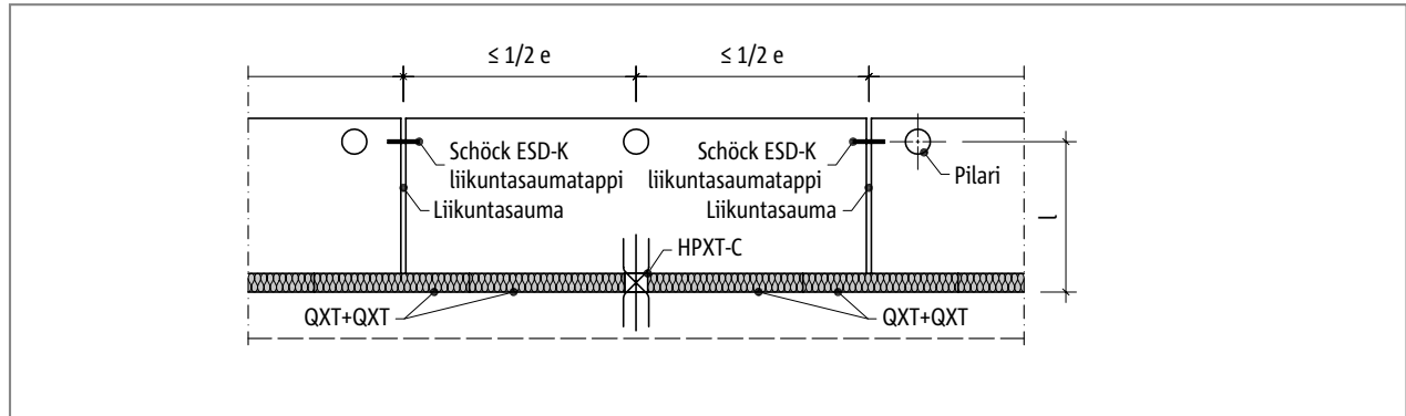
Schöck Isokorb® HPXT: Liikuntasauman valmistus pituussuunnassa työnnettävän liikuntasaumatapin avulla, esim. Schöck ESD-K-liikuntasaumatappi
