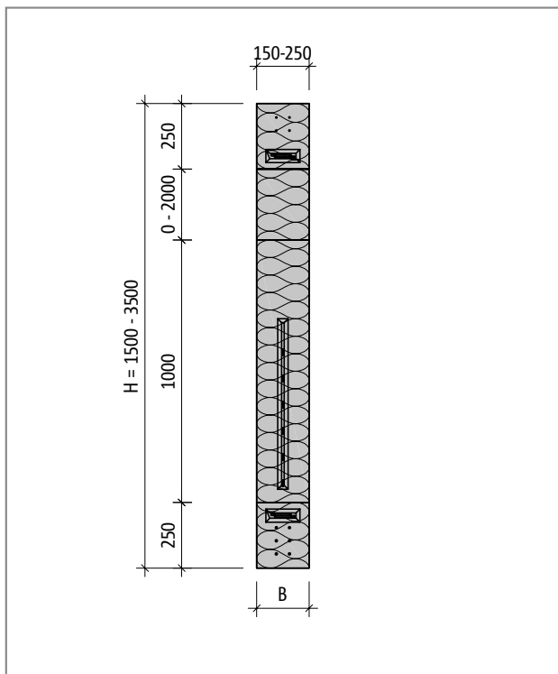
Schöck Isokorb® WXT1: Tuotenäkymä
