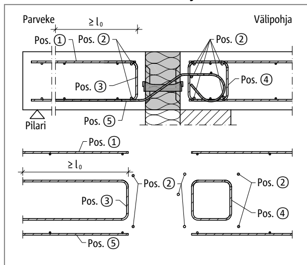
Schöck Isokorb® QXT10 - QXT40: Liittyvä raudoitus
