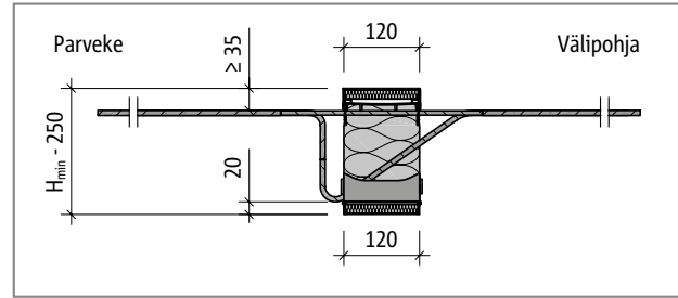
Schöck Isokorb® KXT45 ja KXT50, REI120: Leikkaus
