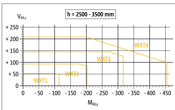
Schöck Isokorb® WXT: Interaktiogrammi C25/30 H = 2500 - 3500
