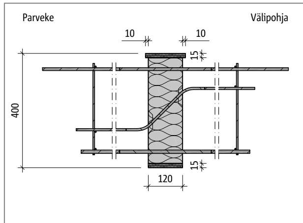
Schöck Isokorb® SXT1, R90: Leikkaus, palosuojalevyt ympäriinsä
