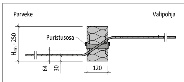
Schöck Isokorb® QXT60 - QXT90: Leikkaus
