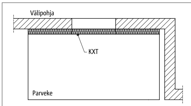
Schöck Isokorb® KXT: Nurkkaparveke ulokkeena
