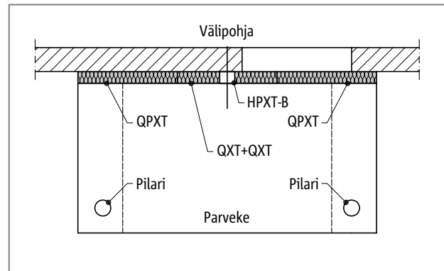
Schöck Isokorb® QPXT ja QXT+QXT: Pilareilla tuettu parveke, liitos erilaisilla vaakajäykistyksillä (esimerkiksi tyyppi HPXT-B kanssa vaakasuuntaisten kuormitusten siirtämiseen).
