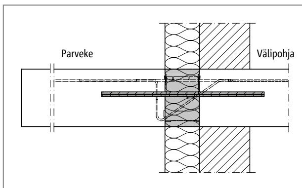
Schöck Isokorb® KXT ja HPXT-A: Rapattu seinärakenne, ulkoeriste
