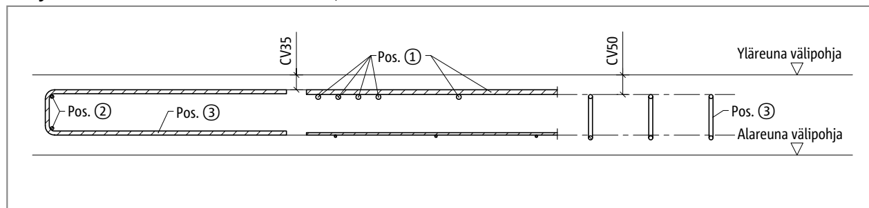
Schöck Isokorb® EXT: Liittyvä raudoitus, ulkonurkka (leikkaus EXT-L-CV35, näkymä EXT-R-CV50)
