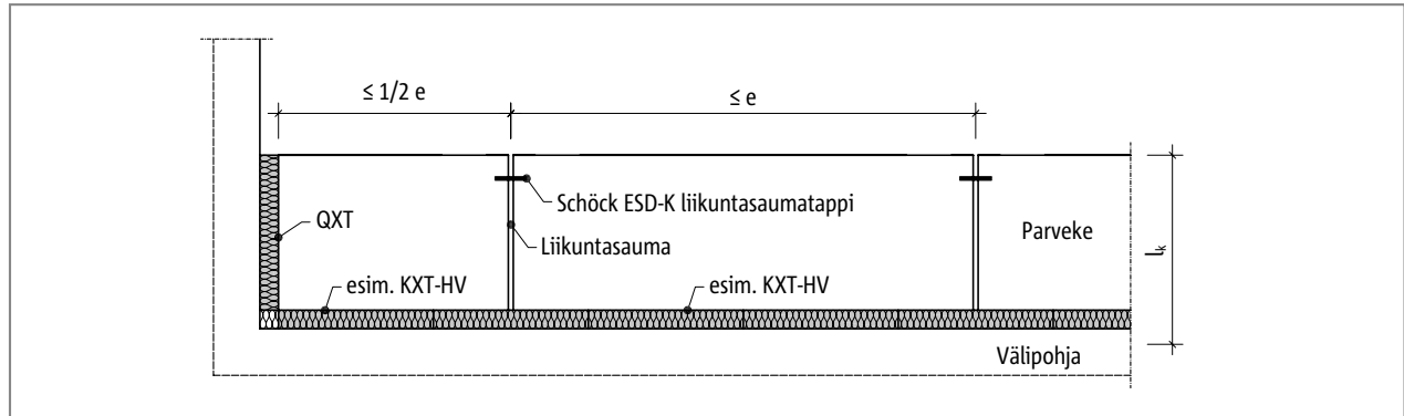
Schöck Isokorb® KXT-HV: Liikuntasauman valmistus pituussuunnassa työnnettävän liikuntasaumatapin avulla, esim. Schöck ESD-K-liikuntasaumatappi
