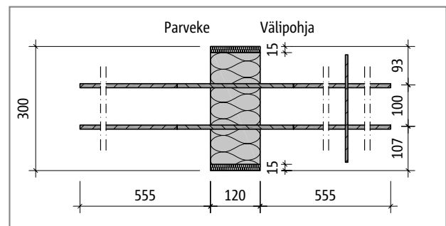
Schöck Isokorb® QPZXT10, REI90: Tasokuva
