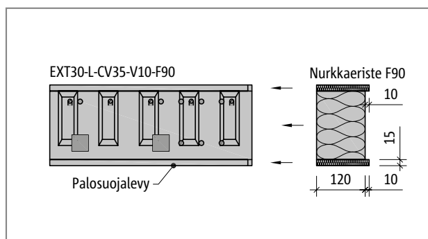
Schöck Isokorb® EXT30-L-CV35, REI90: Tuotenäkymä
