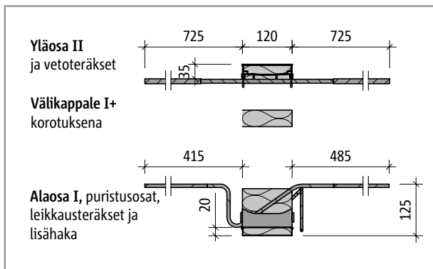
Schöck Isokorb® KFXT65-CV35-V8 (KFXT50-CV35 ilman lisähakaa)
