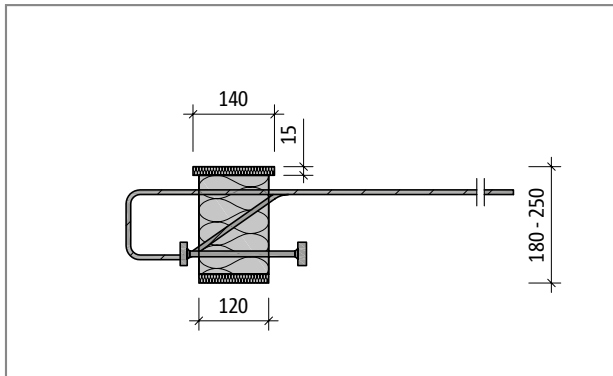
Schöck Isokorb® OXT: Leikkaus, R90, palosuojauslevyt ylhäällä ja alhaalla
