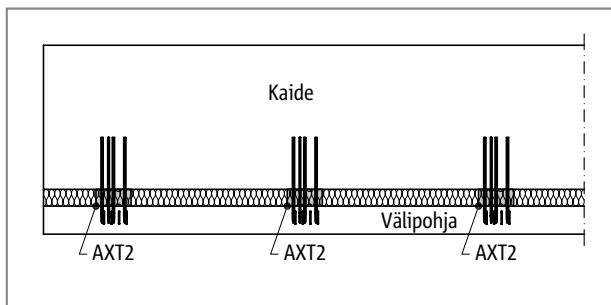
Schöck Isokorb® AXT2: Kaide
