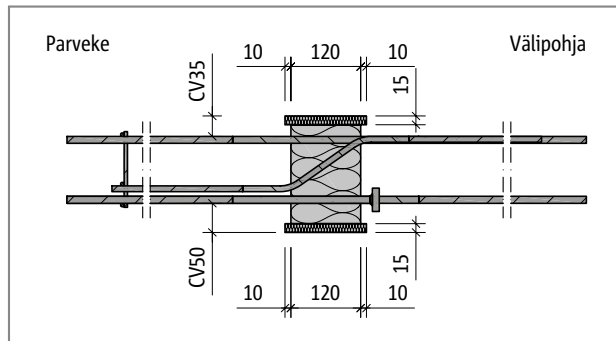
Schöck Isokorb® EXT30-CV35, REI90: Leikkaus
