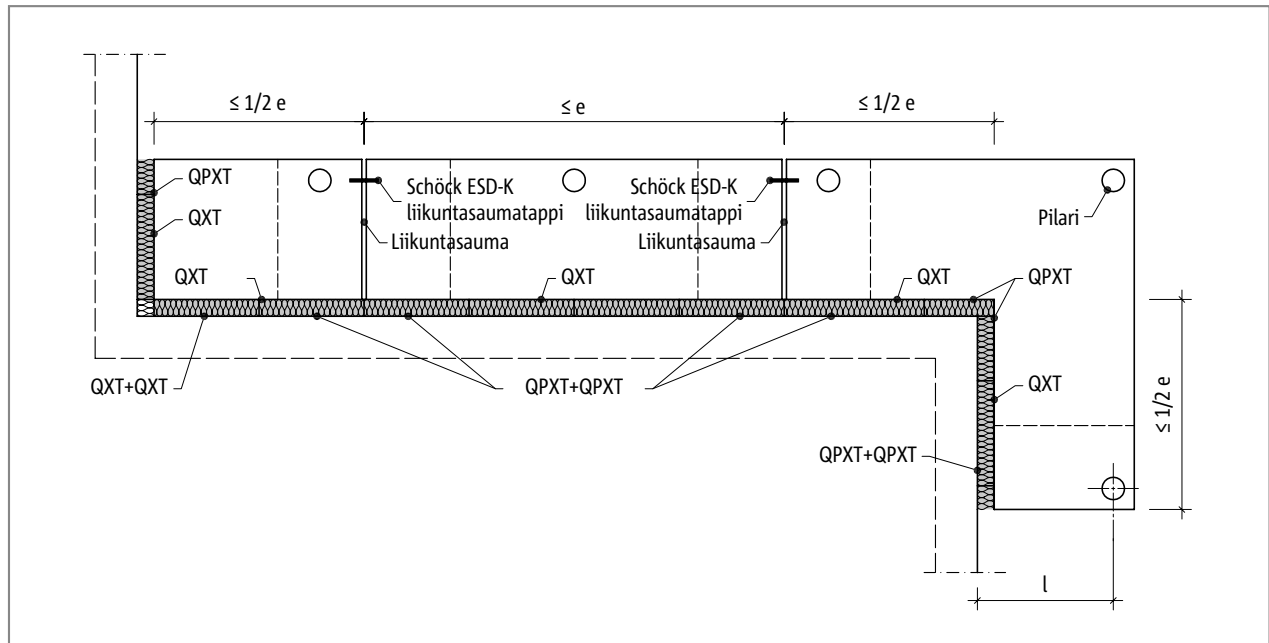
Schöck Isokorb® QPXT ja QPXT+QPXT: Liikuntasauman valmistus pituussuunnassa liikkuvan liikuntasaumatapin avulla, esim. Schöck ESD-K liikuntasaumatappi
