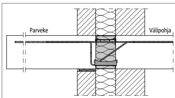
Schöck Isokorb® KXT: Sandwich-verhottu ulkoseinä ja ulokeparveke
