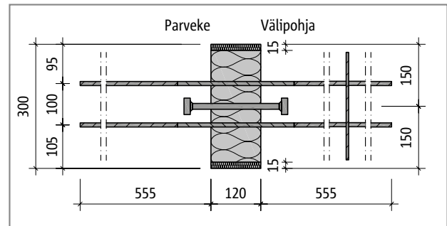
Schöck Isokorb® QPXT10, REI90: Tasokuva
