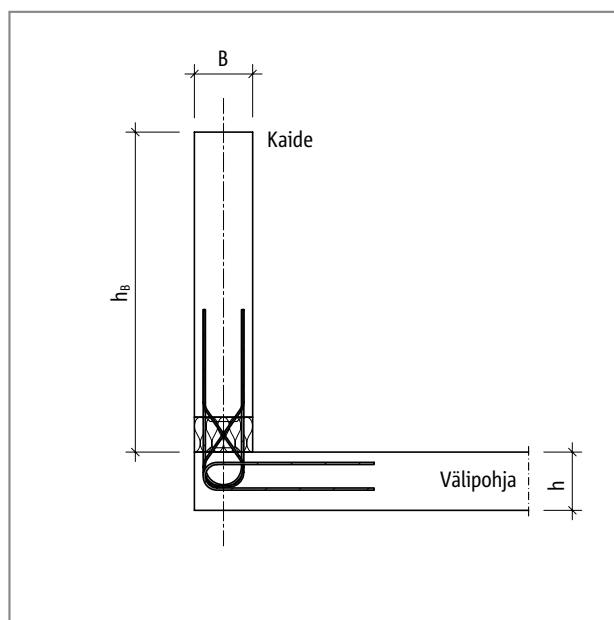
Schöck Isokorb® AXT: Staattinen järjestelmä
