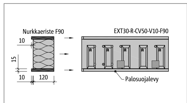
Schöck Isokorb® EXT30-R-CV50, REI90: Tuotenäkymä
