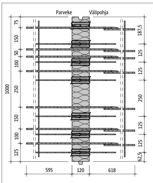
Schöck Isokorb® KXT30-HV: Tasokuva
