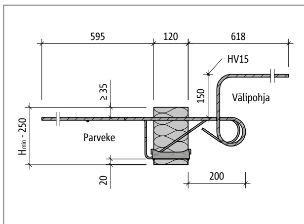
Schöck Isokorb® KXT30-HV15: Leikkaus
