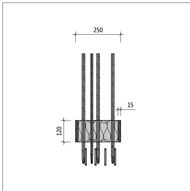
Schöck Isokorb® AXT2, R90: Sivunäkymä, palosuojalevyt sivuilla
