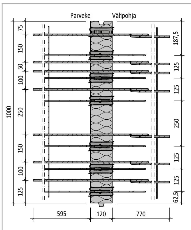
Schöck Isokorb® KXT30-BH: Tasokuva
