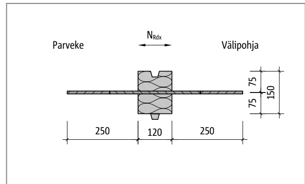
Schöck Isokorb® HPXT-B: Tasokuva
