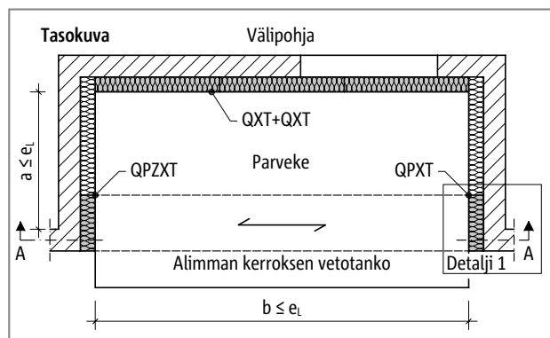
Schöck Isokorb® QPXT, QPXT: Sisäänvedetyn parvekkeen tasokuva
