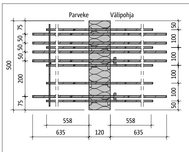
Schöck Isokorb® EXT30-L: Tasokuva
