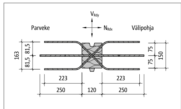
Schöck Isokorb® HPXT-C: Tasokuva
