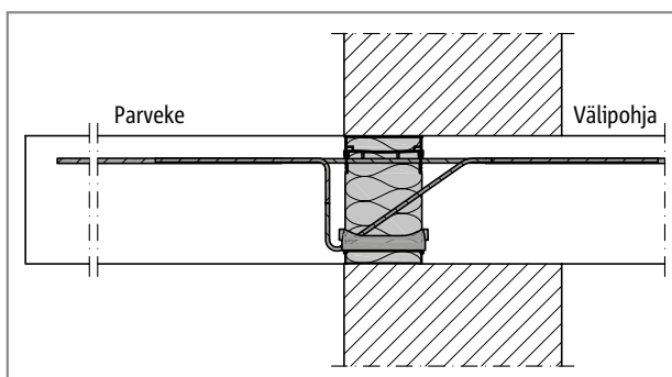
Schöck Isokorb® KXT: Tiiliverhottu ulkoseinä ja ulokeparveke
