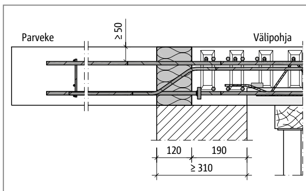
Schöck Isokorb® EXT, parvekelaatta, jossa reunatuki, lämpöeristävällä ulkoseinällä (leikkaus EXT-R-CV50, näkymä EXT-L-CV35)
