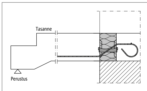
Schöck Isokorb® QXT: Yhtenäinen muurattu seinärakenne portaikon lepotsolla, kuvassa QXT10 - QXT40
