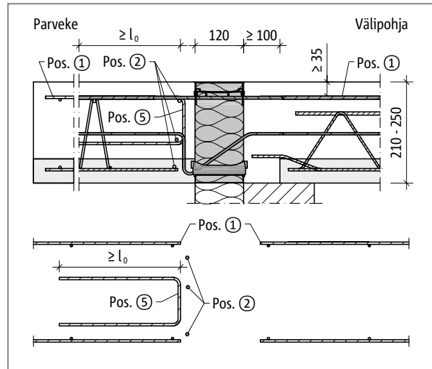
Schöck Isokorb® KTXT, parvekelaatan paksuus h = 210 - 250 mm
