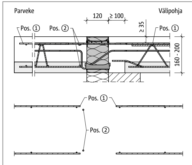
Schöck Isokorb® KTXT, parvekelaatan paksuus h = 160 - 200 mm
