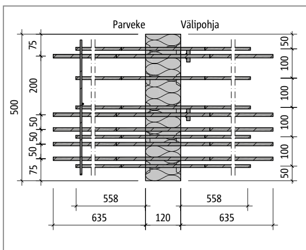
Schöck Isokorb® EXT30-R: Tasokuva
