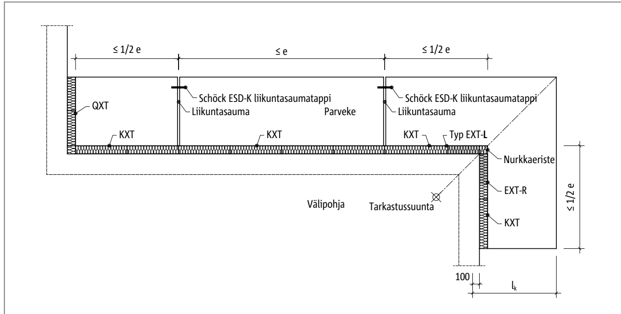
Schöck Isokorb® EXT: Liikuntasauman valmistus pituussuunnassa työnnettävän liikuntasaumatapin avulla, esim. Schöck ESD-K-liikuntasaumatappi
