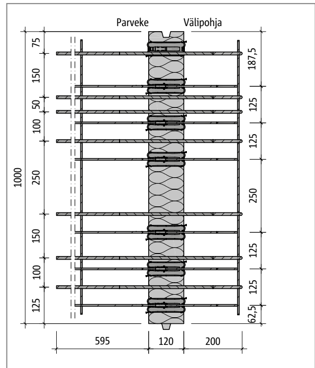
Schöck Isokorb® KXT30-WU: Tasokuva
