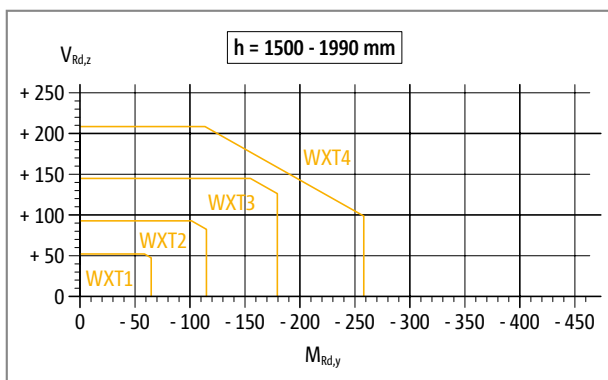
Schöck Isokorb® WXT: Interaktiogrammi C25/30 H = 1500 - 1990
