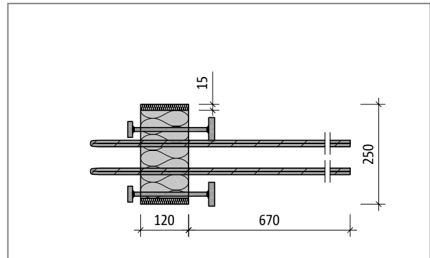
Schöck Isokorb® OXT R90: Tasokuva, palosuojauslevyt sivuilla
