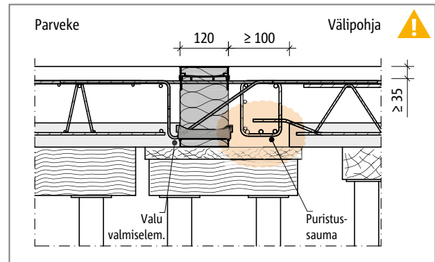
Schöck Isokorb® KXT: Epäsuora asennus, asennus Hollow Core -ontelolaattojen kanssa, puristussaumot välipohjan puolella
