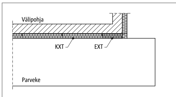
Schöck Isokorb® KXT: Ulkonurkkaparveke sivu-ulokkeella tyyppi EXT kanssa siirtämään suuria pistekuormia (katso s. 81)
