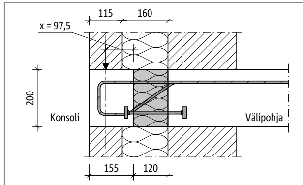
Schöck Isokorb® OXT: Seinäasennuksen mitoitusmerkki
