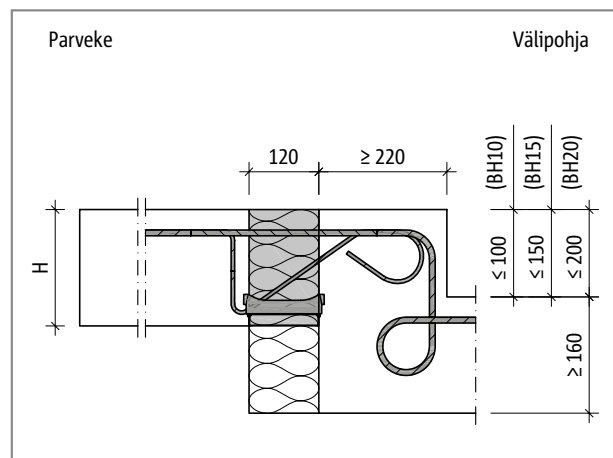
Schöck Isokorb® KXT-BH: Ylösnostettu parveke ja ulkoeriste
