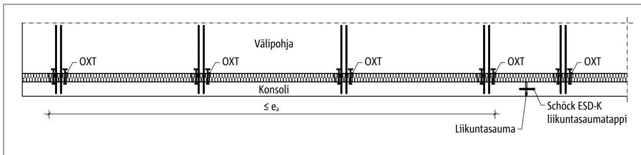
Schöck Isokorb® OXT: Liikuntasauman kohta pituussuunnassa liikuvan liikuntasaumatapin avulla, esim. Schöck ESD-K-liikuntasaumatappi
