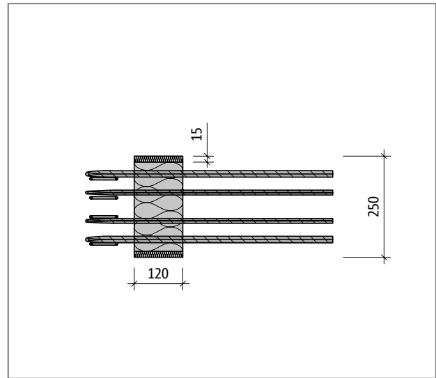
Schöck Isokorb® FXT, R90: Tasokuva, palosuojauslevyt sivuilla
