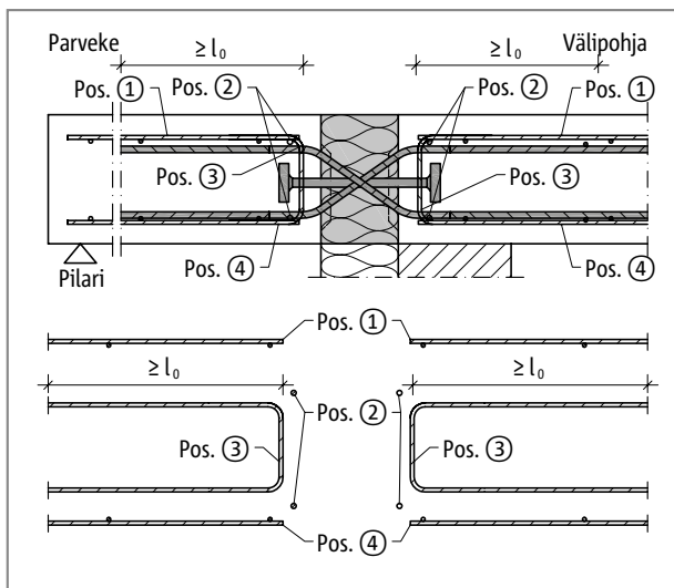
Schöck Isokorb® QPXT10+QPXT10 - QPXT70+QPXT70
