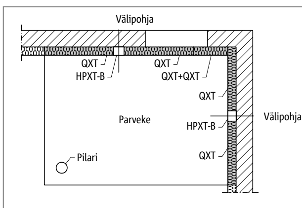
Schöck Isokorb® HPXT: Tuettu nurkkaparveke, pilari
