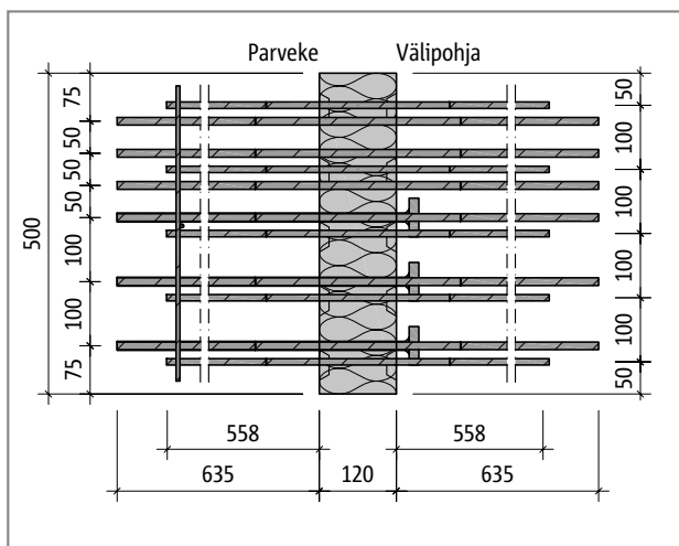
Schöck Isokorb® EXT50-L: Tasokuva
