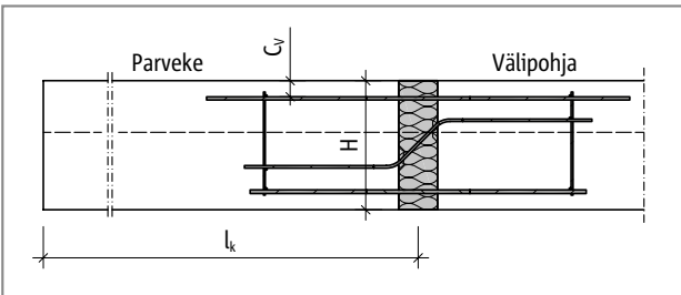
Schöck Isokorb® SXT: Mittausarvot määräytyvät esitetyn ulokemitan l_k mukaan suorassa tai epäsuorassa asennuksessa
