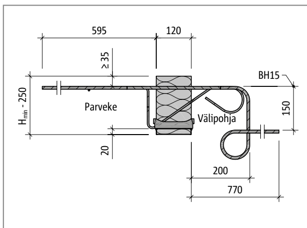
Schöck Isokorb® KXT30-BH15: Leikkaus
