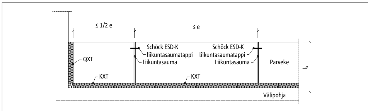
Schöck Isokorb® KXT: Liikuntasauman valmistus pituussuunnassa työnnettävän liikuntasaumatapin avulla, esim. Schöck ESD-K liikuntasaumatappi
