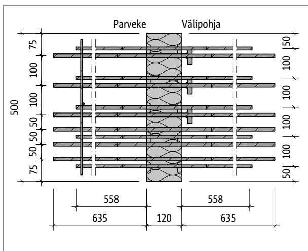
Schöck Isokorb® EXT50-R: Tasokuva
