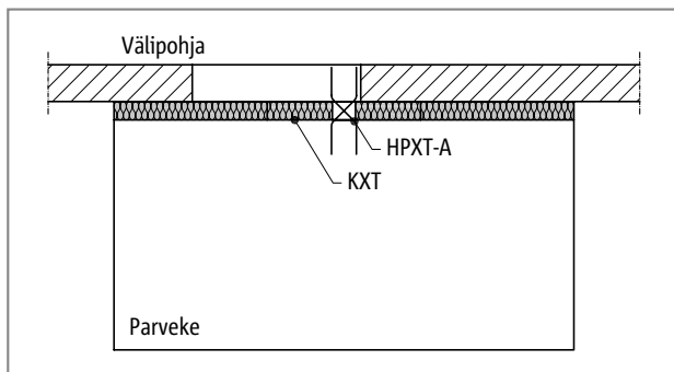
Schöck Isokorb® KXT: Vapaa ulokeparveke, vaihtoehtoisesti tyyppi HPXT kanssa (alk. sivulta 157) vaakasuuntaisia kuormituksia varten, esim. suljetut kaiteet
