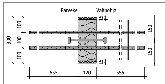
Schöck Isokorb® QPXT10+QPXT10, REI90: Tasokuva
