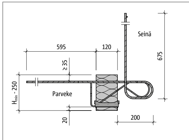
Schöck Isokorb® KXT30-WO: Leikkaus
