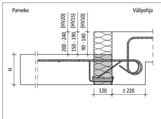
Schöck Isokorb® KXT-HV: Alaslaskettu parveke ja ulkoeriste
