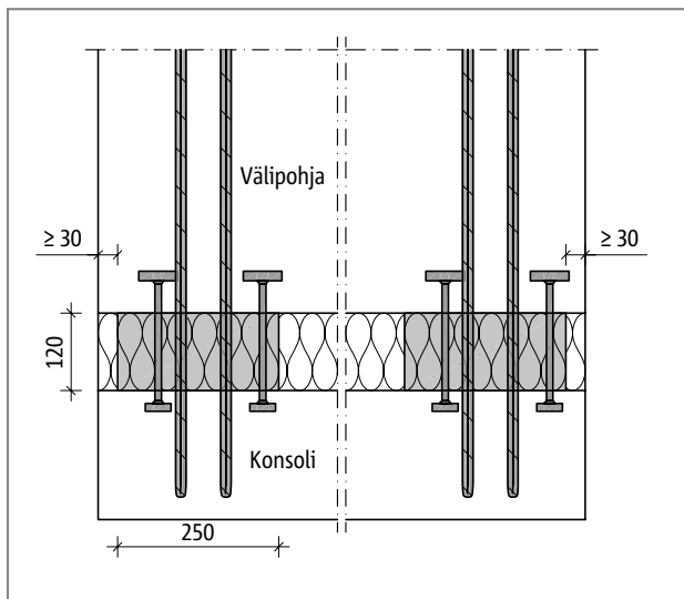
Schöck Isokorb® OXT: Noudatettava reunaetäisyys
