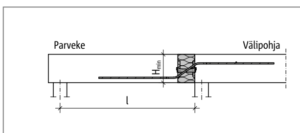
Schöck Isokorb® QXT60 - QXT90: Staattinen järjestelmä
