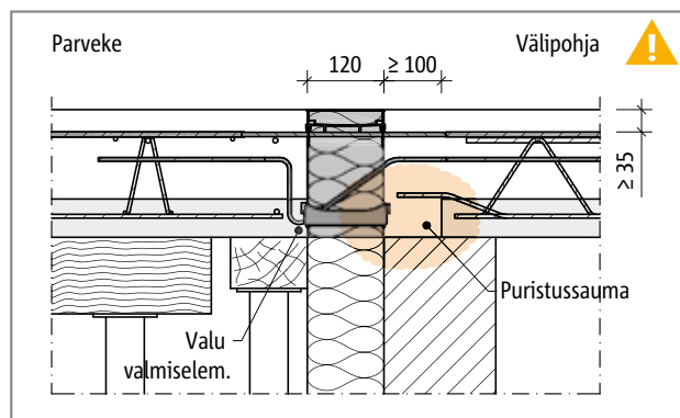
Schöck Isokorb® KFXT: Asennus elementtilaattojen (tässä: h \leq 200 mm) kanssa, suora asennus, puristussauma välipohjan puolella
