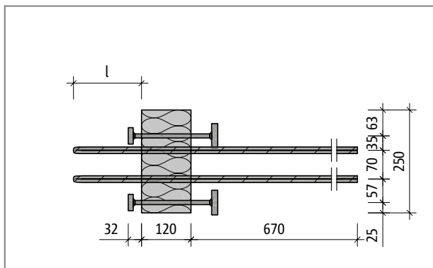
Schöck Isokorb® OXT: Tasokuva
