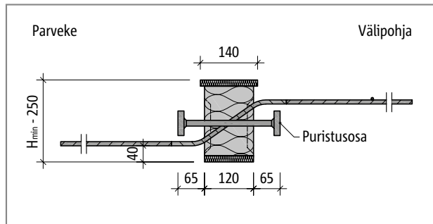
Schöck Isokorb® QPXT10 - QPXT100, REI90: Leikkaus
