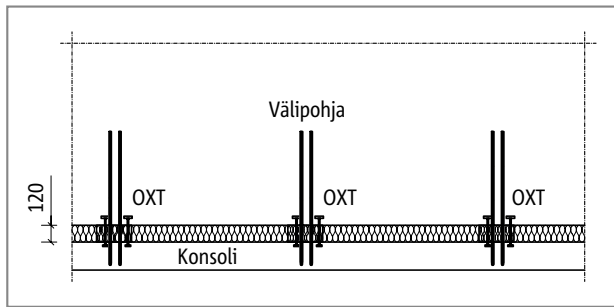
Schöck Isokorb® OXT: Konsoli
