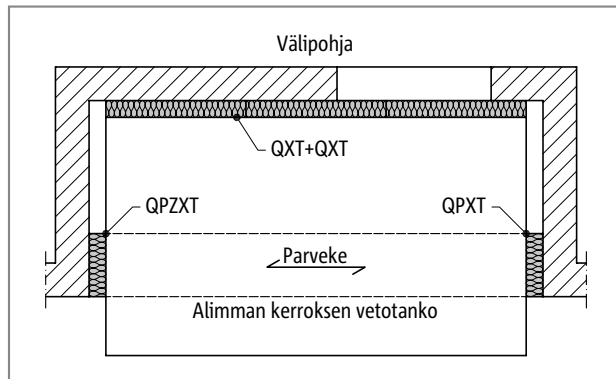
Schöck Isokorb® QXT+QXT, QPXT ja QPZXT: Sisäänvedetty parveke, tuettu kolmelta sivulta
