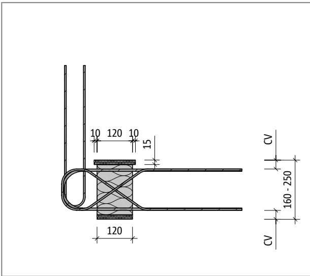
Schöck Isokorb® FXT, R90: Leikkaus, palosuojauslevyt ylhäällä ja alhaalla
