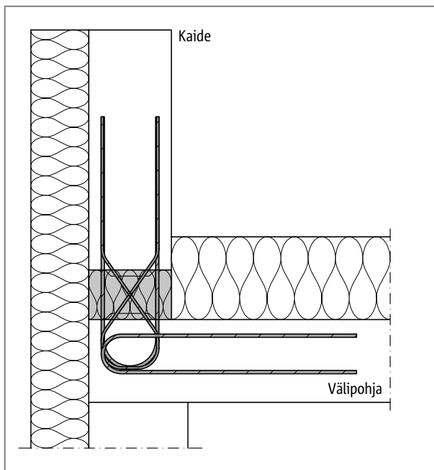
Schöck Isokorb® AXT2: Kaiteen liitos
