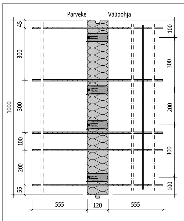
Schöck Isokorb® QXT70: Tasokuva
