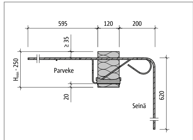
Schöck Isokorb® KXT30-WU: Leikkaus
