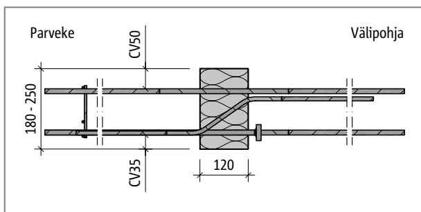
Schöck Isokorb® EXT-L-CV50: Leikkaus
