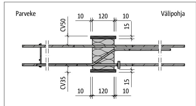
Schöck Isokorb® EXT30-CV50, REI90: Leikkaus
