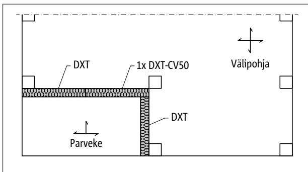
Schöck Isokorb® DXT: Käyttö välipohjiissa
