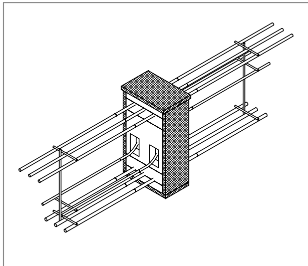
Schöck Isokorb® SXT1, R90: Palosuojalevyt ympäriinsä
