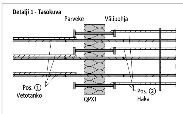
Schöck Isokorb® QPXT: Detalji 1 Tasokuva - vetotangon rauditusliitos
