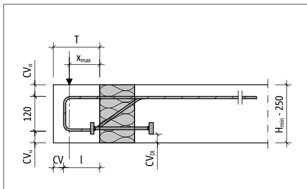
Schöck Isokorb® OXT: Leikkaus
