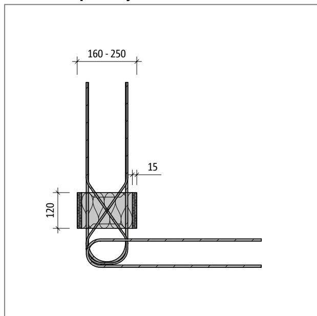
Schöck Isokorb® AXT2, R90: Leikkaus, palosuojalevyt sivuilla
