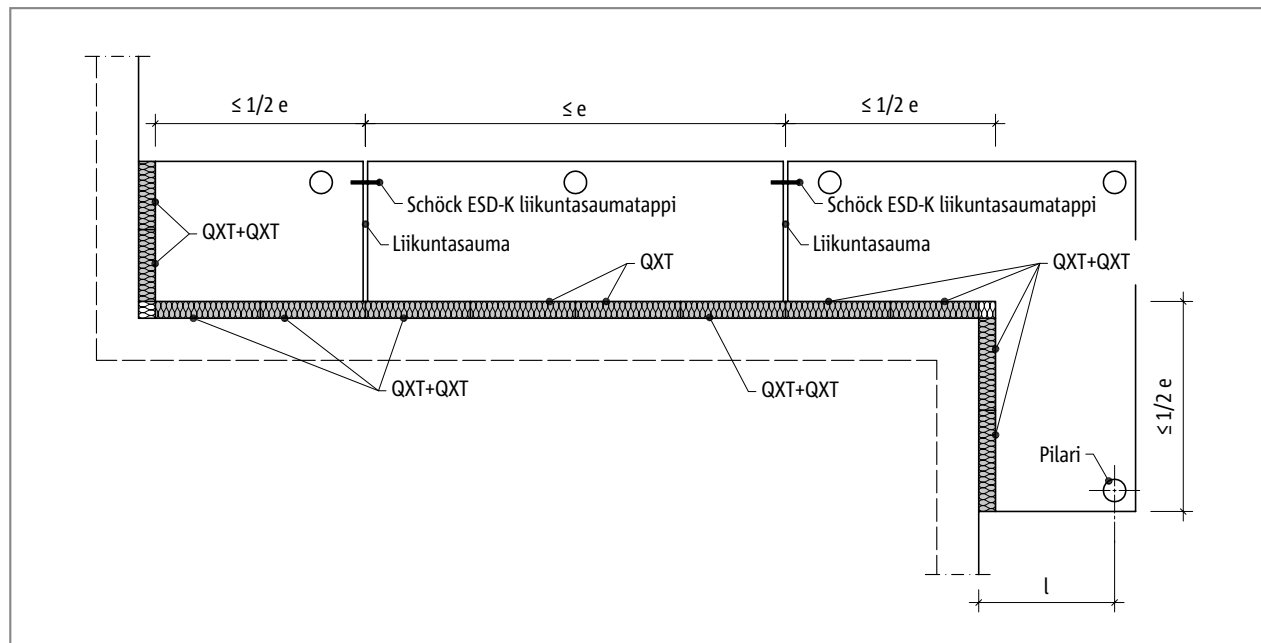
Schöck Isokorb® QXT ja QXT+QXT: Liikuntasauman toteutus pituussuunnassa työnnettävän liikuntasaumatapin avulla, esim. Schöck ESD-K liikuntasaumatappi
