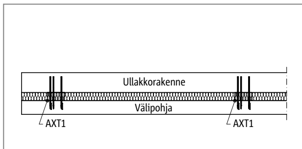
Schöck Isokorb® AXT1: Ullakkorakenne
