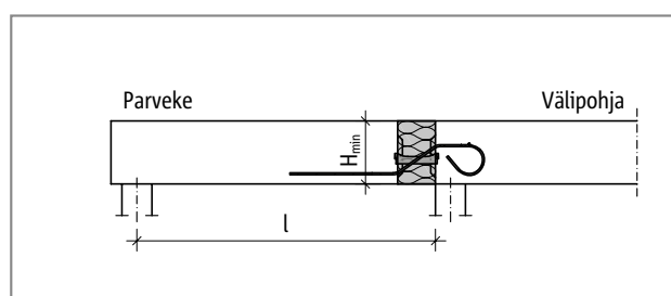
Schöck Isokorb® QXT10 - QXT40: Staattinen järjestelmä
