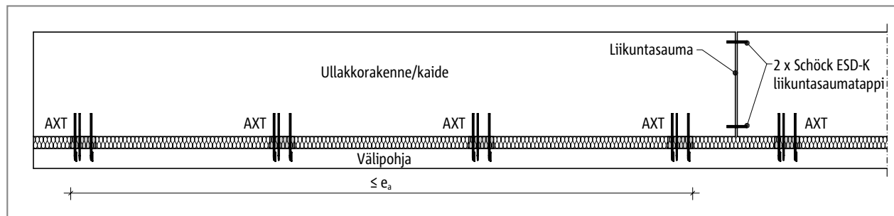
Schöck Isokorb® AXT: Liikuntasauman toteutus pituussuunnassa työnnettävän liikuntasaumatapin avulla, esim. Schöck ESD-K-liikuntasaumatappi
