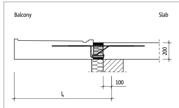
Fig. 57: Schöck Isokorb® XT type K: Static system
