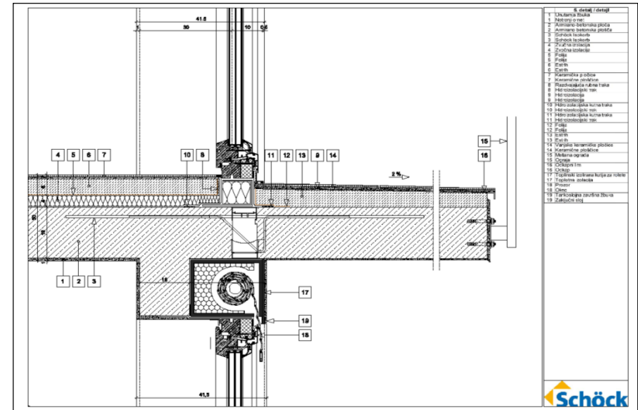
Detalj balkona sa Isokorb elementom.
