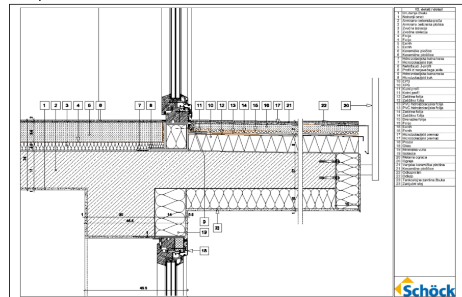
Detalj balkona bez Isokorb elementa.
