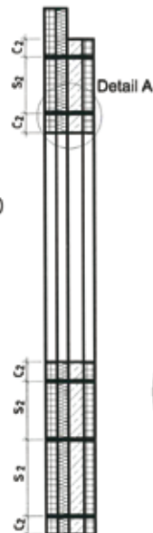
Schnitt B-B Elementwand:
