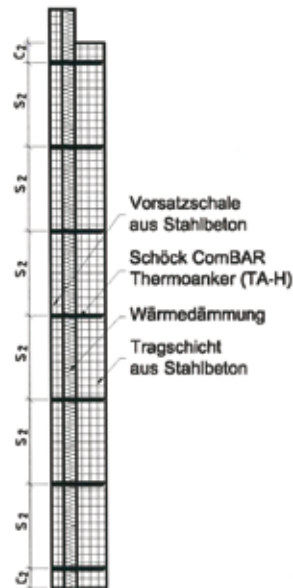
Schnitt A-A Sandwichwand:
