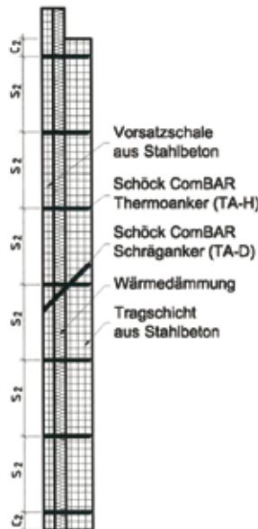
Schnitt A-A Sandwichwand:
