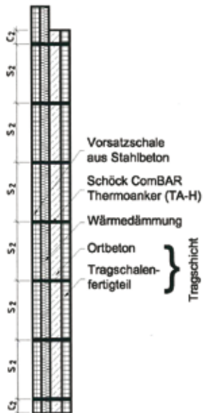
Schnitt A-A Elementwand:
