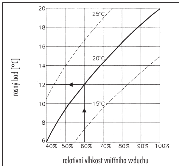
Graf 2: Závislost teploty rosného bodu na relativní vlhkosti vnitřního vzduchu za různých teplot vnitřního vzduchu. Z grafu je patrné, že při běžné teplotě a relativní vlhkosti vnitřního vzduchu (teplota 20°C, relativní vlhkost < 60 %) dochází již při povrchové teplotě 12°C ke kondenzaci vodní páry na povrchu stavební konstrukce (šipka).
