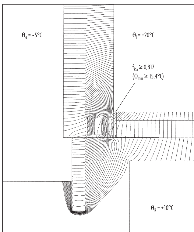
Izočáry tepelného toku, teplotní činitel vnitřního povrchu a nejnižší vnitřní povrchová teplota u kontaktního zateplovacího systému
