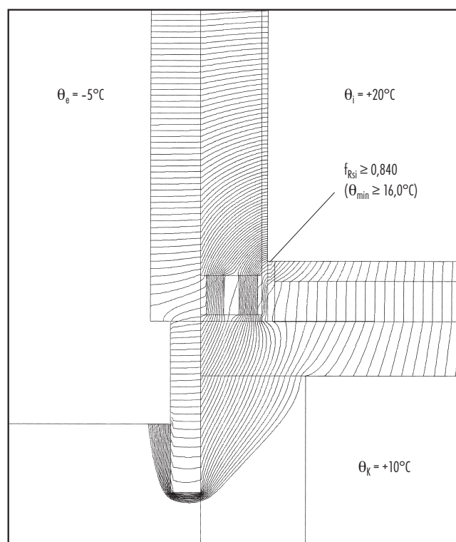
Izočáry tepelného toku, teplotní činitel vnitřního povrchu a nejnižší vnitřní povrchová teplota u kontaktního zateplovacího systému
