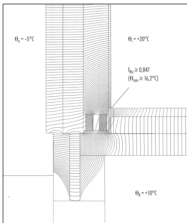
Izočáry tepelného toku, teplotní činitel vnitřního povrchu a nejnižší vnitřní povrchová teplota u sendvičové obvodové stěny
