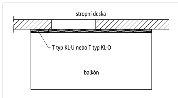
Obr. 68: Schöck Isokorb® T typ KL-U/KL-O: Volně vyložený balkón
