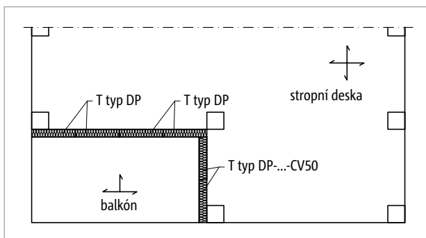
Obr. 190: Schöck Isokorb® T typ DP: Užití v bezprůvlakových stropních deskách
