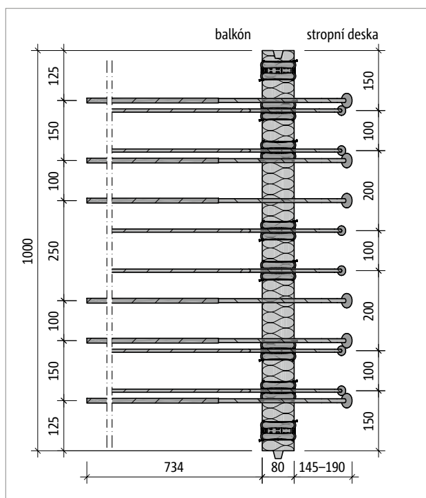
Obr. 90: Schöck Isokorb® T typ KL-O-M2: Půdorys prvku
