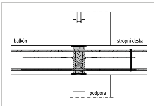
Obr. 192: Schöck Isokorb® T typ DP: Řez, bezprůvlaková stropní deska
