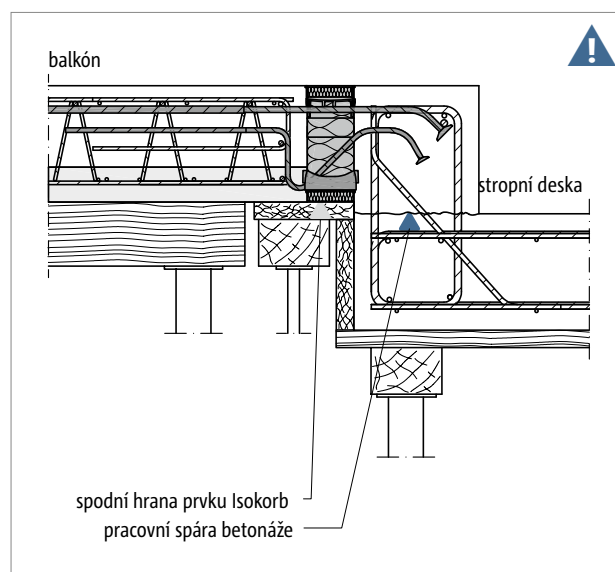
Obr. 113: Schöck Isokorb® T typ KL-O-F: Poloprefabrikovaný balkón nadvýšeň oproti stropní desce
