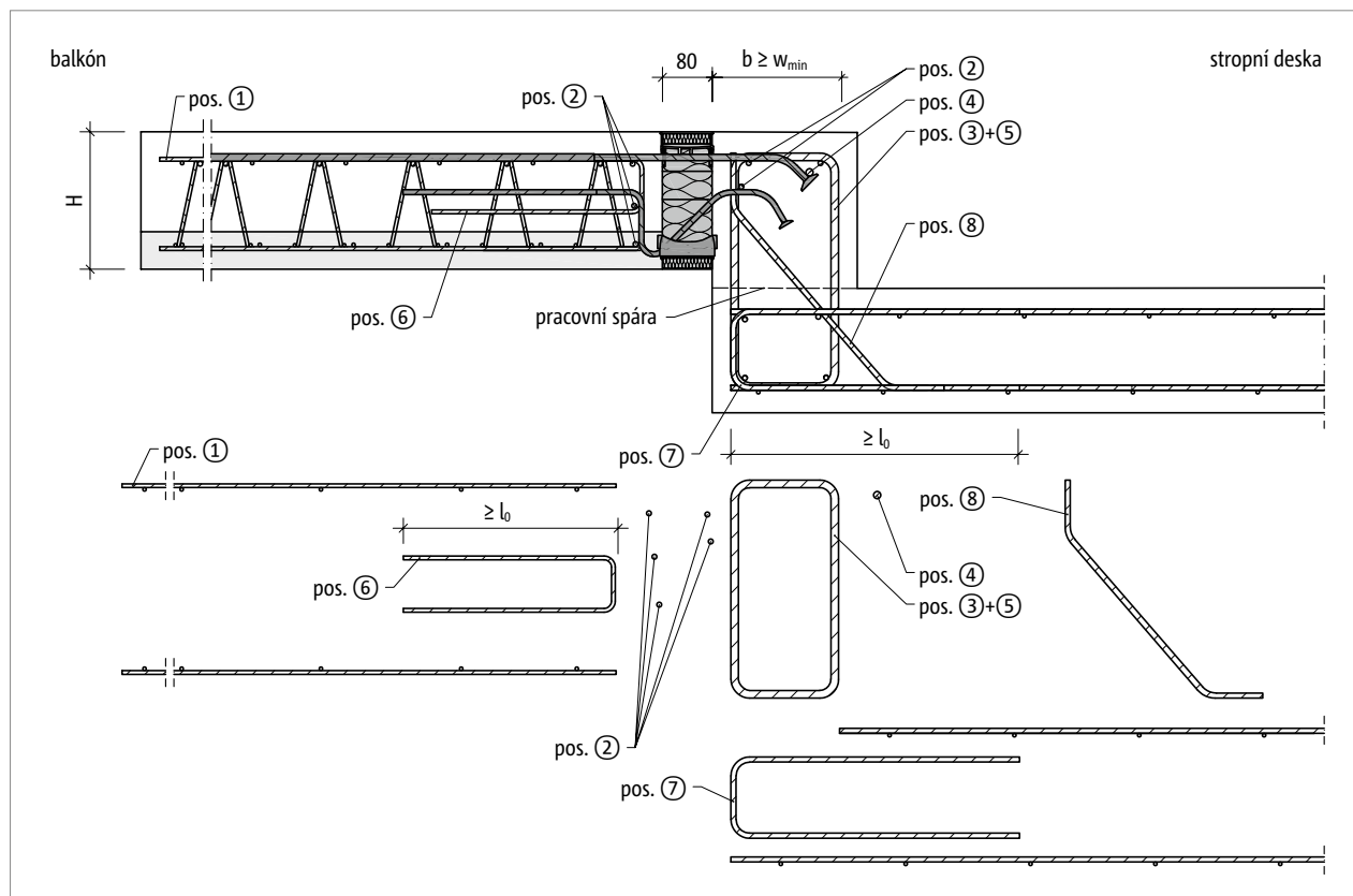
Obr. 108: Schöck Isokorb® T typ KL-O-F: Napojovací stavební výztuž pro balkón nadvýšený oproti stropní desce
