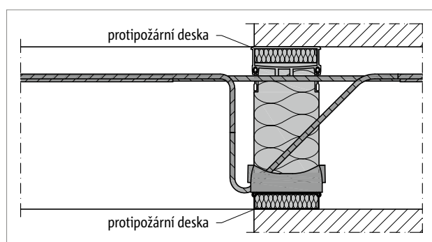
Obr. 40: Schöck Isokorb® T typ KL v provedení REI120: detail 1
