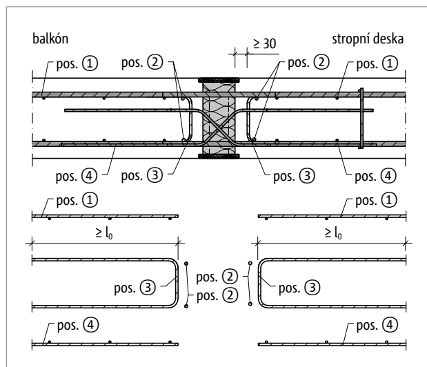
Obr. 200: Schöck Isokorb® T typ DP: Napojovací stavební výztuž
