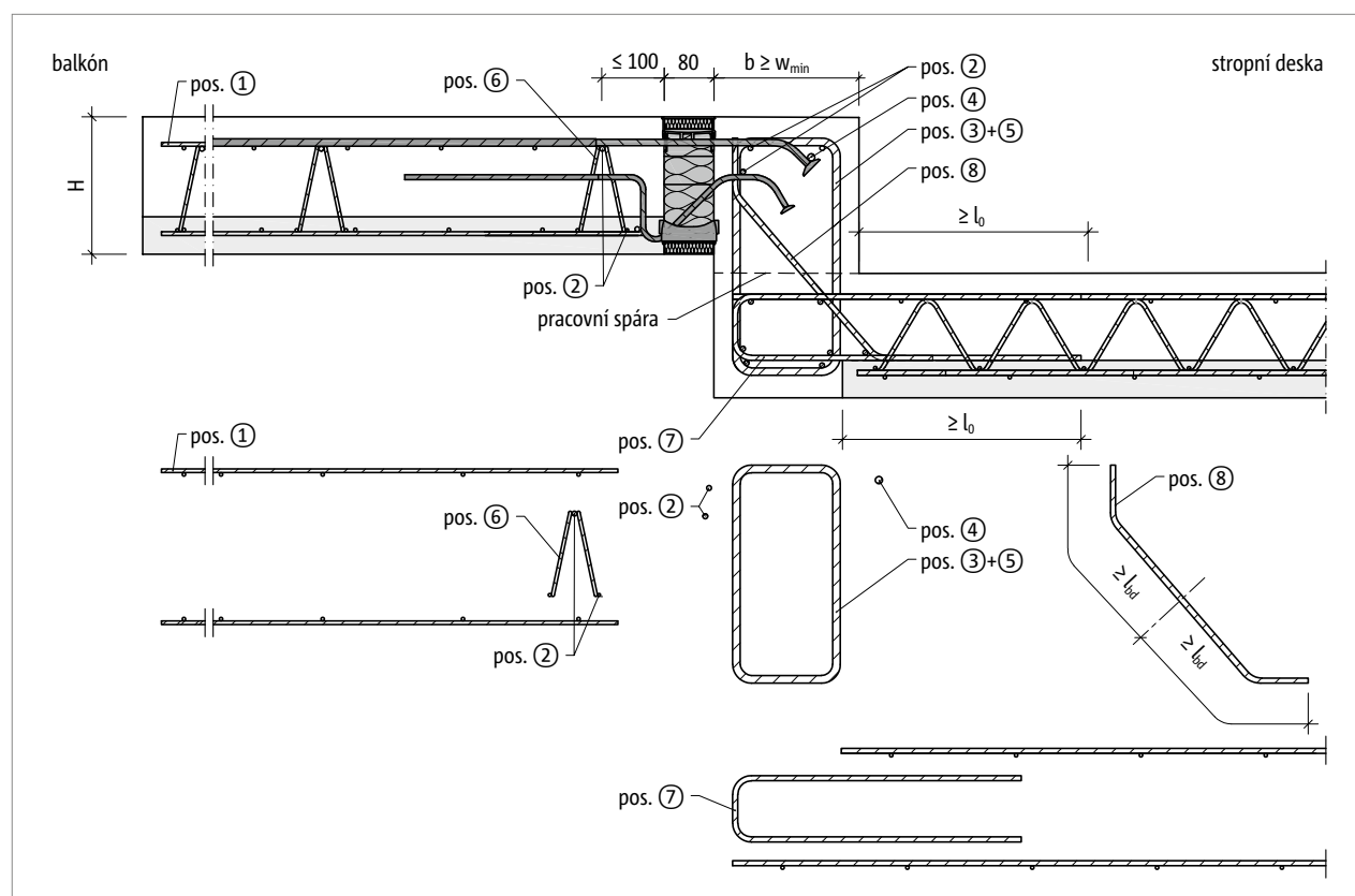
Obr. 111: Schöck Isokorb® T typ KL-O-F: Napojovací stavební výztuž pro balkón nadvýšený oproti stropní desce
