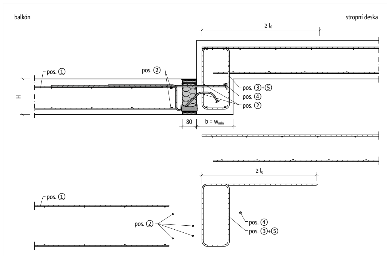
Obr. 92: Schöck Isokorb® T typ KL-U: Napojovací stavební výztuž pro balkón snížený oproti stropní desce – s minimálním rozměrem ( w_{skut} = w_{min} )
