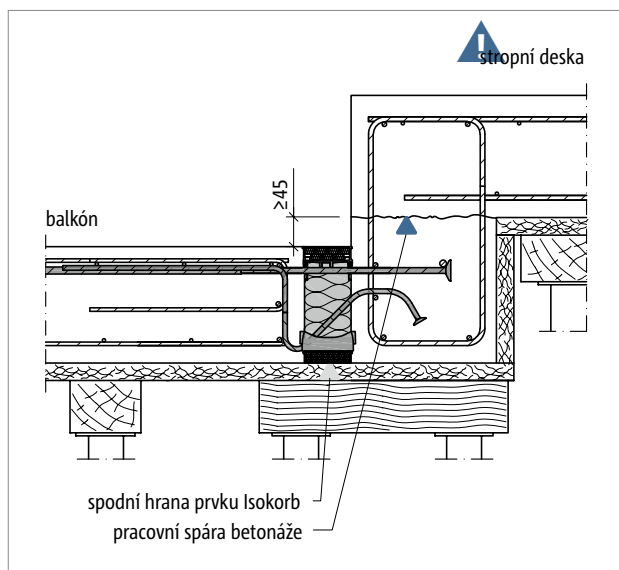
Obr. 100: Schöck Isokorb® T typ KL-U: Monolitický balkón snížený oproti stropní desce
