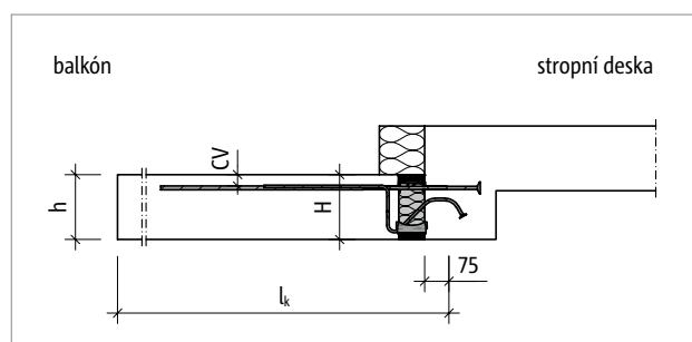
Obr. 78: Schöck Isokorb® T typ KL-U: Statický systém
