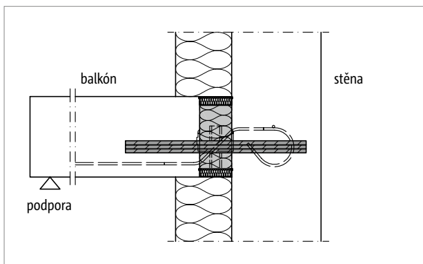
Obr. 176: Schöck Isokorb® T typ QL, HP-VV-NN: Napojení na železobetonovou stěnu s vnějším zateplením
