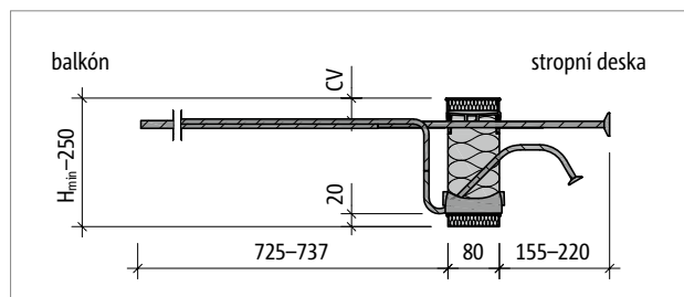
Obr. 84: Schöck Isokorb® T typ KL-U-M2: Řez prvkem
