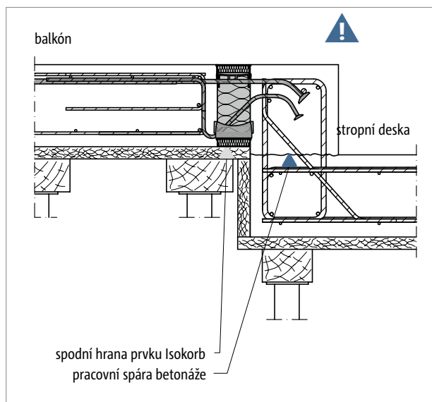
Obr. 101: Schöck Isokorb® T typ KL-O: Monolitický balkón nadvýšený oproti stropní desce
