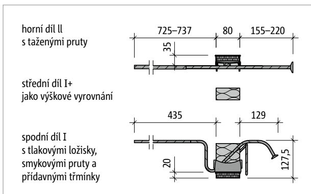
Obr. 103: Schöck Isokorb® T typ KL-U-F-M3-V1-CV1 až KL-U-F-M4-V1-CV1
