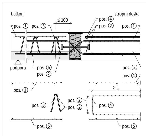
Obr. 158: Schöck Isokorb® T typ QP: Napojovací stavební výztuž, na straně balkónu s filigránovou výztuží
