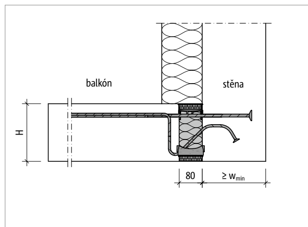
Obr. 76: Schöck Isokorb® T typ KL-U: Kotvení do paty stěny u vnějšího zateplení
