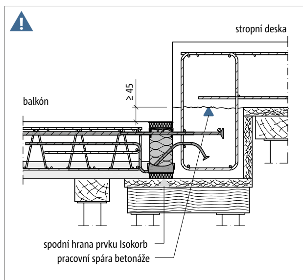
Obr. 112: Schöck Isokorb® T typ KL-U-F: Poloprefabrikovaný balkón snížený oproti stropní desce
