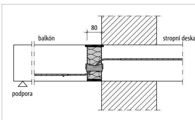
Obr. 41: Schöck Isokorb® T typ QL v provedení REI120: Protipožární desky na horní i spodní straně
