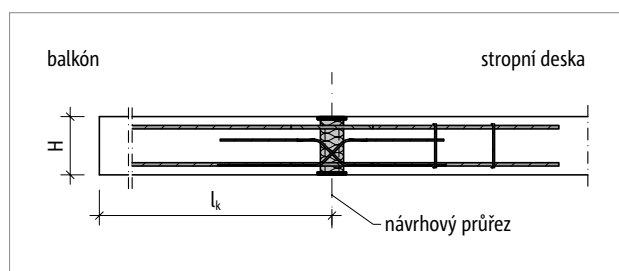
Obr. 194: Schöck Isokorb® T typ DP: Statický systém
