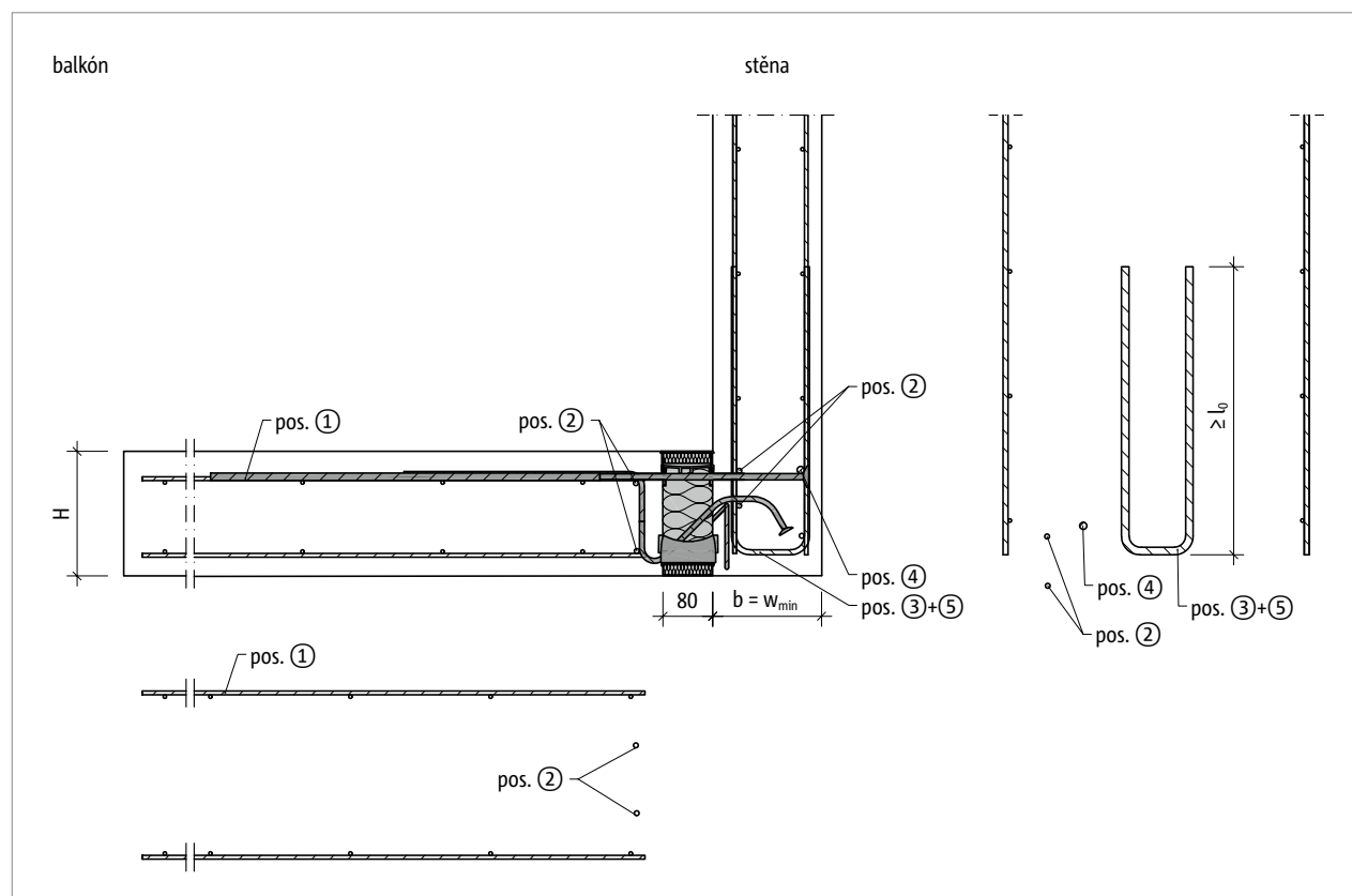
Obr. 94: Schöck Isokorb® T typ KL-U: Napojovací stavební výztuž pro desku kotvenou do paty stěny s minimálním rozměrem ( w_{skut} = w_{min} )
