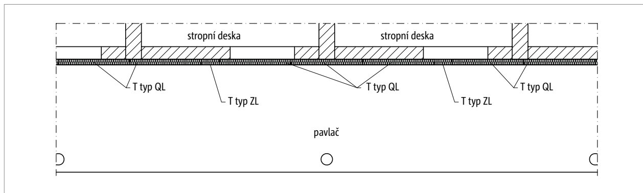
Obr. 42: Schöck Isokorb® T typ QL-REI120, T typ ZL-EI120: Pavlač s požadavkem na celistvost
