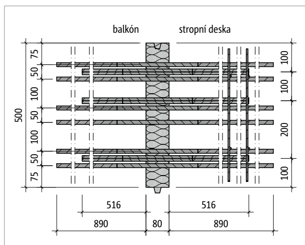
Obr. 199: Schöck Isokorb® T typ DP-MM6-VV3: Půdorys
