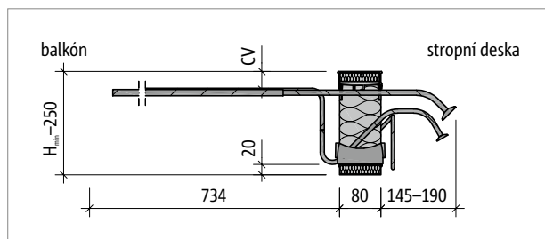
Obr. 89: Schöck Isokorb® T typ KL-O-M4: Řez prvkem
