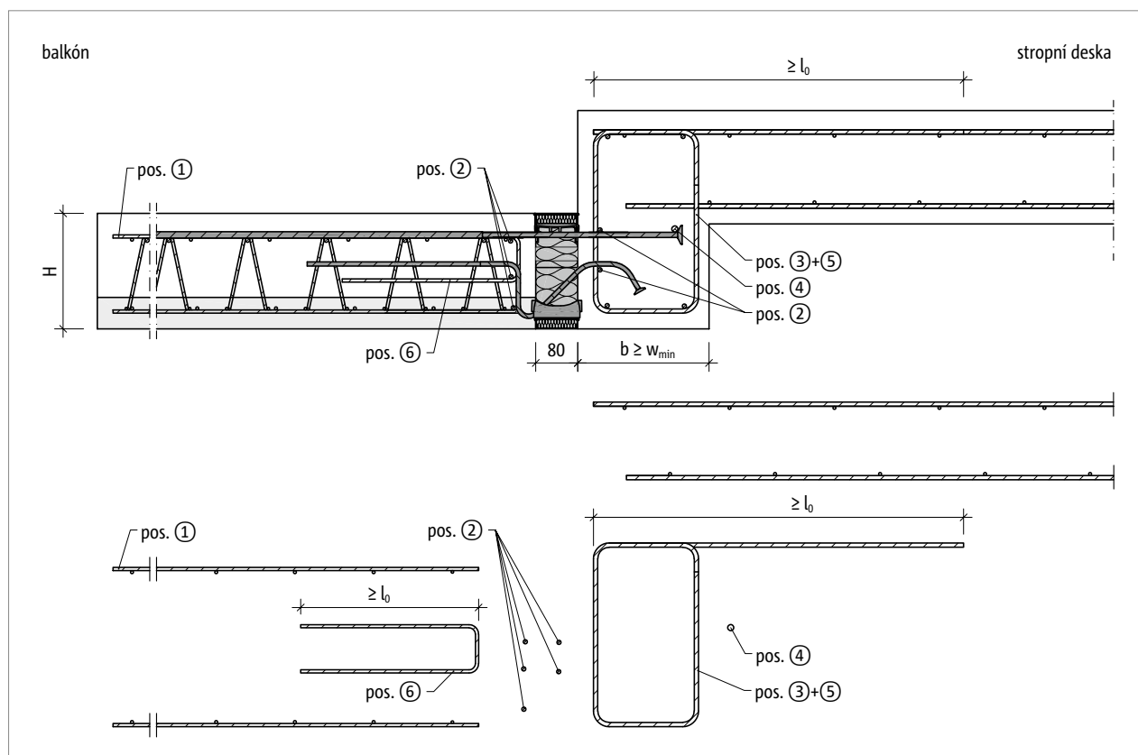
Obr. 106: Schöck Isokorb® T typ KL-U-F: Napojovací stavební výztuž pro balkón snížený oproti stropní desce
