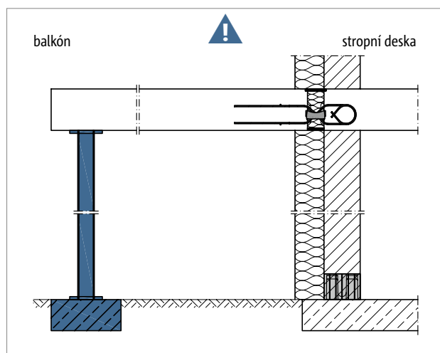
Obr. 167: Schöck Isokorb® T typ QL-VV: Podepření je nutno zajistit i během provádění
