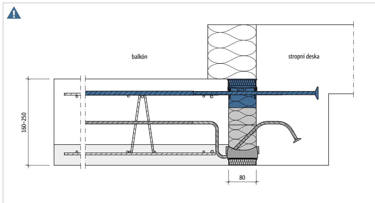
Obr. 114: Schöck Isokorb® T typ KL-U-F: Prvek složený z několika částí – horního dílu, středního dílu (k případnému výškovému vyrovnání) a spodního dílu. Zde: horní díl je barevně označen.
