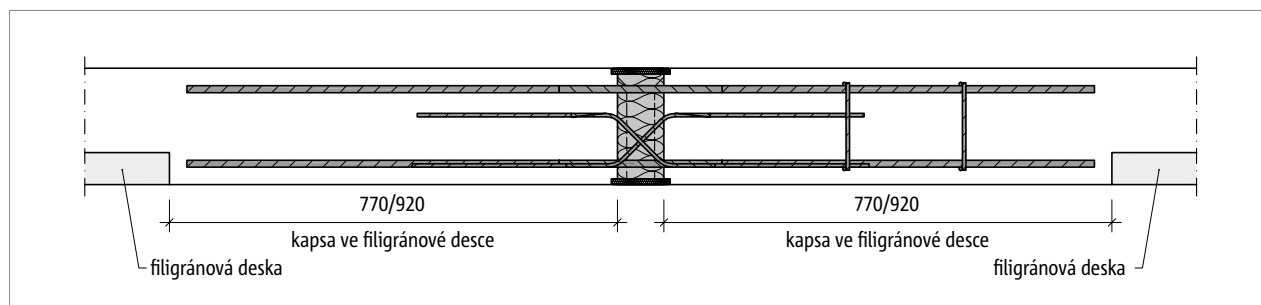
Obr. 202: Schöck Isokorb® T typ DP: Filigránová deska s kapsami pro zabudování prvku Isokorb® T typ DP v úrovni spodní hrany desky
