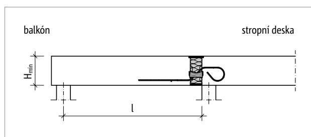
Obr. 129: Schöck Isokorb® T typ QL-V1: Statický systém
