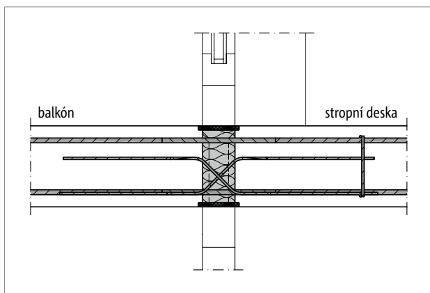
Obr. 191: Schöck Isokorb® T typ DP: Řez, deska vyztužená v jednom směru
