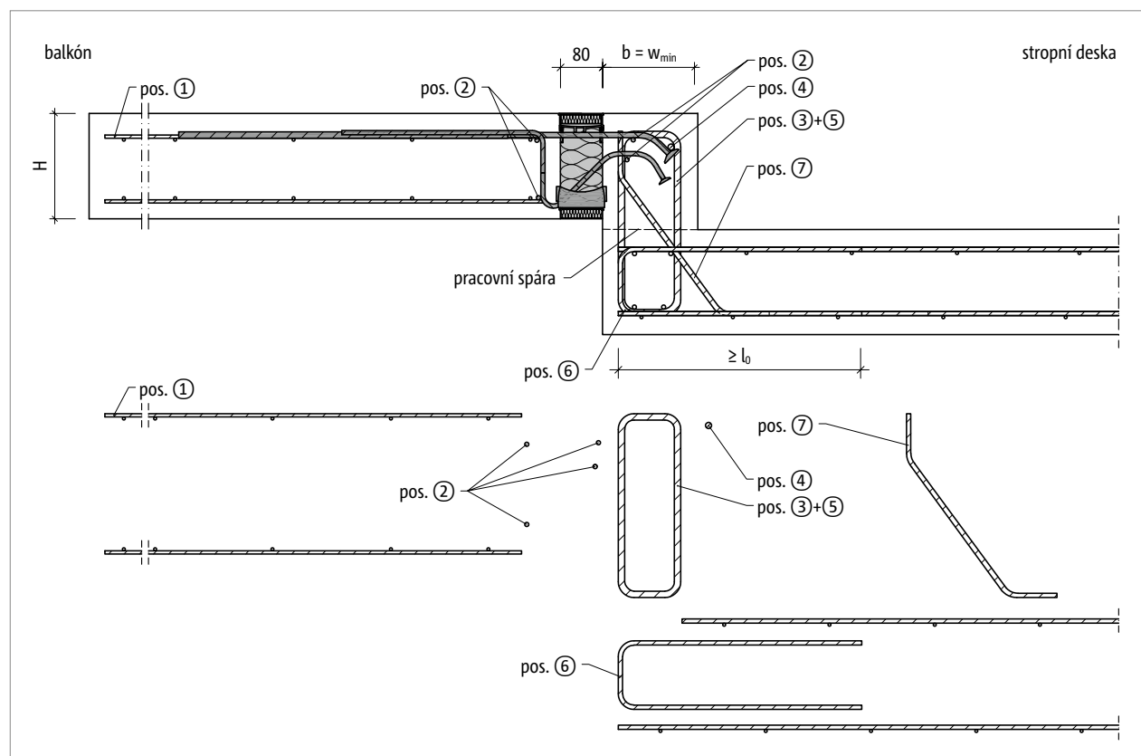
Obr. 96: Schöck Isokorb® T typ KL-O: Napojovací stavební výztuž pro balkón nadvýšený oproti stropní desce – s minimálním rozměrem ( w_{skut} = w_{min} )
