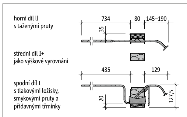
Obr. 105: Schöck Isokorb® T typ KL-O-F-M4-V1-CV1
