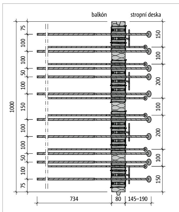
Obr. 91: Schöck Isokorb® T typ KL-O-M4: Půdorys prvku
