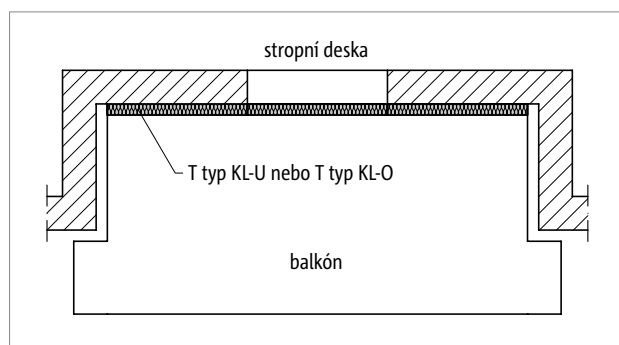
Obr. 70: Schöck Isokorb® T typ KL-U/KL-O: Balkón na zalomené fasádě
