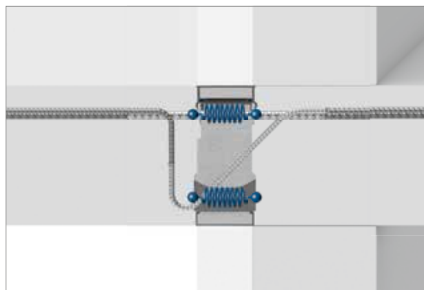
Obr. 12: Schöck Isokorb®: Tažený prut a tlačené ložisko působí jako pružina
