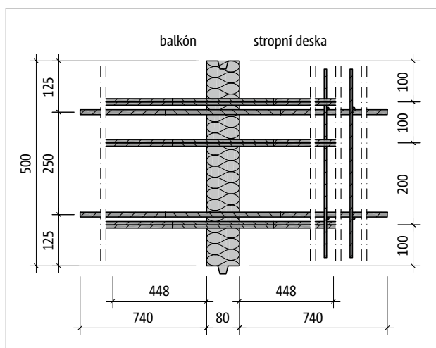
Obr. 198: Schöck Isokorb® T typ DP-MM1-VV3: Půdorys
