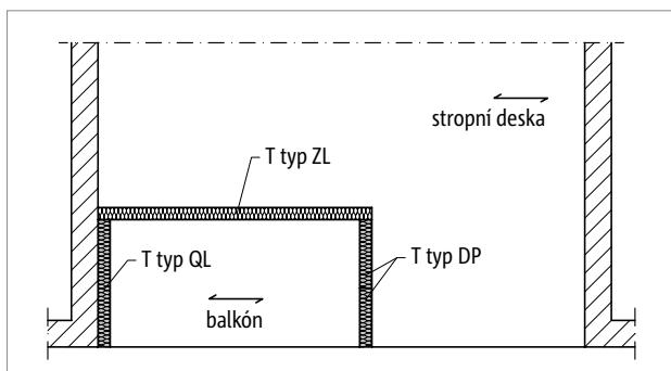
Obr. 189: Schöck Isokorb® T typ DP, QL-Z, ZL: Deska vyztužená v jednom směru
