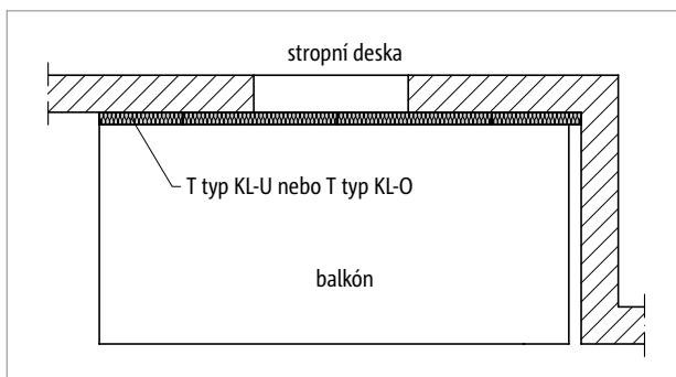
Obr. 69: Schöck Isokorb® T typ KL-U/KL-O: Balkón na zalomené fasádě
