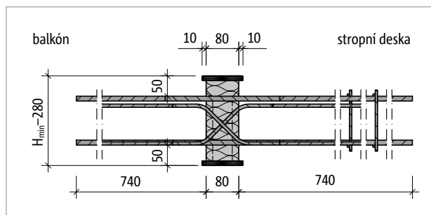
Obr. 197: Schöck Isokorb® T typ DP-MM1-VV3 u CV2: Řez prvkem
