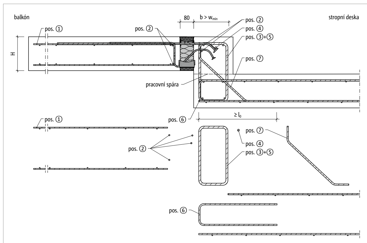
Obr. 97: Schöck Isokorb® T typ KL-O: Napojovací stavební výztuž pro balkón nadvýšený oproti stropní desce – s větším rozměrem ( w_{skut} > w_{min} )
