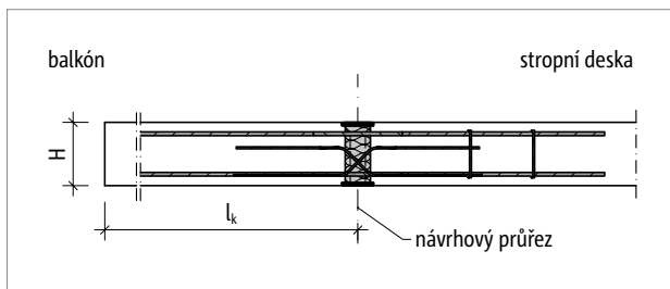
Obr. 193: Schöck Isokorb® T typ DP: Statický systém
