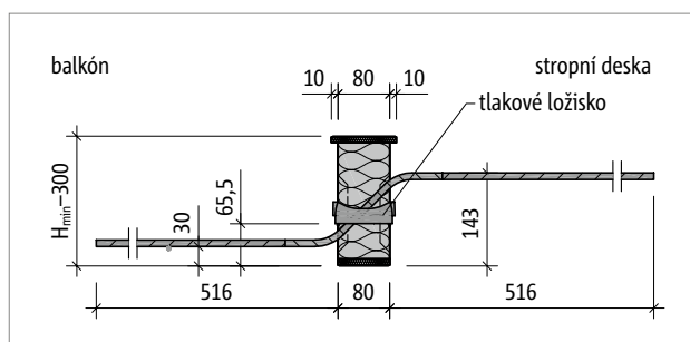
Obr. 138: Schöck Isokorb® T typ QL-V4: Řez prvkem
