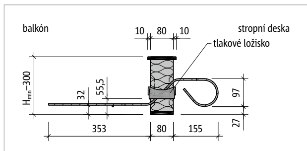
Obr. 136: Schöck Isokorb® T typ QL-V1: Řez prvkem
