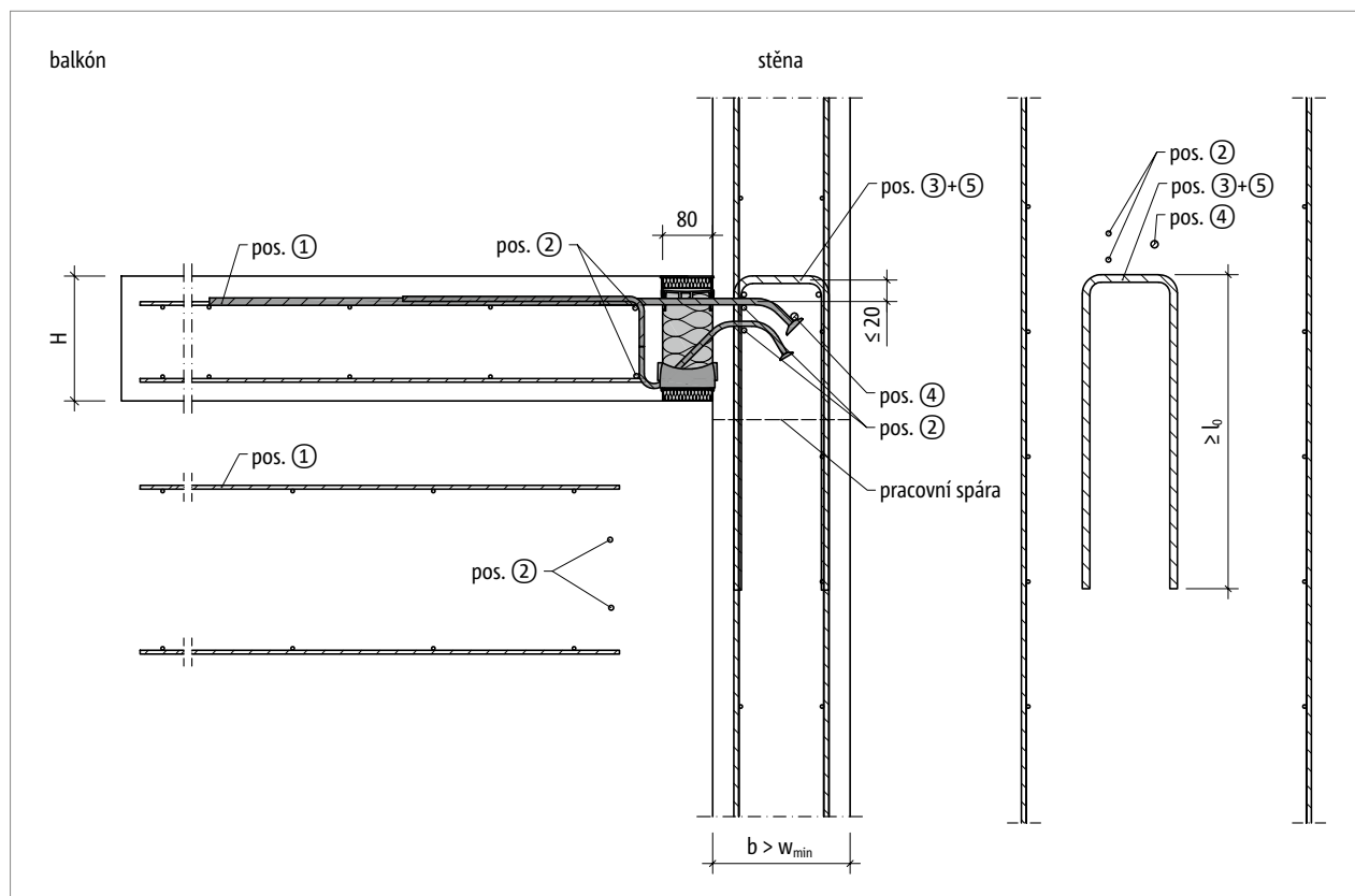
Obr. 99: Schöck Isokorb® T typ KL-O: Napojovací stavební výztuž pro desku kotvenou do stěny s větším rozměrem ( w_{skut} > w_{min} )
