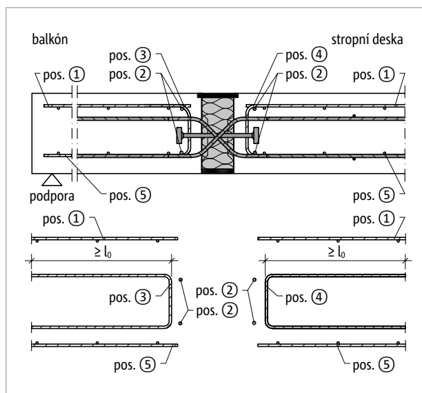
Obr. 156: Schöck Isokorb® T typ QP-VV: napojovací stavební výztuž
