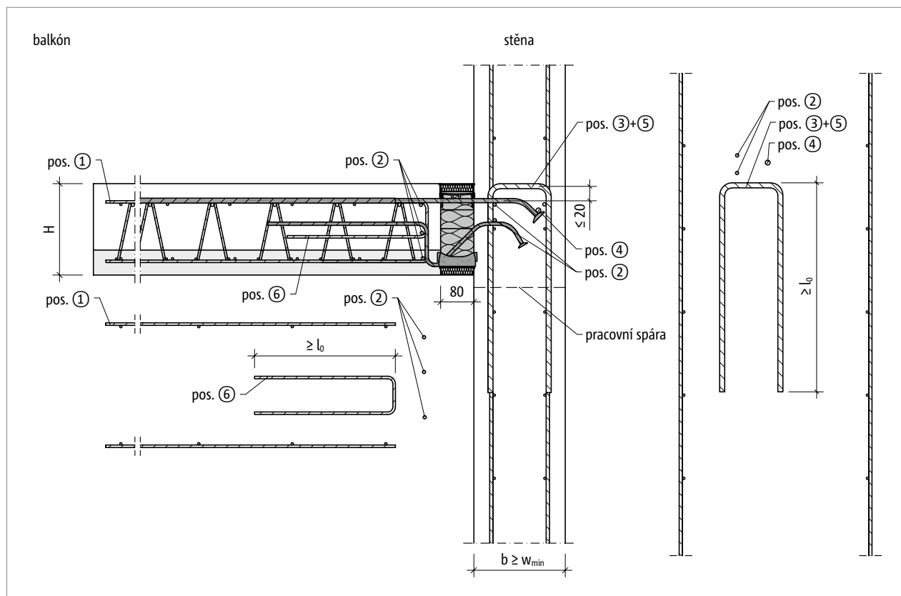
Obr. 109: Schöck Isokorb® T typ KL-O-F: Napojovací stavební výztuž pro desku kotvenou do stěny pod úrovní balkónu
