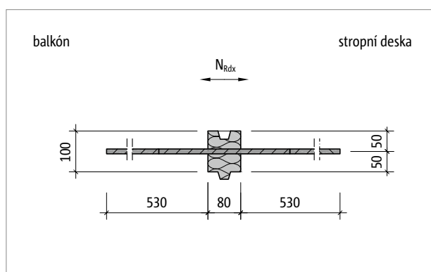
Obr. 182: Schöck Isokorb® T typ HP-NN2: Půdorys prvku
