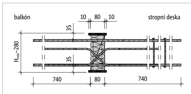
Obr. 196: Schöck Isokorb® T typ DP-MM1-VV3 u CV1: Řez prvkem
