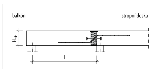
Obr. 133: Schöck Isokorb® T typ QP: Statický systém
