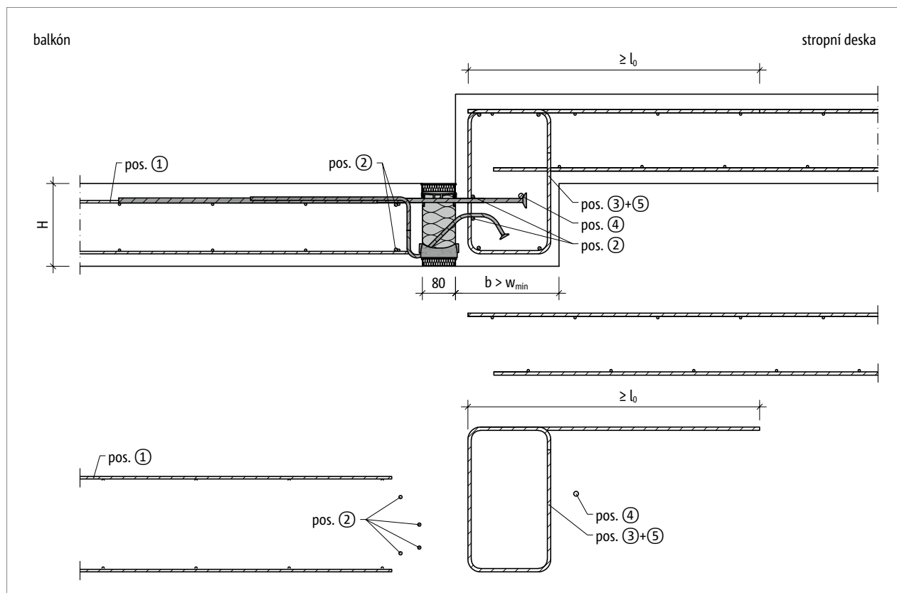
Obr. 93: Schöck Isokorb® T typ KL-U: Napojovací stavební výztuž pro balkón snížený oproti stropní desce – s větším rozměrem ( w_{skut} > w_{min} )
