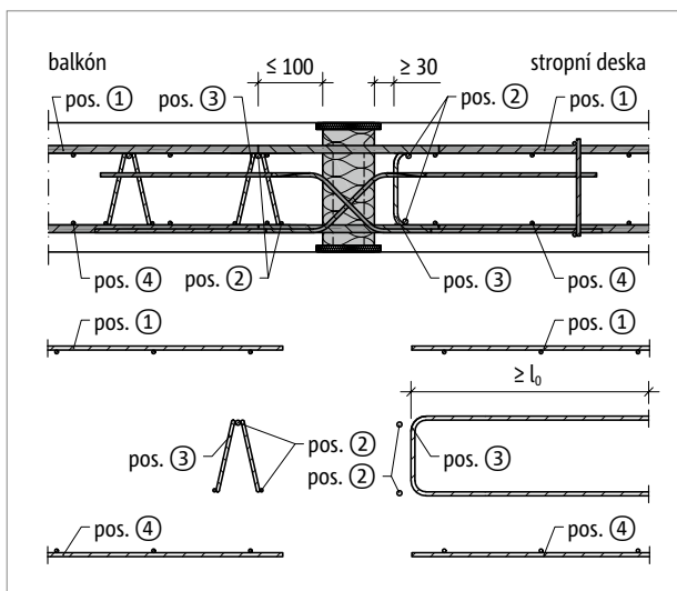
Obr. 201: Schöck Isokorb® T typ DP: Napojovací stavební výztuž s filigránovou výztuží
