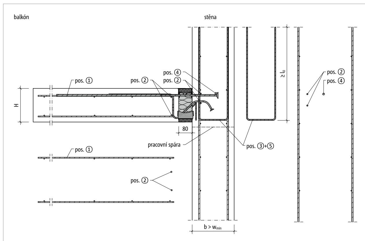
Obr. 95: Schöck Isokorb® T typ KL-U: Napojovací stavební výztuž pro desku kotvenou do stěny s větším rozměrem ( w_{skut} > w_{min} )
