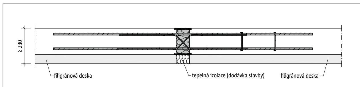
Obr. 203: Schöck Isokorb® T typ DP: Isokorb® T typ DP zabudovaný nad filigránovou deskou
