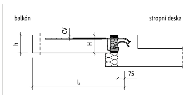
Obr. 79: Schöck Isokorb® T typ KL-O: Statický systém
