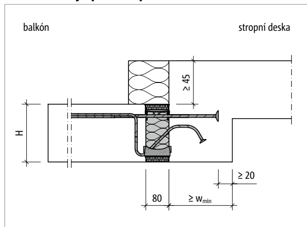
Obr. 72: Schöck Isokorb® T typ KL-U: Balkón snížený oproti stropní desce, vnější zateplení
