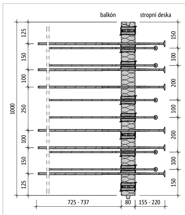
Obr. 86: Schöck Isokorb® T typ KL-U-M2: Půdorys prvku
