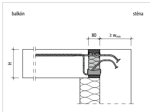
Obr. 77: Schöck Isokorb® T Typ KL-O: Kotvení do hlavy stěny u vnějšího zateplení
