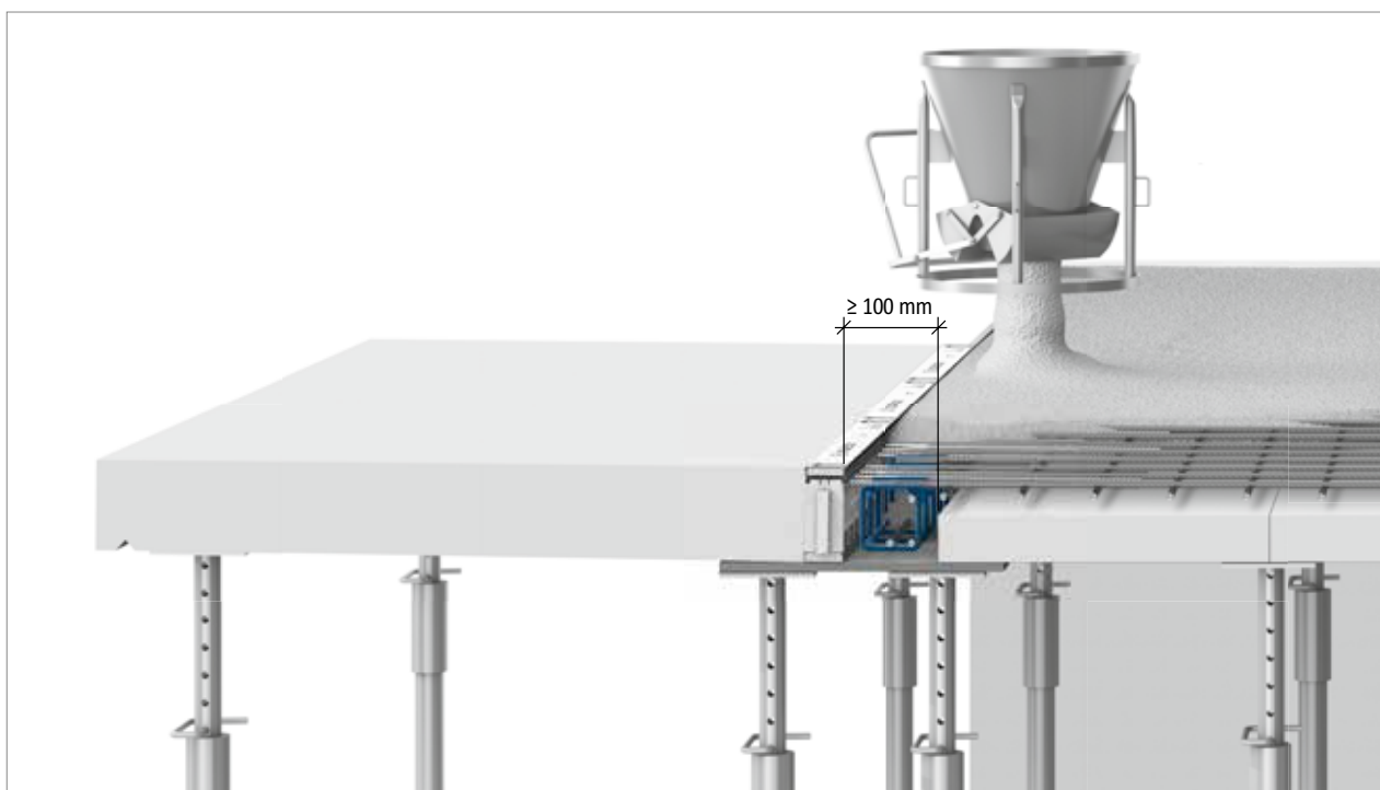
Obr. 37: Schöck Isokorb® T typ KL: Betonáž monolitického pásu (tlačená oblast)
