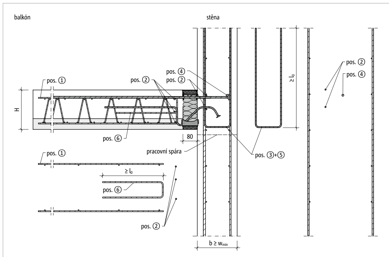
Obr. 107: Schöck Isokorb® T typ KL-U-F: Napojovací stavební výztuž pro desku kotvenou do stěny nad úrovní balkónu
