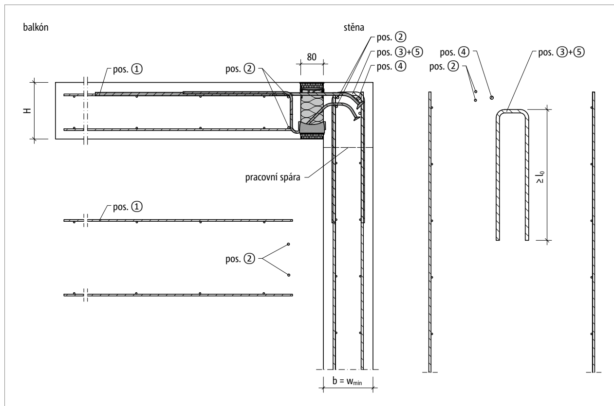
Obr. 98: Schöck Isokorb® T typ KL-O: Napojovací stavební výztuž pro desku kotvenou do hlavy stěny s minimálním rozměrem ( w_{skut} = w_{min} )
