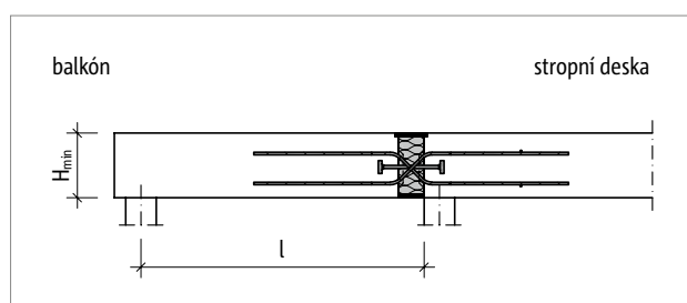
Obr. 135: Schöck Isokorb® T typ QP-VV: Statický systém
