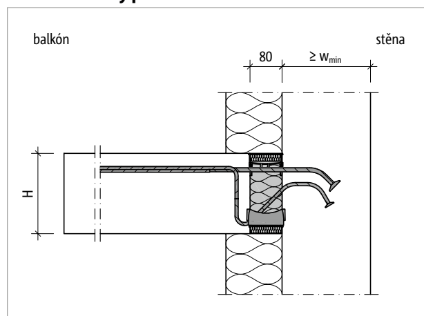
Obr. 75: Schöck Isokorb® T typ KL-O: Spojení stěn směrem dolů s vnější izolací
