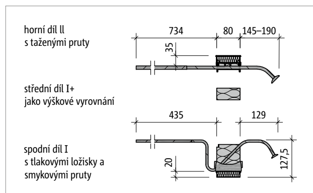
Obr. 104: Schöck Isokorb® T typ KL-O-F-M1-V1-CV1 až KL-O-F-M3-V1-CV1
