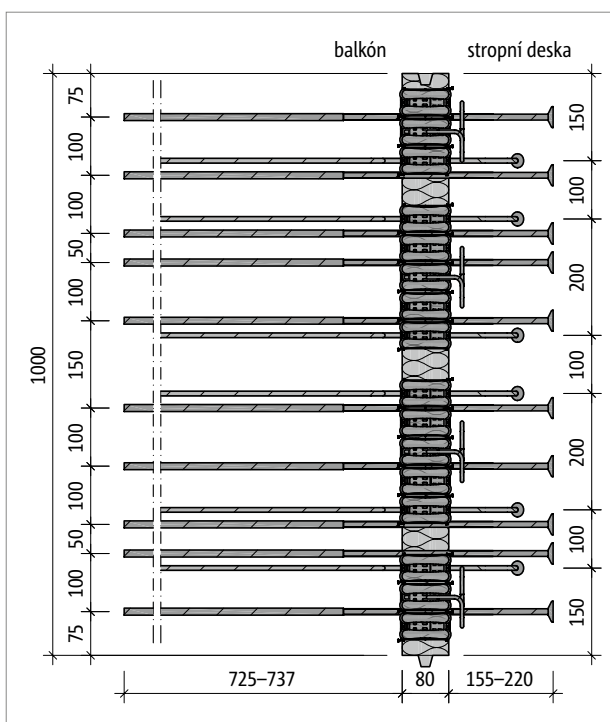
Obr. 87: Schöck Isokorb® T typ KL-U-M4: Půdorys prvku
