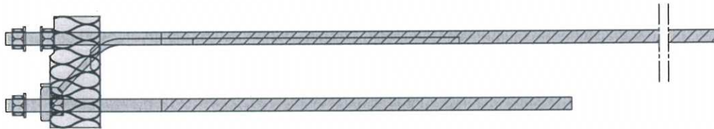
Abb.3 Schöck Isokorb Typ KS20 V10 und KS20 V12
