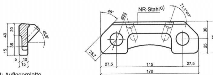
Abb. 21: Auflagerplatte
