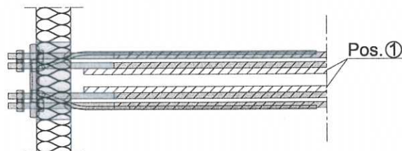
Abb. 47 Draufsicht: Schöck Isokorb Typ KS14 VV
