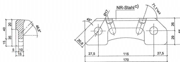
Abb. 15: Auflagerplatte
