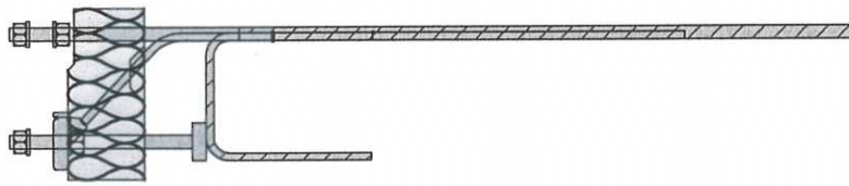
Abb.1 Schöck Isokorb Typ KS14 V8 und KS14 V10
