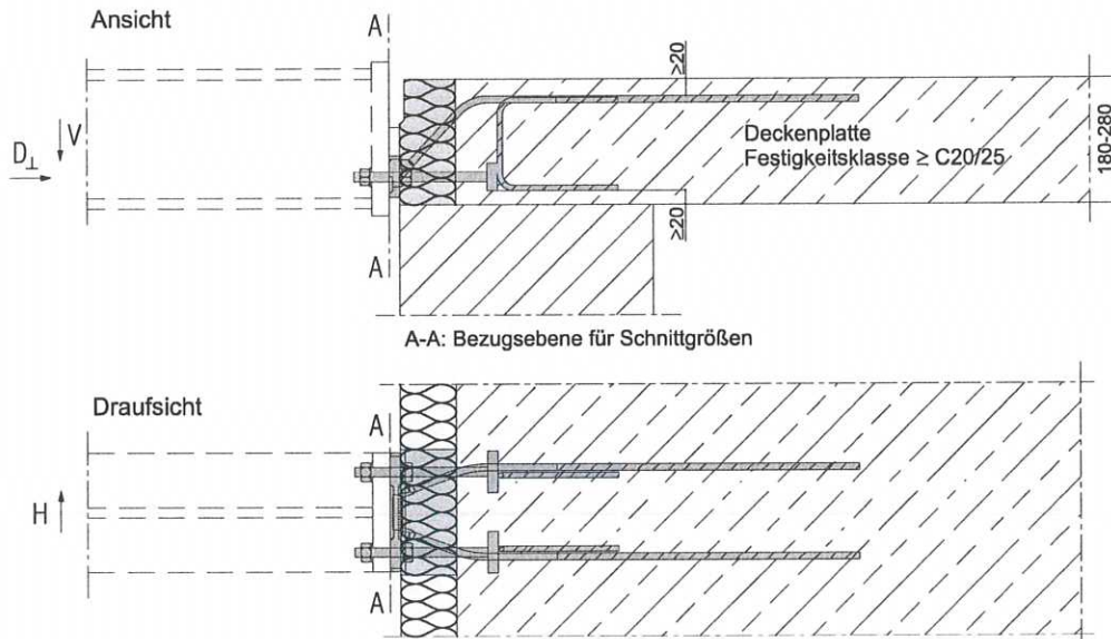
Abb. 33 und 34: Schöck Isokorb Typ QS10 und QS22, Schnittgrößendefinition
