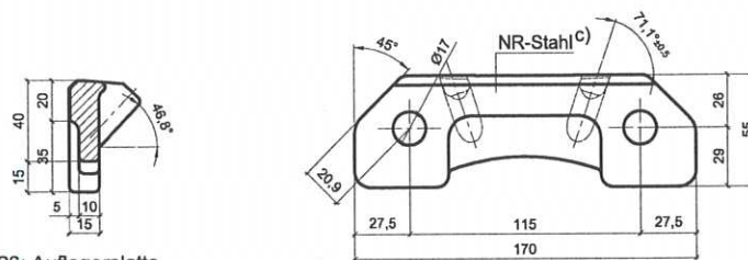
Abb. 26: Auflagerplatte
