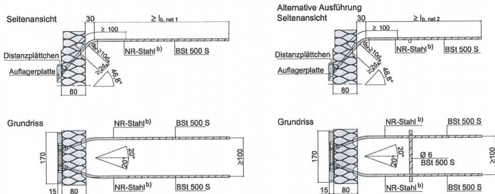
Abb. 9a bis 9d: Querkräftestäbe 2 Ø d s inkl. Auflagerplatte
