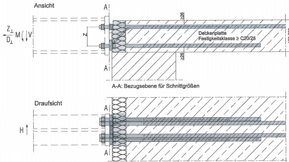
Abb. 31 und 32: Schöck Isokorb Typ KS20, Schnittgrößendefinition
