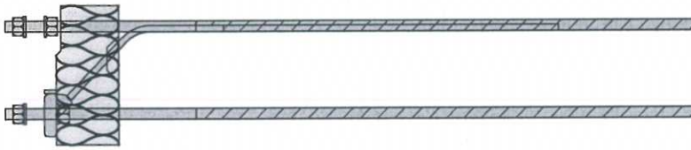
Abb.2 Schöck Isokorb Typ KS14 VV
