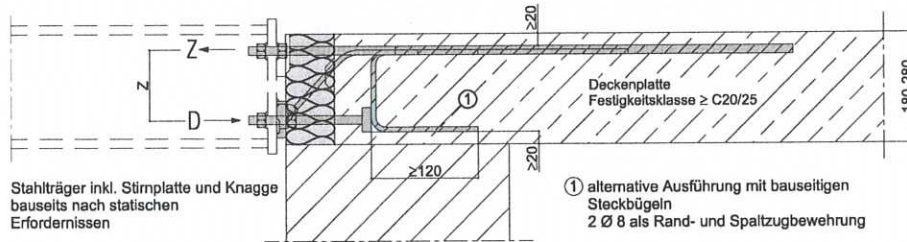
Abb. 5: Schöck Isokorb Typ KS14 V8 und KS14 V10
