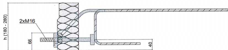
Abb. 42 Seitenansicht: Schöck Isokorb Typ QS10 und QS12
