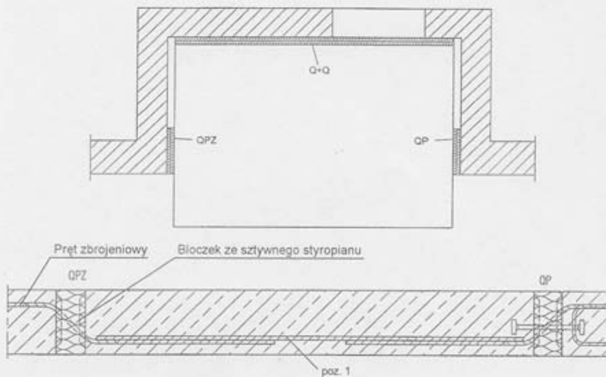
Rysunek 23. Połączenia wykonane z zastosowaniem łączników w wersjach QPZ, Q oraz QP
