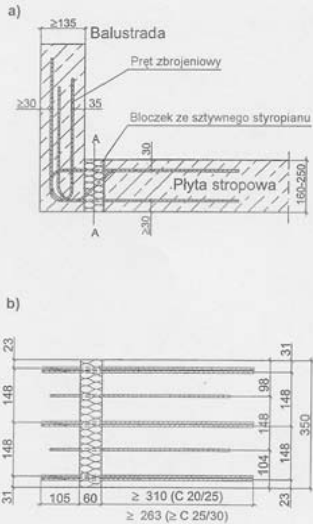
Rysunek 33. Połączenie wykonane z zastosowaniem łącznika w wersji F (a), łącznik w wersji F (b)
