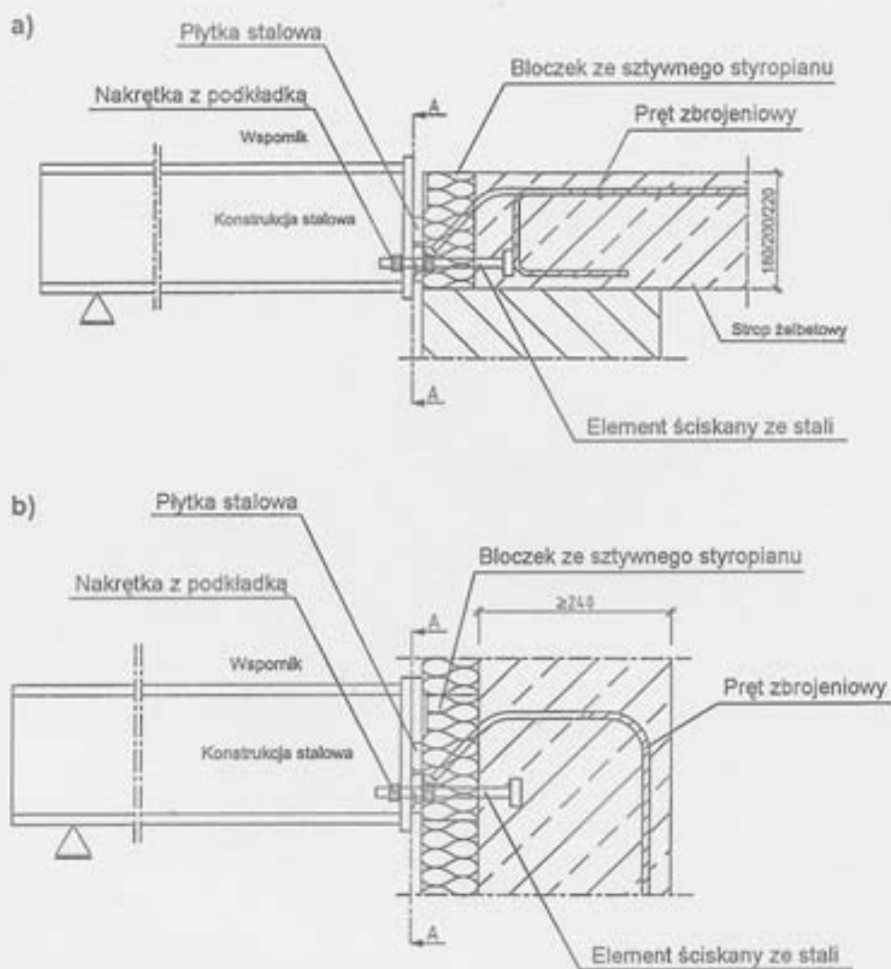
Rysunek 46. Połączenie wykonane z zastosowaniem łączników w wersji QS a) z zastosowaniem łącznika QS, b) z zastosowaniem łącznika QS-WU
