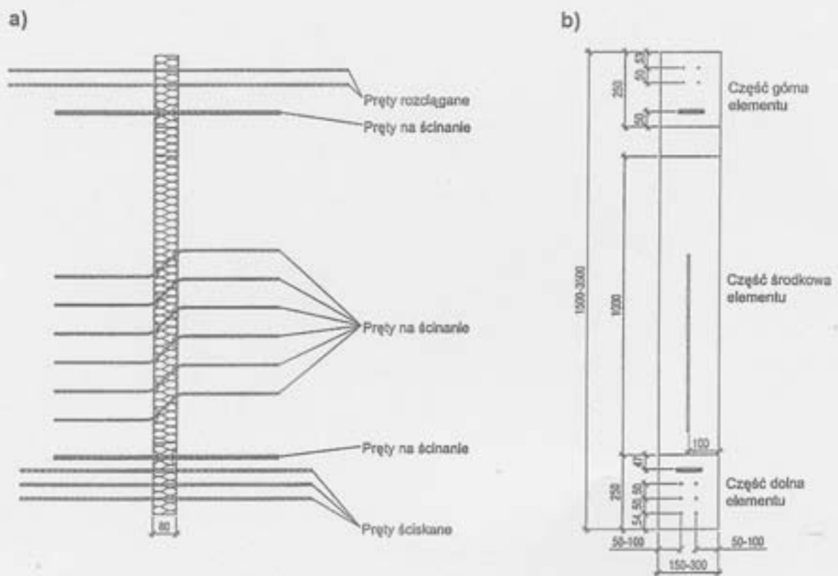
Rysunek 40. Rzut poziomy i pionowy łącznika w wersji W a) widok z boku, b) widok z przodu
