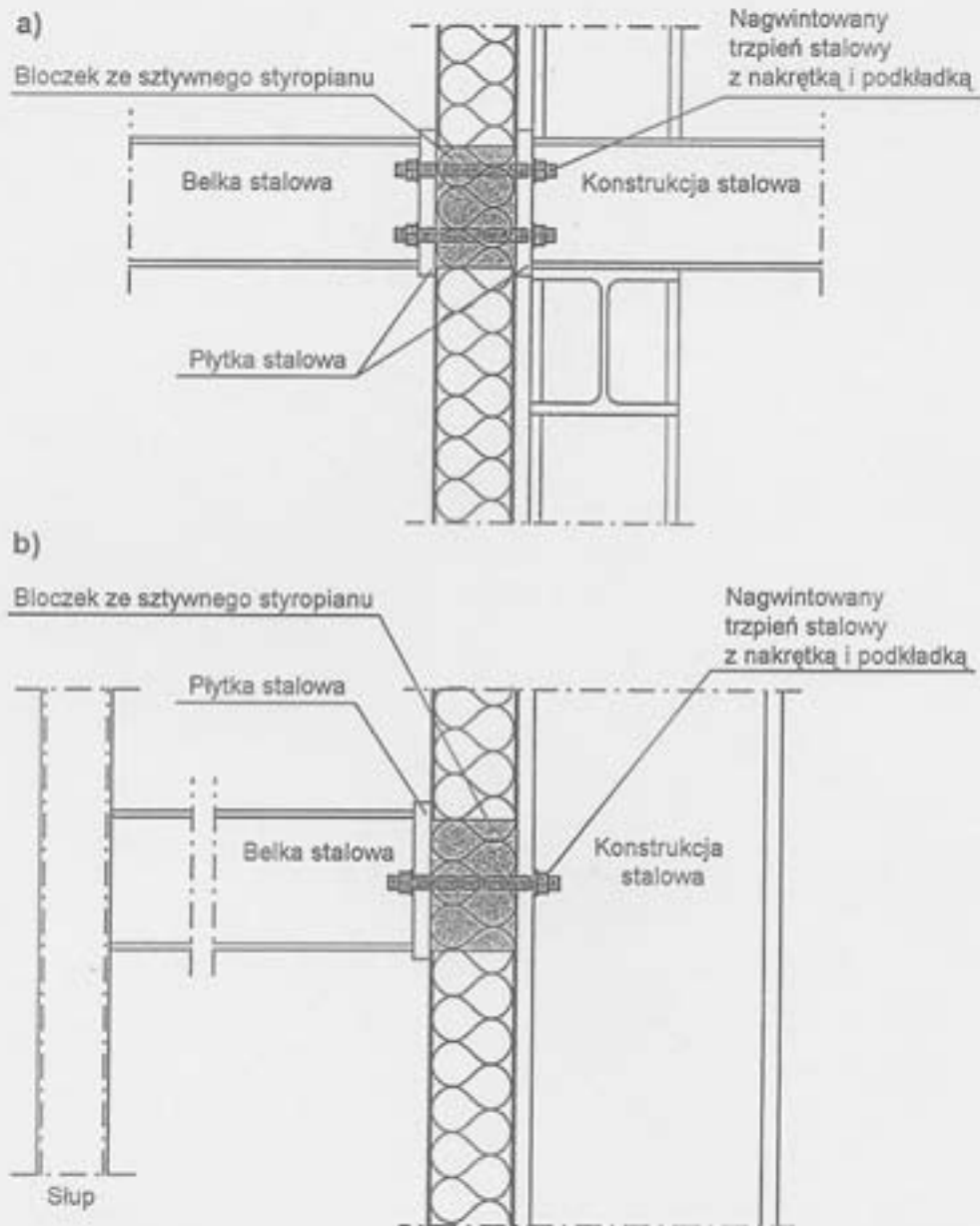
Rysunek 49. Połączenie wykonane z zastosowaniem łączników w wersji KST a) z zastosowaniem łącznika KST, b) z zastosowaniem łącznika KST-QST lub KST-ZQST
