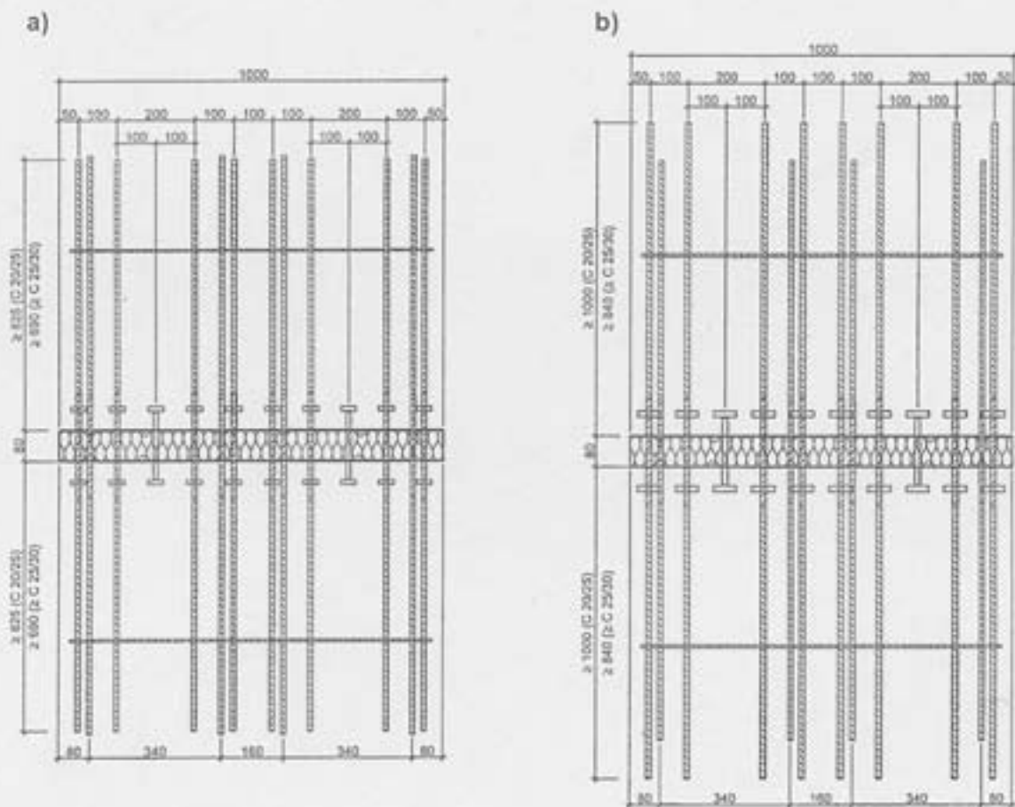
Rysunek 5. Łączniki w wersji K. Część III a) łącznik K 120, b) łącznik K 140
