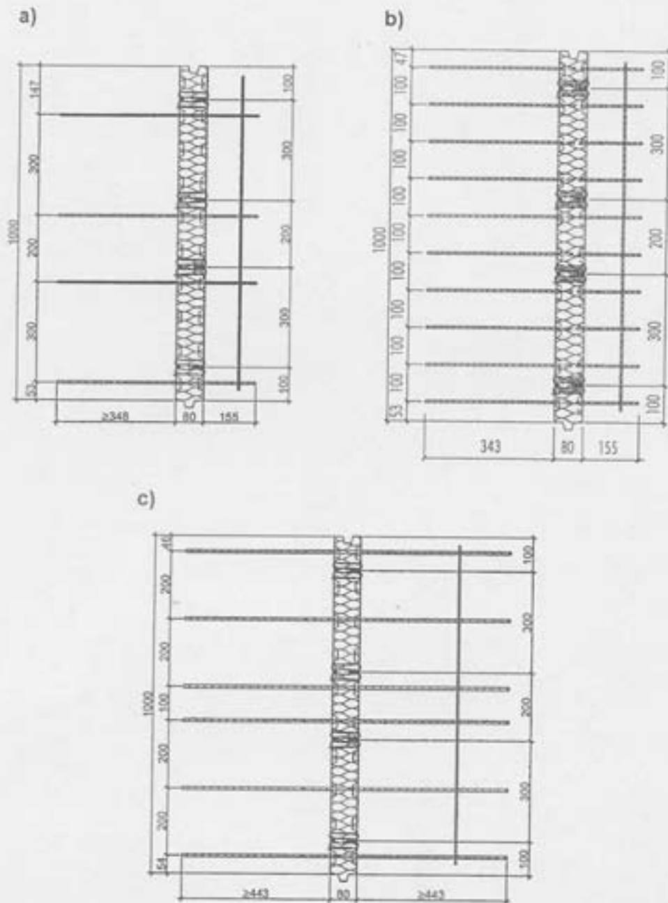
Rysunek 20. Łącznik w wersji Q
