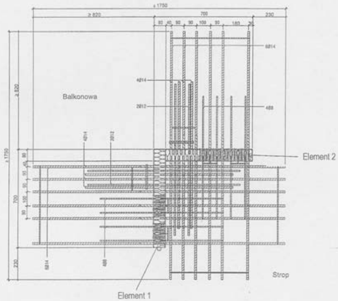
Rysunek 14. Łącznik K 50-Eck
