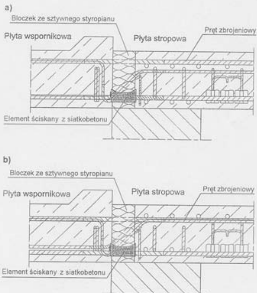
Rysunek 12. Połączenia wykonane z zastosowaniem łączników w wersji K-Eck
