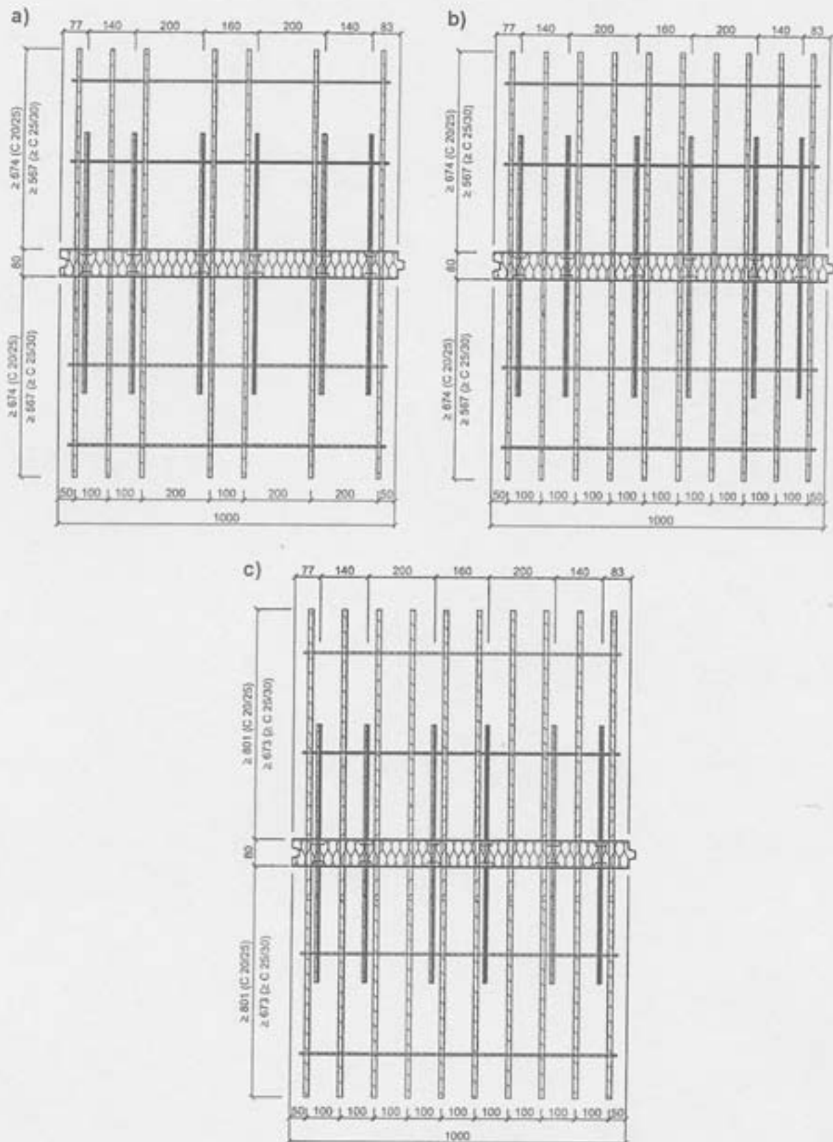
Rysunek 17. Łączniki w wersji D a) łącznik D 30, b) łącznik D 50, c) łącznik D 70
