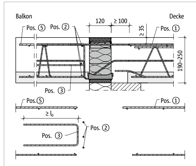
Abb. 69: Schöck Isokorb® XT Typ K-F: Bauseitige Bewehrung bei Balkonplattendicke h = 190\text{--}250\text{ mm} ; Variante mit Steckbügel
