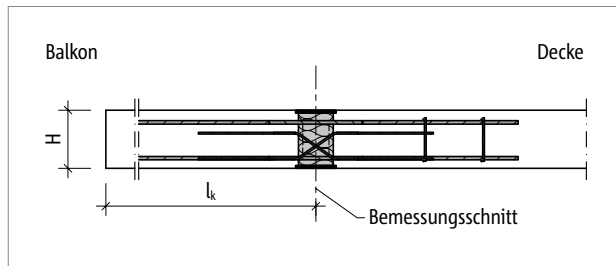
Abb. 253: Schöck Isokorb® XT Typ D: Statisches System
