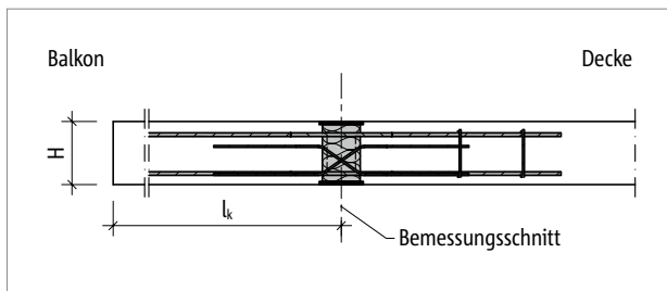
Abb. 251: Schöck Isokorb® XT Typ D: Statisches System
