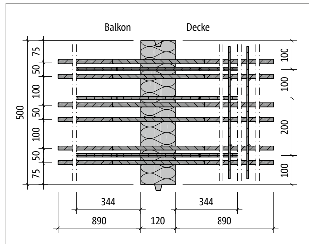
Abb. 259: Schöck Isokorb® XT Typ D-MM6-VV1: Grundriss
