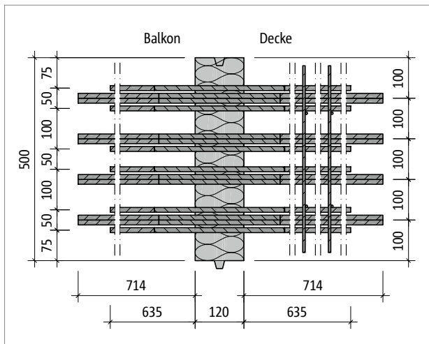
Abb. 258: Schöck Isokorb® XT Typ D-MM5-VV5: Grundriss
