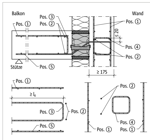
Abb. 156: Schöck Isokorb® XT Typ Q-V1 bis V4: Bauseitige Bewehrung in Wand
