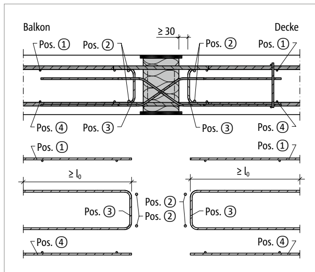
Abb. 260: Schöck Isokorb® XT Typ D: Bauseitige Bewehrung
