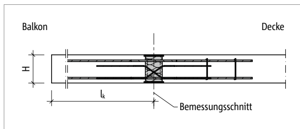
Abb. 252: Schöck Isokorb® XT Typ D: Statisches System
