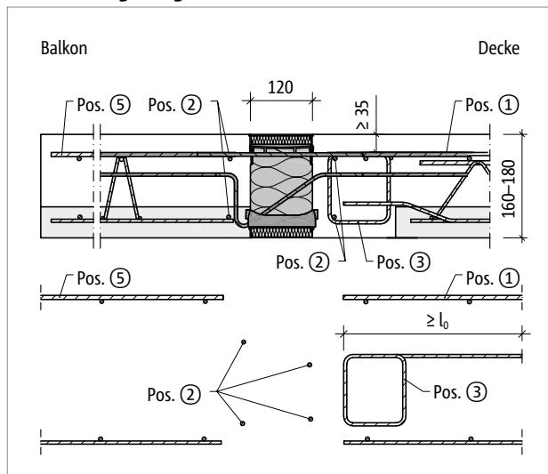
Abb. 72: Schöck Isokorb® XT Typ K-F: Bauseitige Bewehrung bei Balkonplattendicke h = 160-180 \text{ mm}
