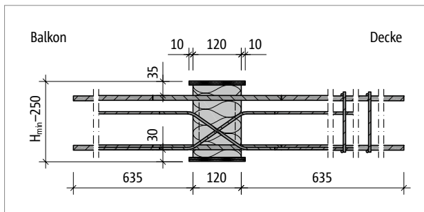
Abb. 254: Schöck Isokorb® XT Typ D-MM1-VV1 bei CV35: Produktschnitt
