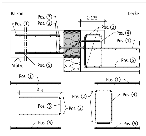
Abb. 206: Schöck Isokorb® XT Typ Q-P-V1 bis V4: Bauseitige Bewehrung für Balkon mit Höhenversatz nach oben
