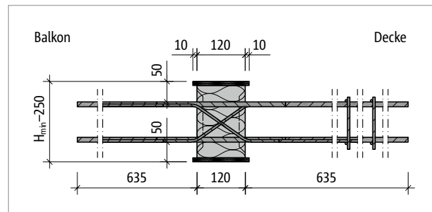
Abb. 255: Schöck Isokorb® XT Typ D-MM1-VV1 bei CV50: Produktschnitt
