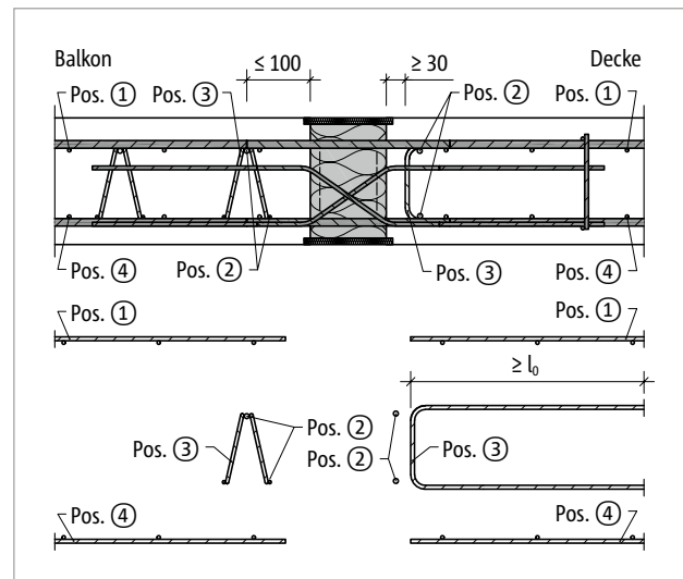
Abb. 261: Schöck Isokorb® XT Typ D: Bauseitige Bewehrung mit Gitterträger
