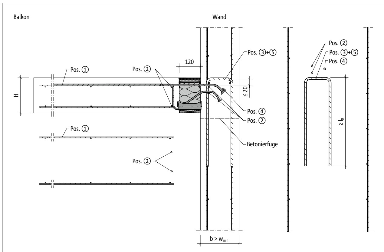
Abb. 119: Schöck Isokorb® XT Typ K-O: Bauseitige Bewehrung für Wandanschluss mit größerer Bauteilabmessung ( w_{\text{vorh}} > w_{\text{min}} )
