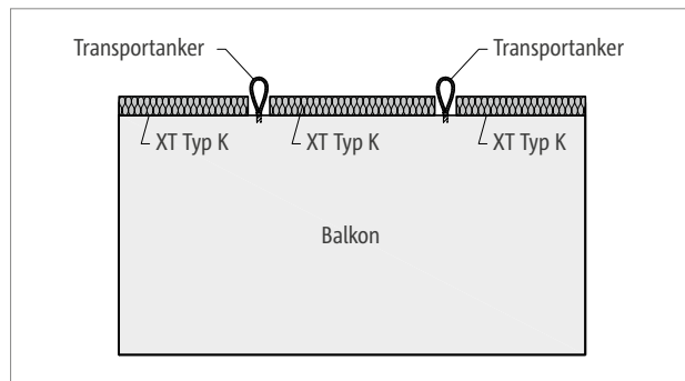
Abb. 238: Schöck Isokorb® XT Typ K: Vollfertigteilbalkon mit Transportanker; Dämmzwischenstück XT Typ Z kann bauseitig eingelegt werden
