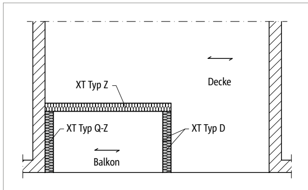
Abb. 247: Schöck Isokorb® XT Typ D, Q-Z: Decke einachsrig gespannt
