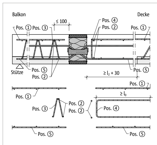
Abb. 164: Schöck Isokorb® XT Typ Q-VV5 bis VV10: Bauseitige Bewehrung mit Gitterträger
