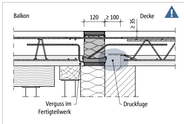
Abb. 75: Schöck Isokorb® XT Typ K-F: Druckfuge deckenseitig in Verbindung mit Halbfertigteilplatten; direkte Lagerung
