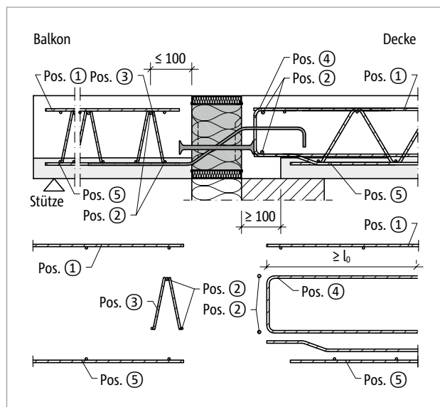
Abb. 196: Schöck Isokorb® XT Typ Q-P-V1 bis V4: Bauseitige Bewehrung mit Gitterträger
