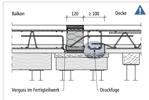
Abb. 76: Schöck Isokorb® XT Typ K-F: Druckfuge deckenseitig in Verbindung mit Halbfertigteilplatten; indirekte Lagerung
