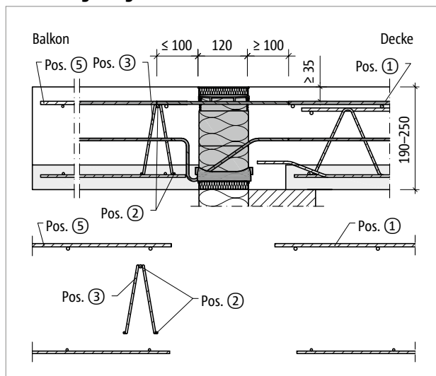
Abb. 70: Schöck Isokorb® XT Typ K-F: Bauseitige Bewehrung bei Balkonplattendicke h = 190\text{--}250\text{ mm} (Pos.2: 2\phi 8 ); Variante mit Gitterträger
