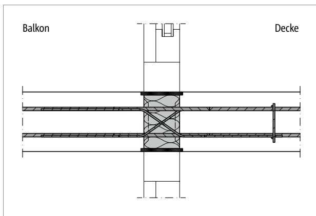
Abb. 249: Schöck Isokorb® XT Typ D: Einbauschritt; einachsrig gespannte Decke
