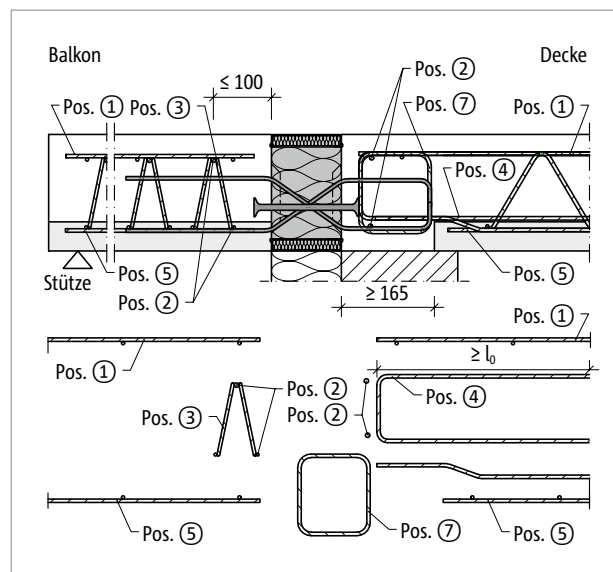
Abb. 197: Schöck Isokorb® XT Typ Q-P-VV1 bis VV4: Bauseitige Bewehrung mit Gitterträger
