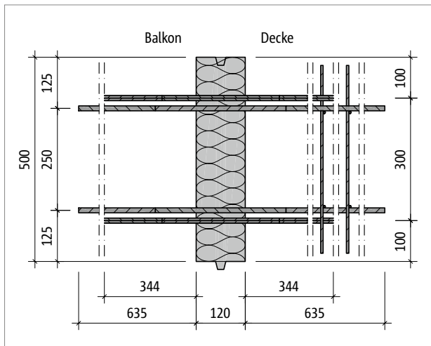
Abb. 256: Schöck Isokorb® XT Typ D-MM1-VV1: Grundriss
