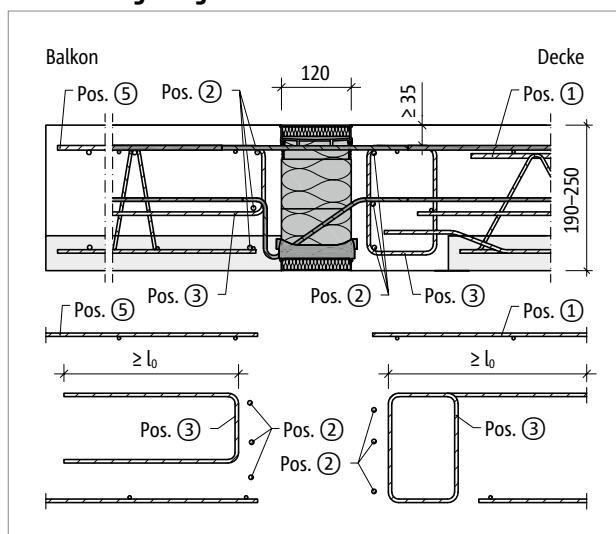
Abb. 73: Schöck Isokorb® XT Typ K-F: Bauseitige Bewehrung bei Balkonplattendicke h = 190-250 \text{ mm} ; Variante mit Steckbügel
