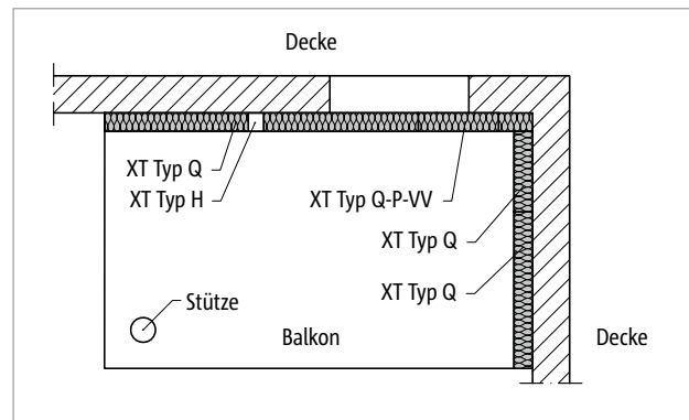
Abb. 177: Schöck Isokorb® XT Typ Q, Q-P-VV: Balkon zweiseitig gelagert mit Stütze und abhebenden Querkraften
