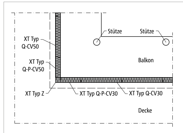
Abb. 213: Schöck Isokorb® XT Typ Q-P, Q: Innenecke; Grundriss bei gestütztem Balkon (ohne Einrücken erforderlich)
