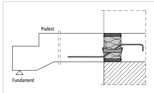
Abb. 140: Schöck Isokorb® XT Typ Q-V1 bis V4: Anschluss Treppenpodest bei einschaligem, wärmedämmendem Mauerwerk
