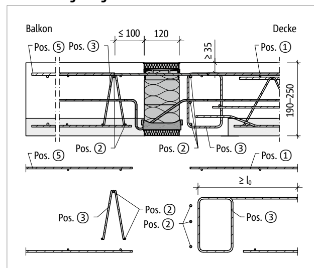
Abb. 74: Schöck Isokorb® XT Typ K-F: Bauseitige Bewehrung bei Balkonplattendicke h = 190-250 \text{ mm} (Pos.2: 5\phi 8 ); Variante mit Gitterträger
