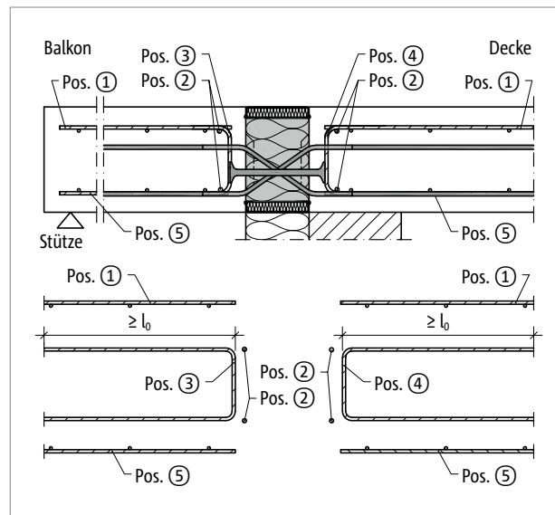
Abb. 195: Schöck Isokorb® XT Typ Q-P-VV5 bis VV16: Bauseitige Bewehrung
