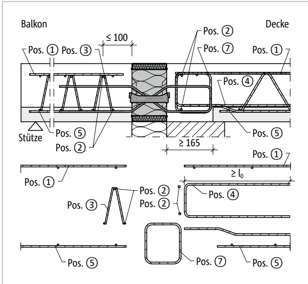
Abb. 154: Schöck Isokorb® XT Typ Q-VV1 bis VV4 Bauseitige Bewehrung mit Gitterträger
