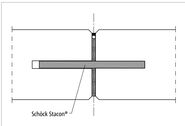
Abb. 17: Schöck Stacon®: Dehnfugenausbildung Ortbeton
