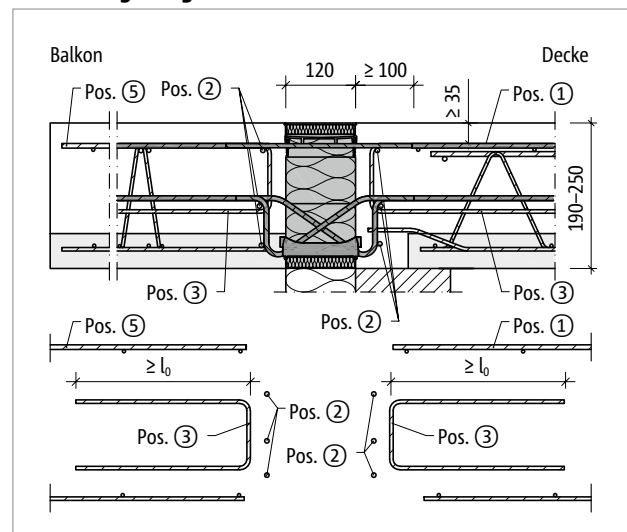
Abb. 71: Schöck Isokorb® XT Typ K-F-VV: Bauseitige Bewehrung bei Balkonplattendicke h = 190\text{--}250\text{ mm} ; Variante mit Steckbügel
