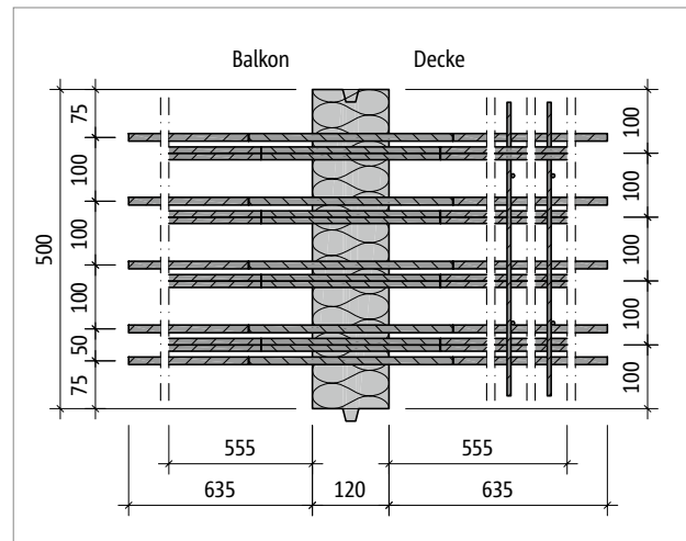
Abb. 257: Schöck Isokorb® XT Typ D-MM4-VV4: Grundriss
