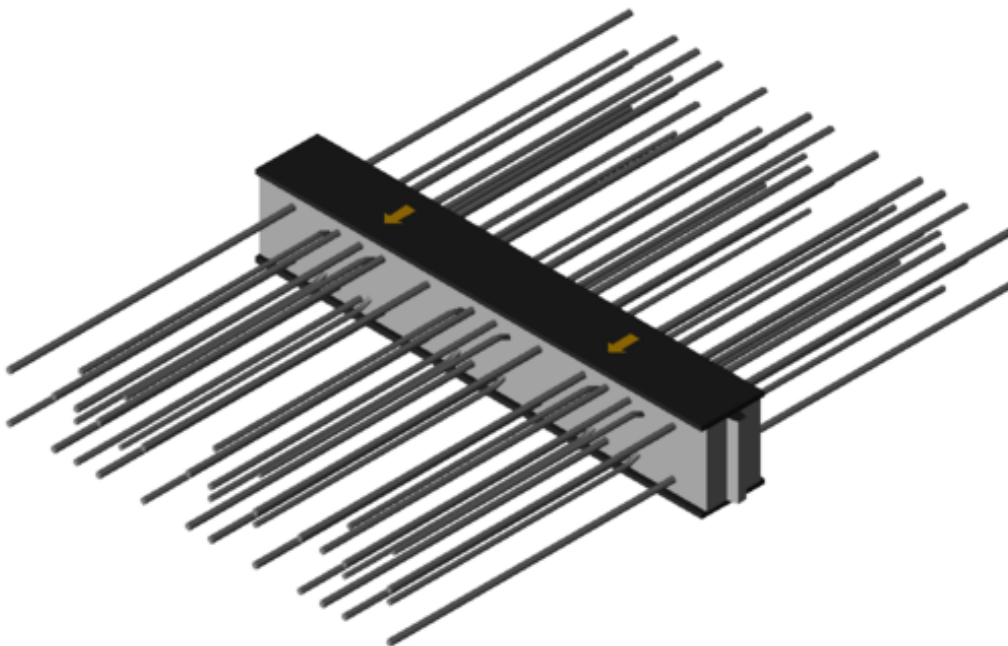
Abbildung 2: Schöck Isokorb® XT Typ D-MM5-VV3-REI120-CV35-X120-H180-L1000-5.0
