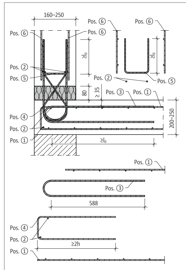
Fig. 240: Schöck Isokorb® T tipo A: Armadura in situ exterior
