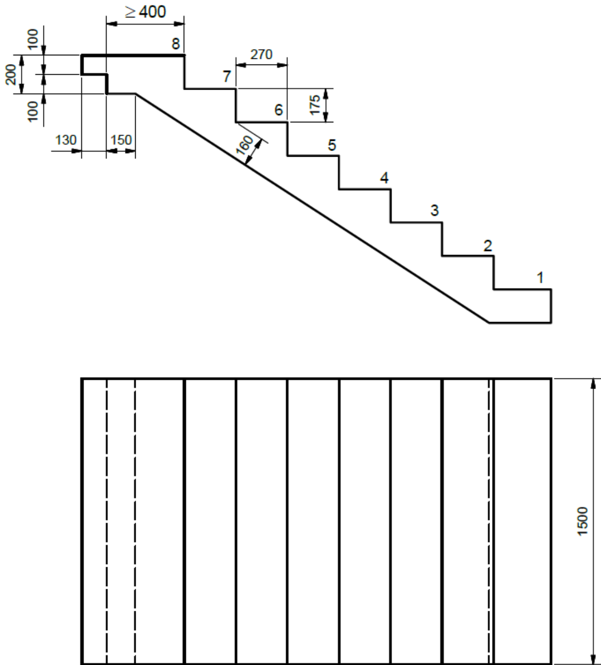
Abbildung 4: Draufsicht und Ansicht des Referenztreppenlaufes (alle Maße in mm)
