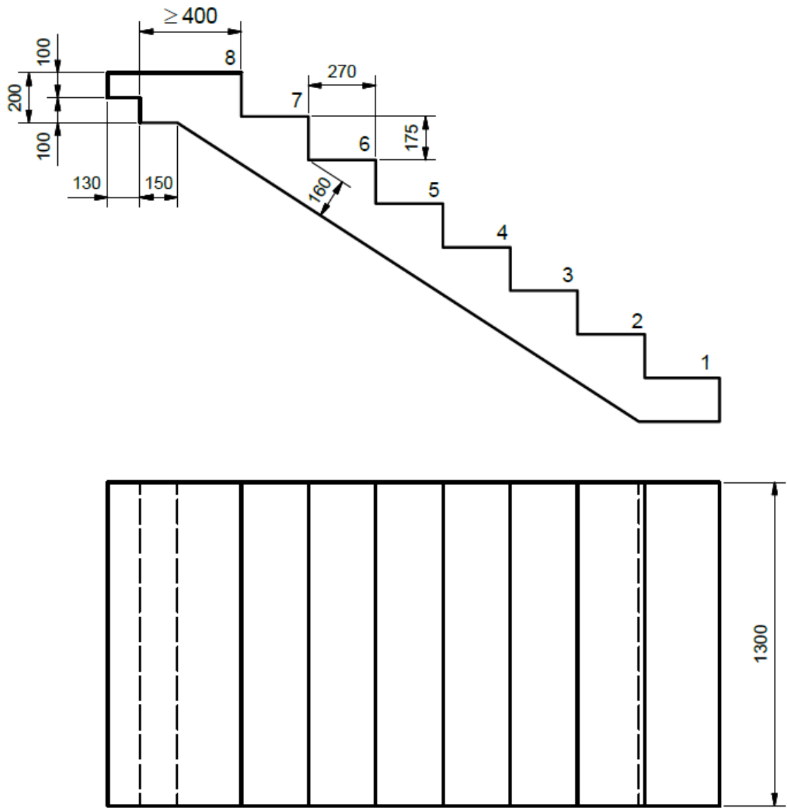
Abbildung 4: Draufsicht und Ansicht des Referenztreppenlaufes (alle Maße in mm)
