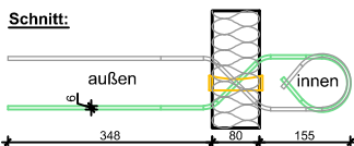
Schöck Isokorb T_Q-V(V)1 bis T_Q-V(V)5
