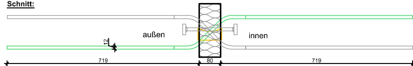
Schöck Isokorb T_Q-V(V)9 bis T_Q-V(V)11 und T_Q-P-V(V)6 + T_Q-P-V(V)7
