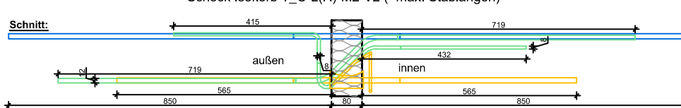
Schöck Isokorb T_C-L(R)-M2-V2 (=max. Stablängen)
