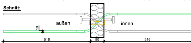
Schöck Isokorb T_Q-V(V)7 + T_Q-V(V)8 und T_Q-P-V(V)4 + T_Q-P-V(V)5
