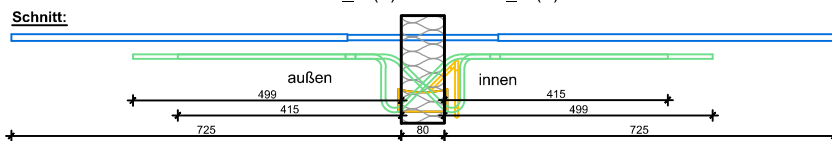
Schöck Isokorb T_K(F)-M6-VV bis T_K(F)-M11-VV
