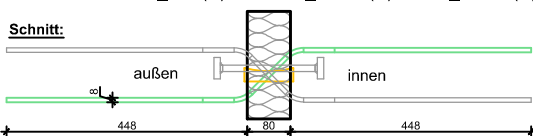
Schöck Isokorb T_Q-V(V)6 und T_Q-P-V(V)1 bis T_Q-P-V(V)3
