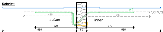
Schöck Isokorb T_K(F)-M1-V1/V2 bis T_K(F)-M6-V1/V3
