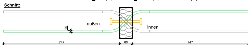
Schöck Isokorb T_Q-V(V)12 + T_Q-P-V(V)8 bis T_Q-P-V(V)10
