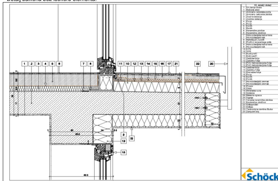
Detalj balkona bez Isokorb elementa.
