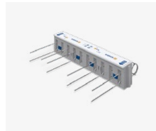
Schöck Isokorb® XT Typ QL-VV positive und negative Querkraft
