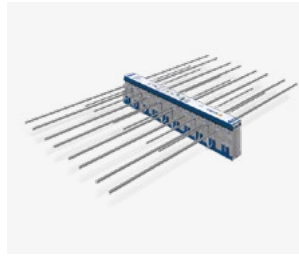
Schöck Isokorb® T Typ KL
