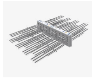
Schöck Isokorb® T Typ DL
