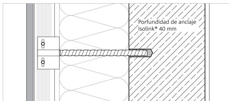
Isolink® con punto fijo
