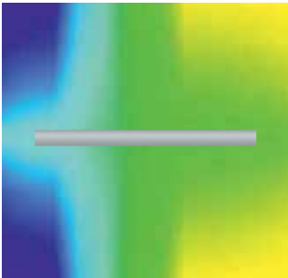
Isotermas con aluminio: 160-200 W/(m · K)
