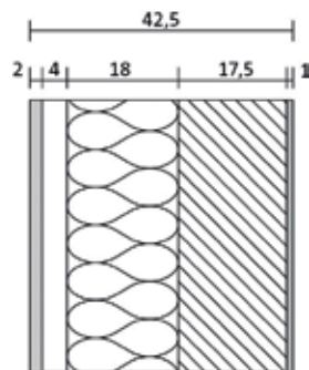
Estructura de pared con 3 soportes de pared de acero inoxidable y lana mineral de 18 cm WLG 035
