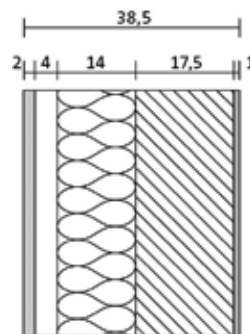
Estructura de pared con 3 soportes de pared Isolink® y lana mineral de 14 cm WLG 035
