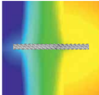
Isotermas con acero inoxidable: 13-15 W/(m · K)
