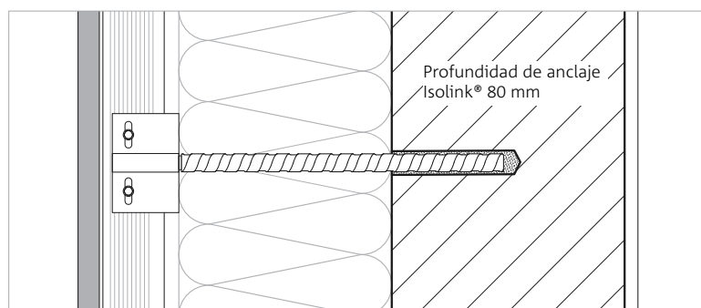
Isolink® con punto de deslizamiento
