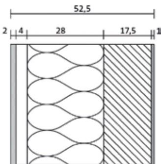
Estructura de pared con 3 soportes de pared de aluminio y lana mineral de 28 cm WLG 035
