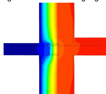
Isothermenbild des XT Typ K-M6V2
